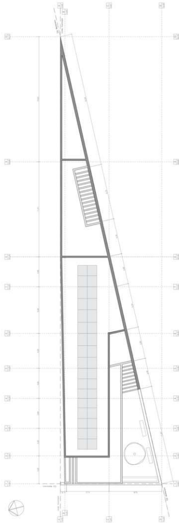
PLANTA DE TECHOS ESC 1:100
