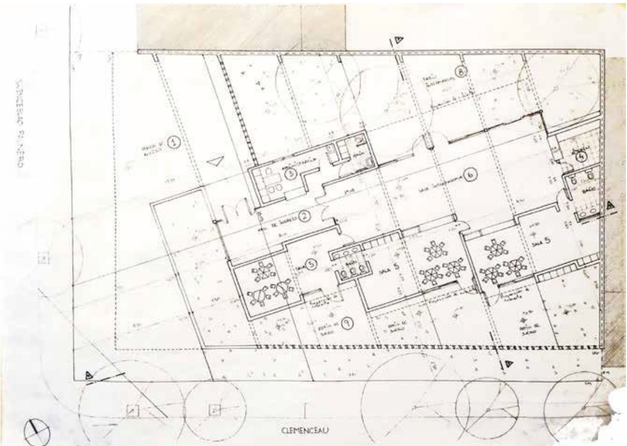
Planta y Vistas. escala original 1:100
