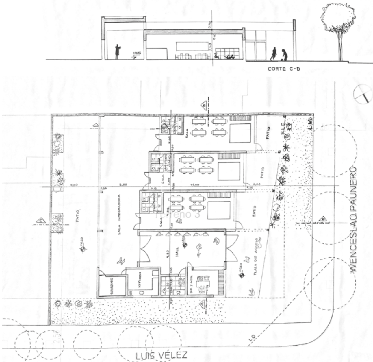
Cortes y Vistas. escala original 1:100
