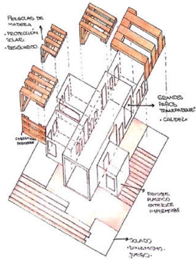
DESPIECE TECNOLÓGICO
