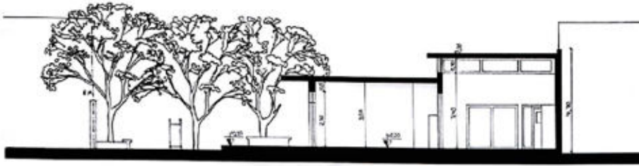
CORTE TRANSVERSAL A-B ESC 1:100
