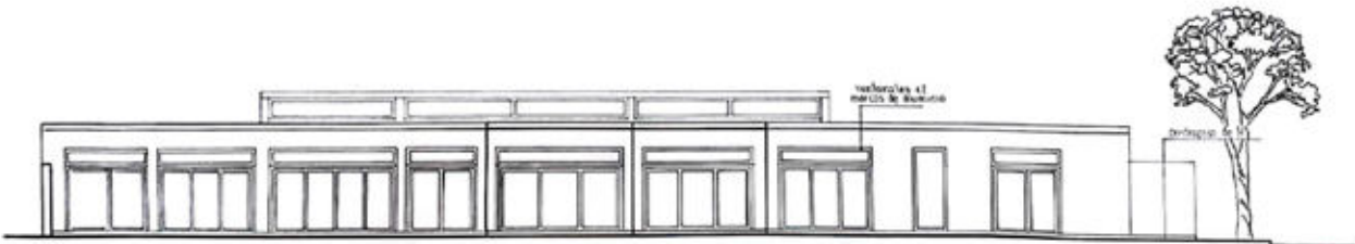
FACHADA LATERAL ESC 1:100
