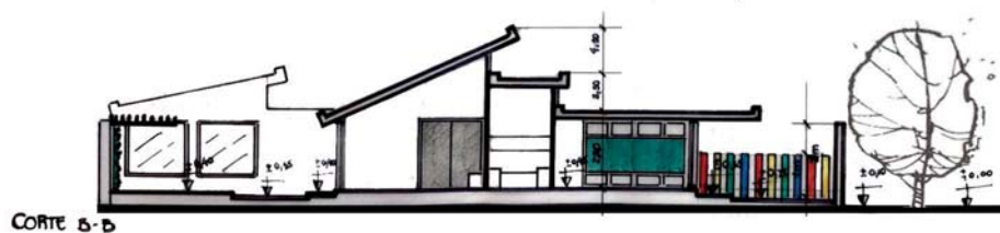
PLANTA, CORTE Y VISTA DE LA PROPUESTA
