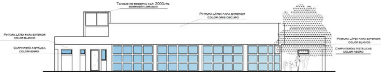
VISTA POSTERIOR Esc: 1/100
