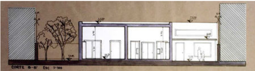
CORTE TRANSVERSAL
