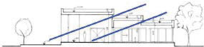
CORTE A-A Ingreso lumínico, orientación norte
