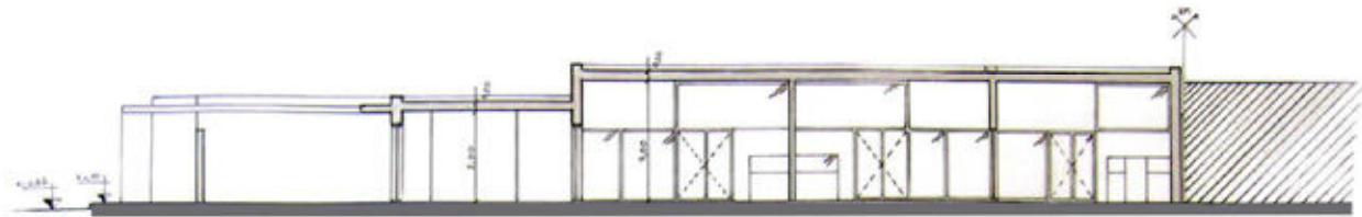
CORTE LONGITUDINAL B-B
