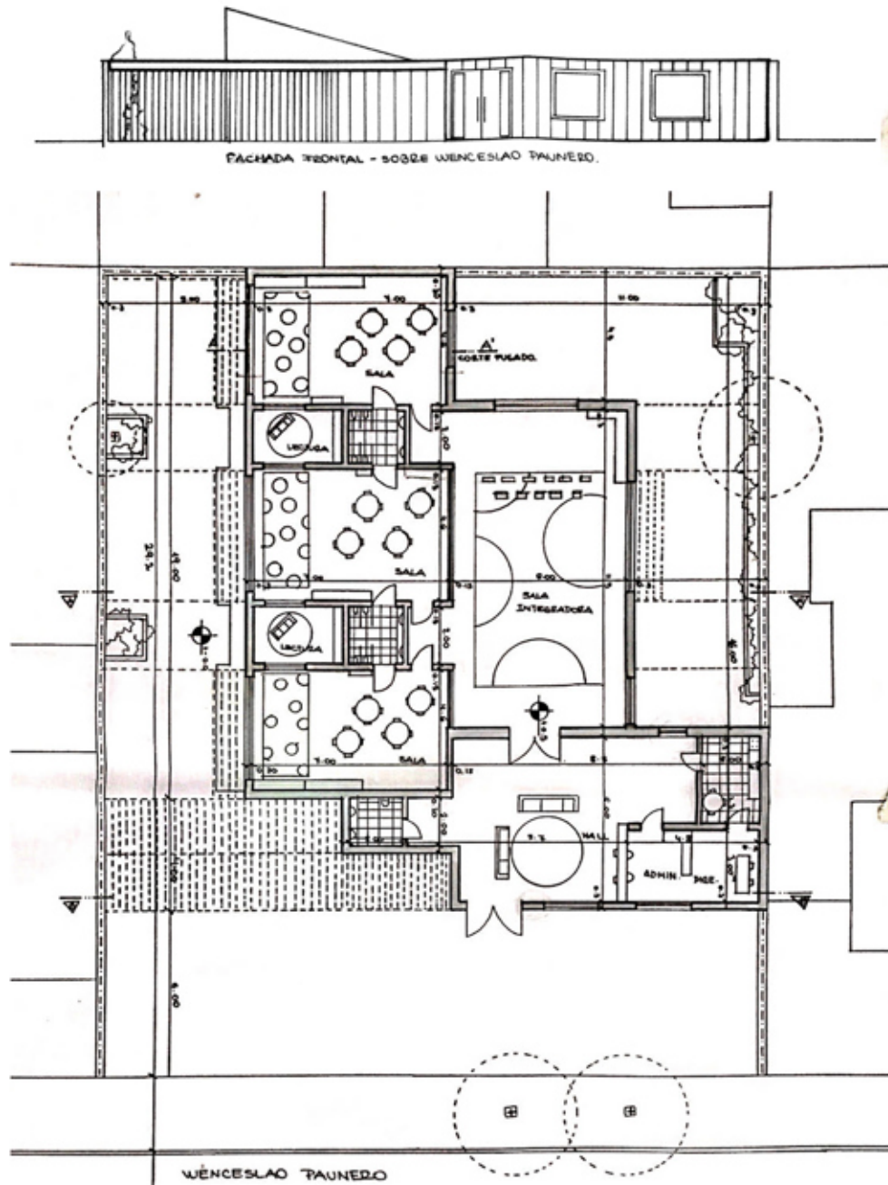
Planta y Vistas. escala original 1:100
