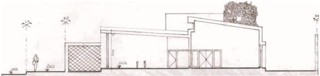
CORTE esc. 1:100
