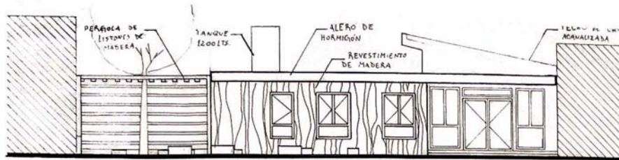
FACHADA OESTE ESC 1:100
