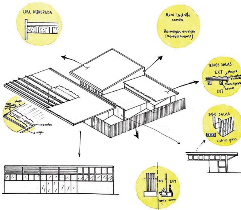
RESOLUCION TECNOLÓGICA DEL CONJUNTO ARQUITECTÓNICO.
