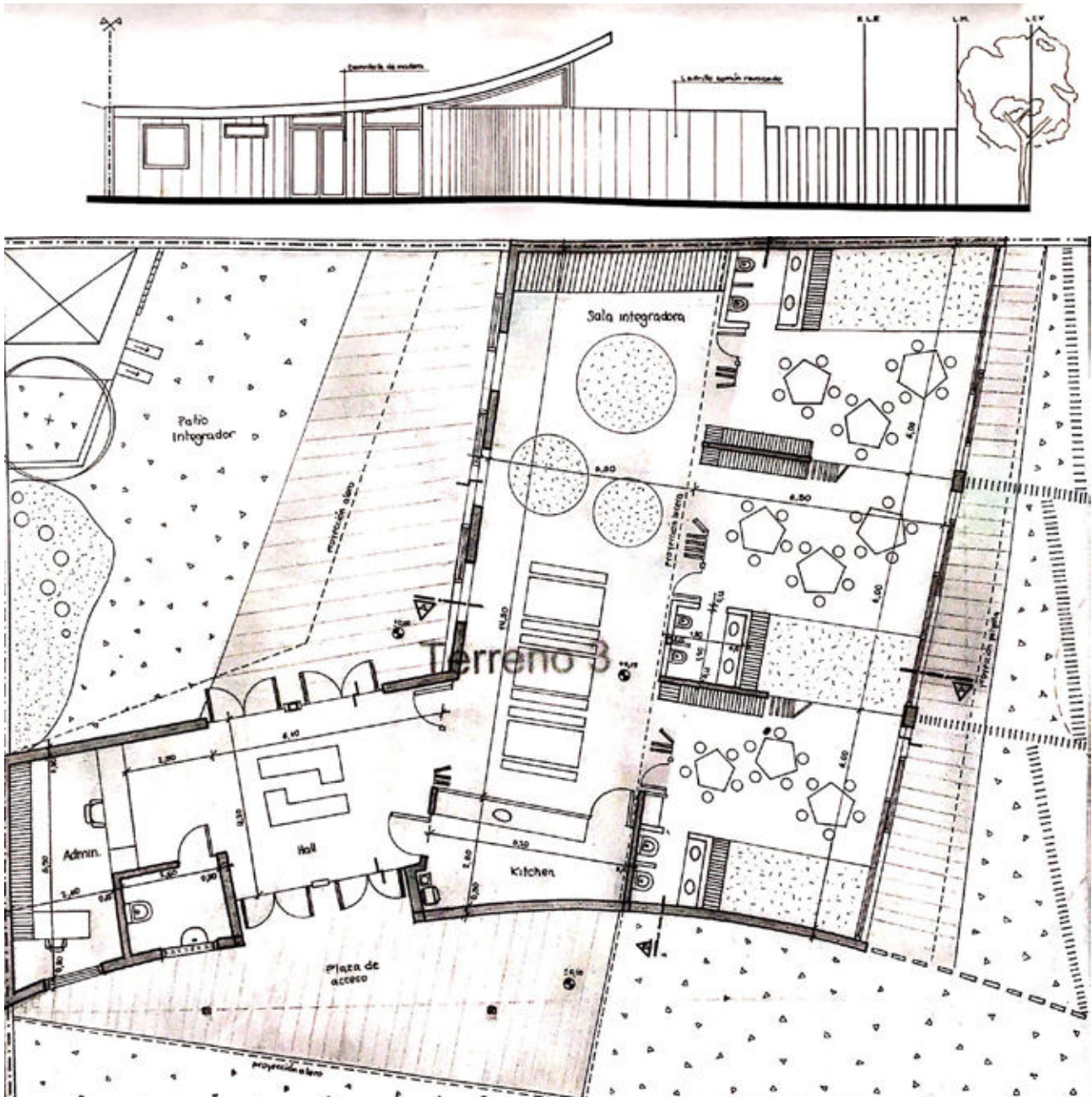
Planta, Vistas. escala original 1:100
