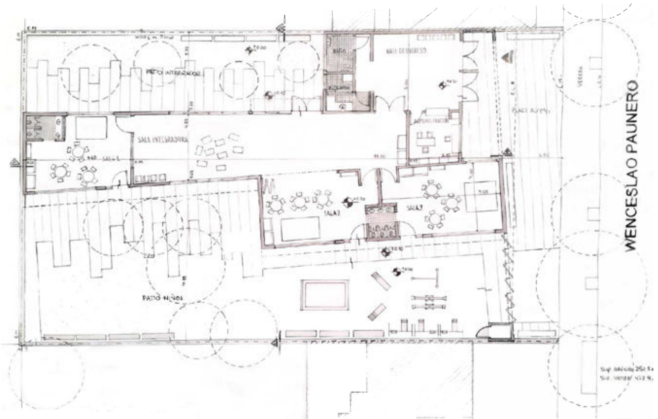
PLANTA JARDÍN MATERNAL Esc 1:100
