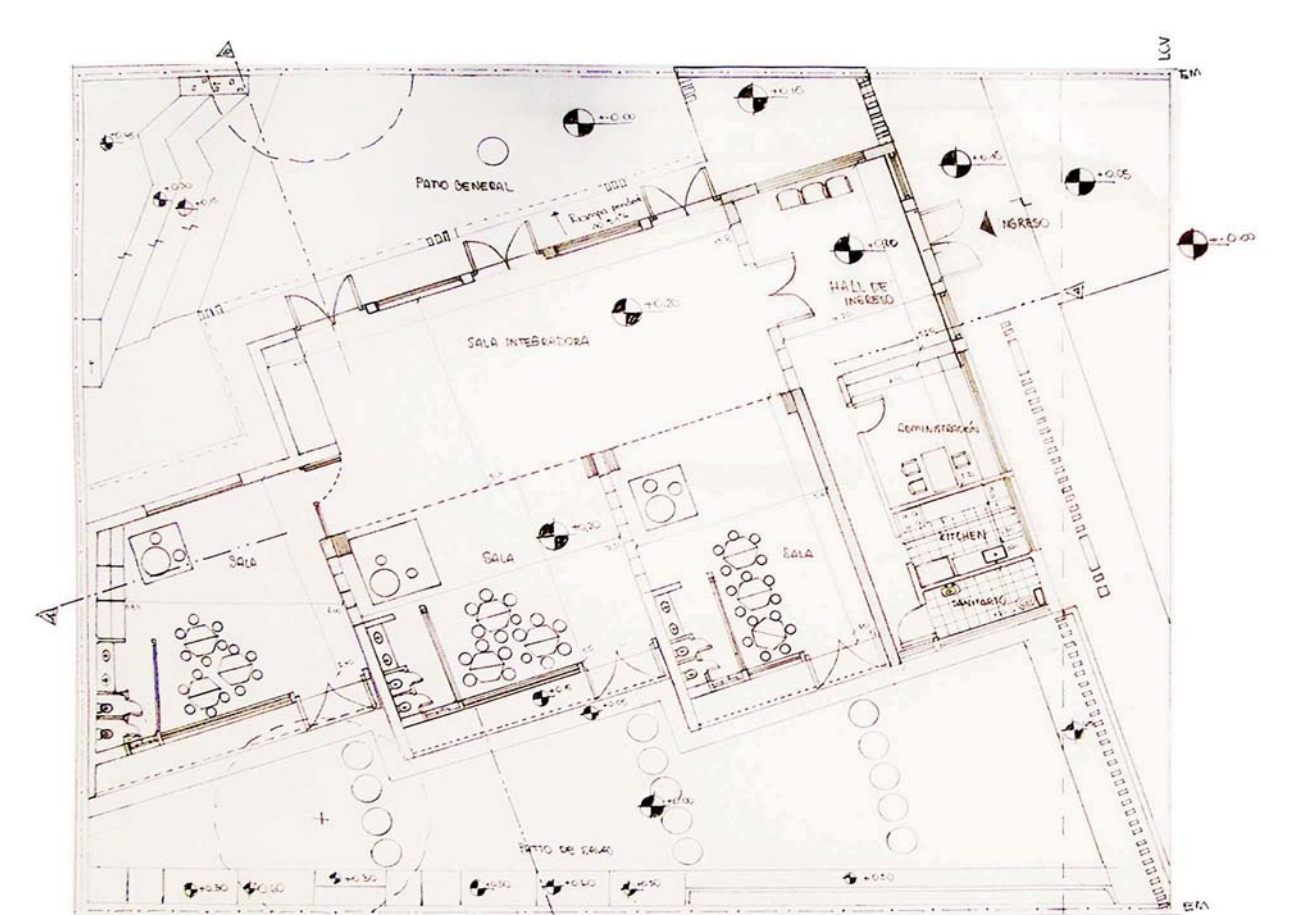
PLANTA BAJA Esc.1.100
