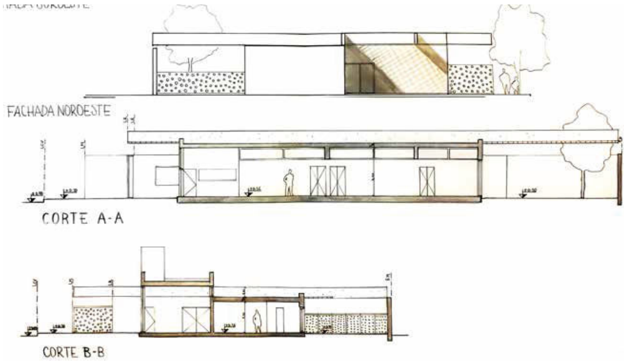
Cortes y Vistas. Escala original 1:100
