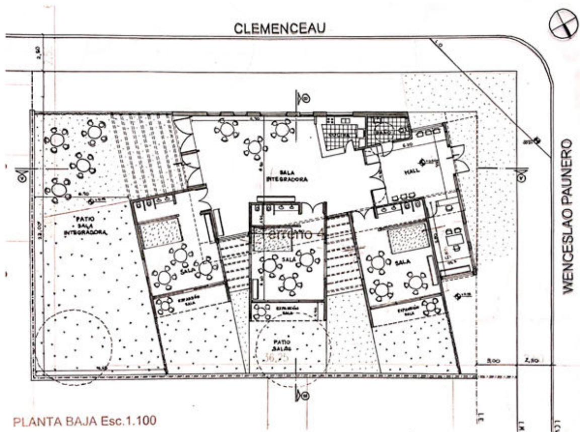
Planta y Vistas. escala original 1:100
