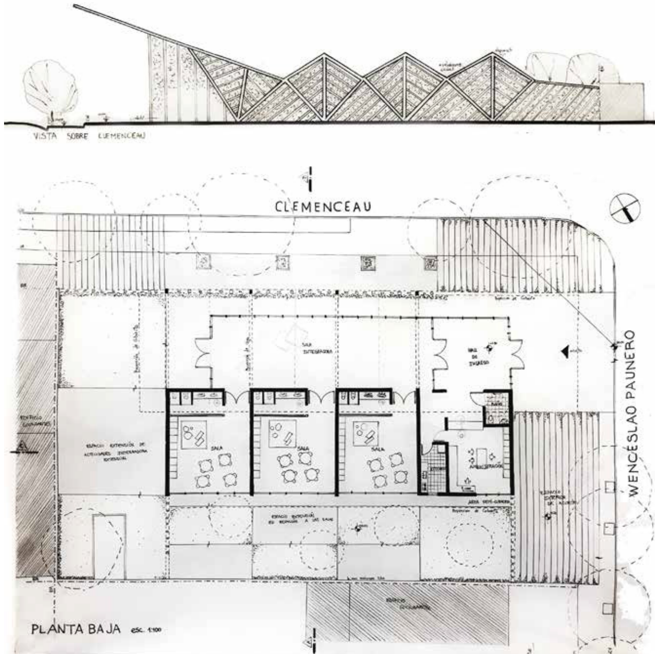
Planta y Vistas. escala original 1:100
