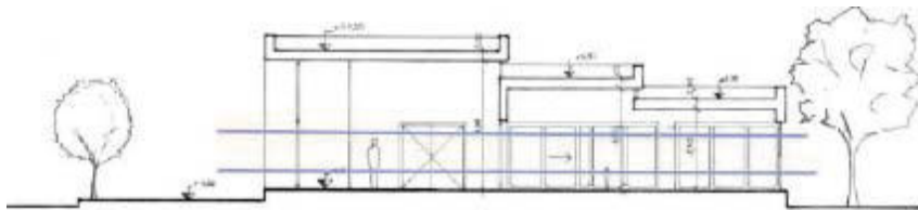
CORTE A-A Esquema de corte, ingreso lumínico y ventilación cruzada
