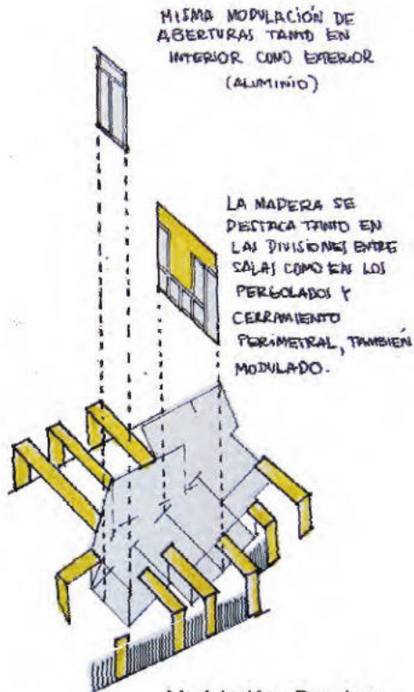
Modulación - Despiece
