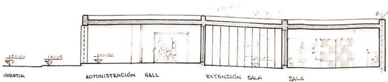
CORTE A-B
