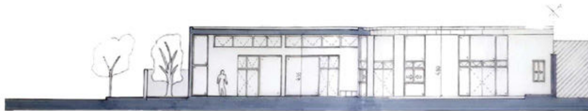
CORTE A-B Esc. 1:100
