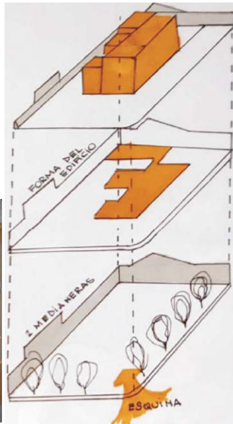
Forma emplazada. despiece volumétrico
