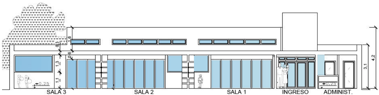
CORTE A-B Esc: 1/100
