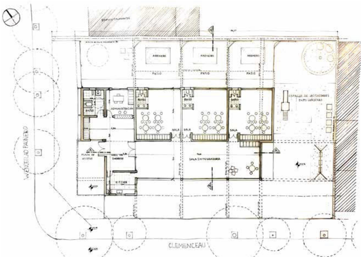
Planta, Vistas. Escala original 1:100
