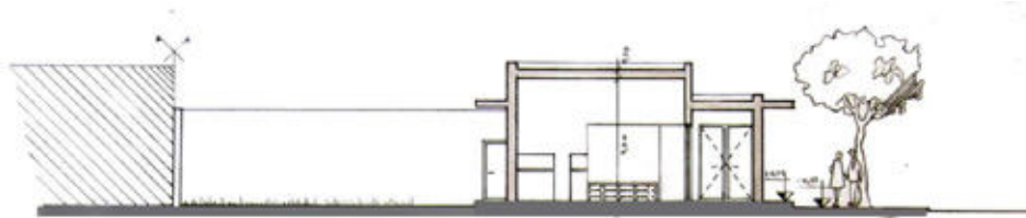
CORTE TRANSVERSAL A-A
