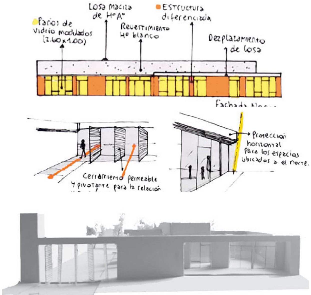
EXPLORACIONES DE MATERIALIDAD Y ENVOLVENTE
