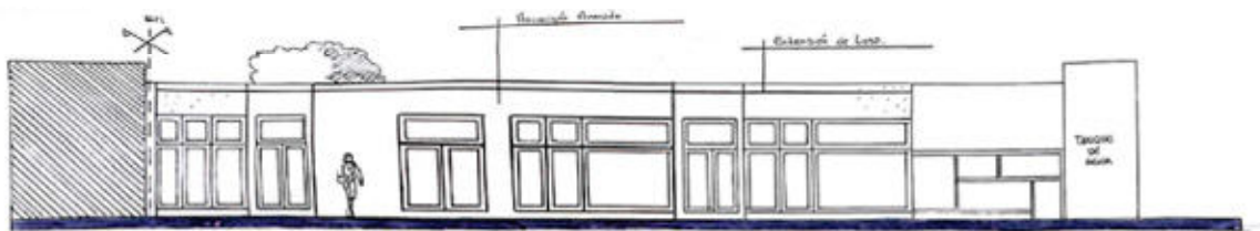
FACHADA NORTE LATERAL ESC. 1:100
