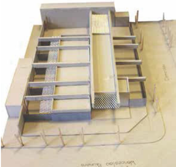
Maquetas Finales. Escala original 1:100 y 1:50
