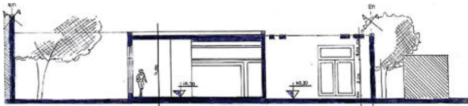
CORTE TRANSVERSAL C-D
