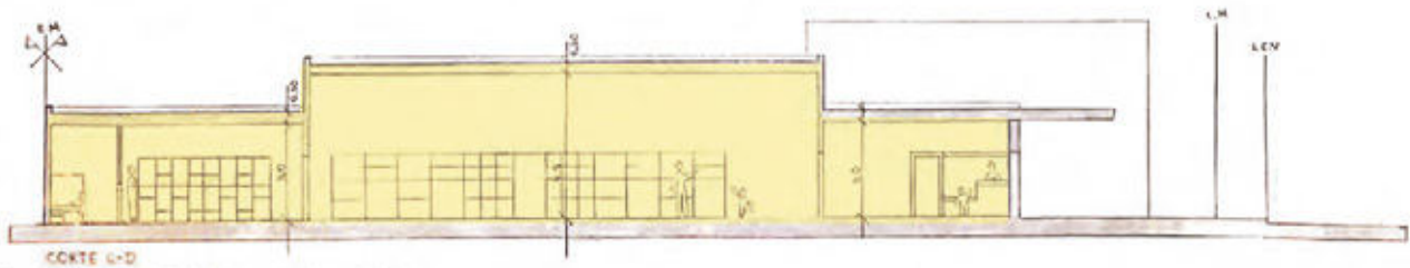
Corte Ingreso-Sala Integradora-Salas
