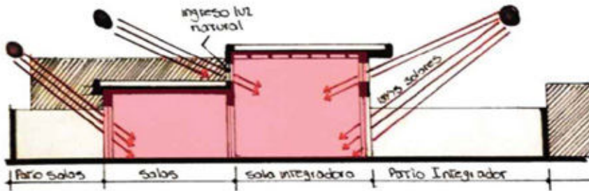
Cortes de Estudio: Asoleamiento
