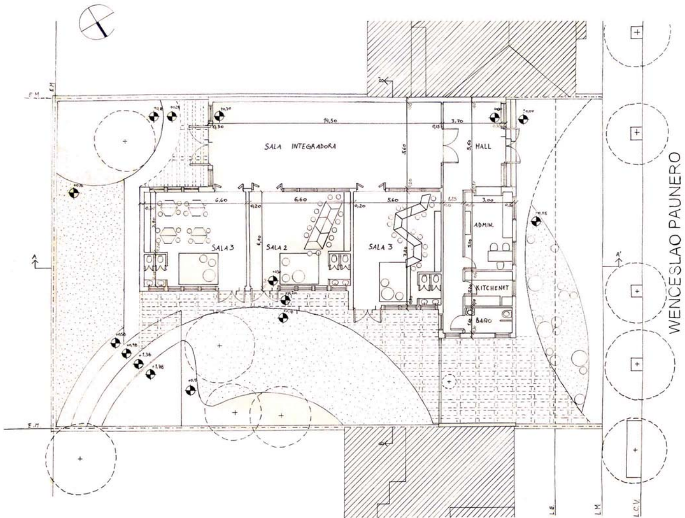
PLANTA BAJA Esc. 1.100
