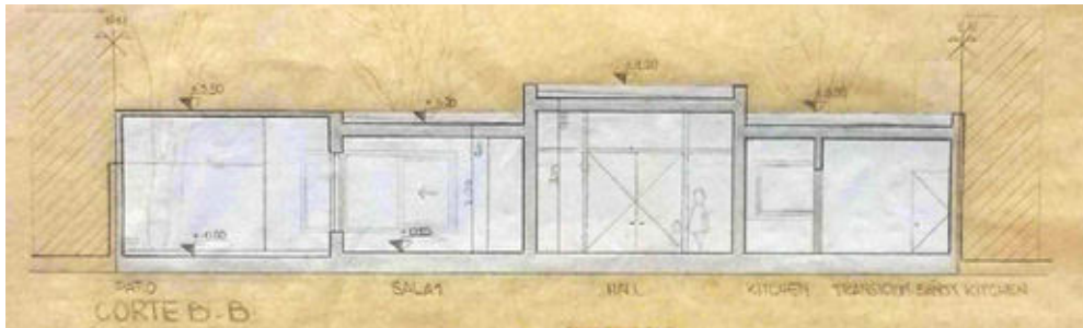
CORTE B-B TRANSVERSAL ESC 1:100
