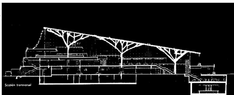
FIGURA No. 7. Corte esquemático aeropuerto Stuttgart
