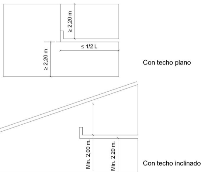
ALTURAS MINIMAS LOCALES CON ENTREPISO
