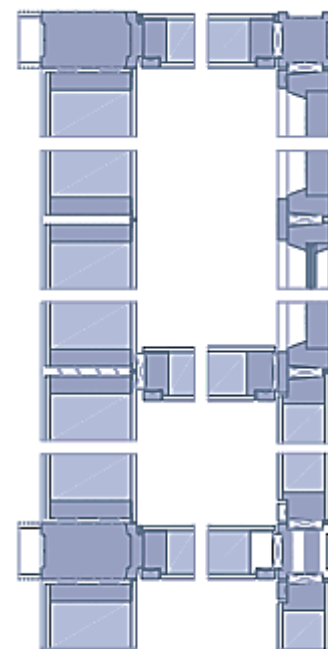
Detalle: sección horizontal
