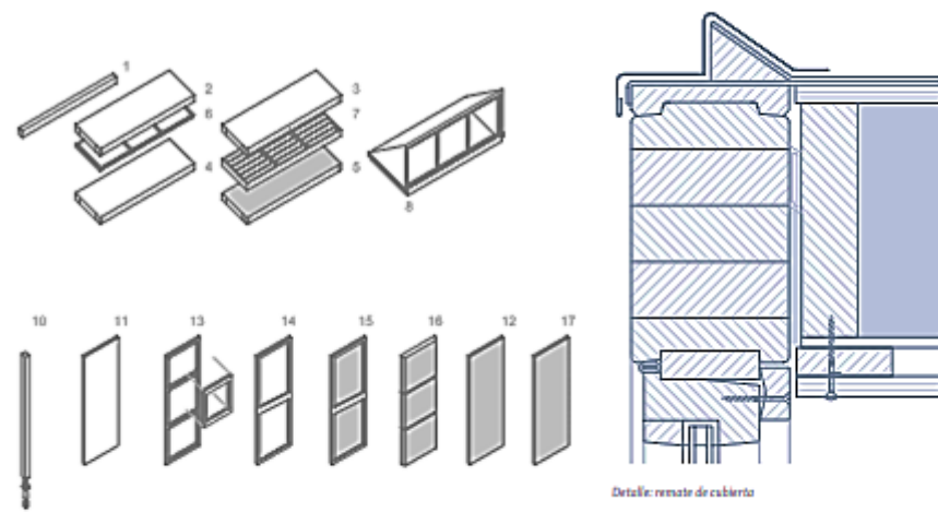
Sistema Modali: componentes horizontales y verticales
