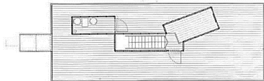
PLANTA SEGUNDO PISO
