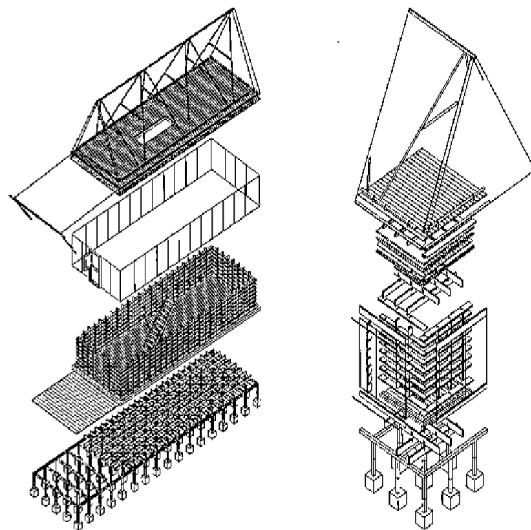
Fig.2: Axonometría Estructura-Estante y Fig. 3: Detalle Estructura-Estante [S. Radic, El Croquis,
