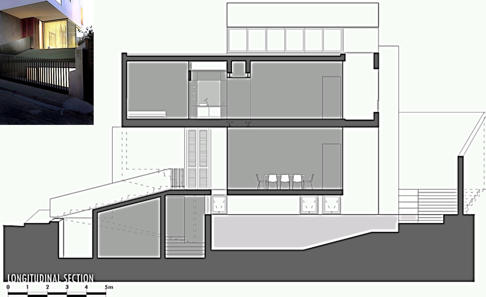
Fachada de escorzo y Corte Longitudinal con espacio distensivo o de trabajo junto a pileta
