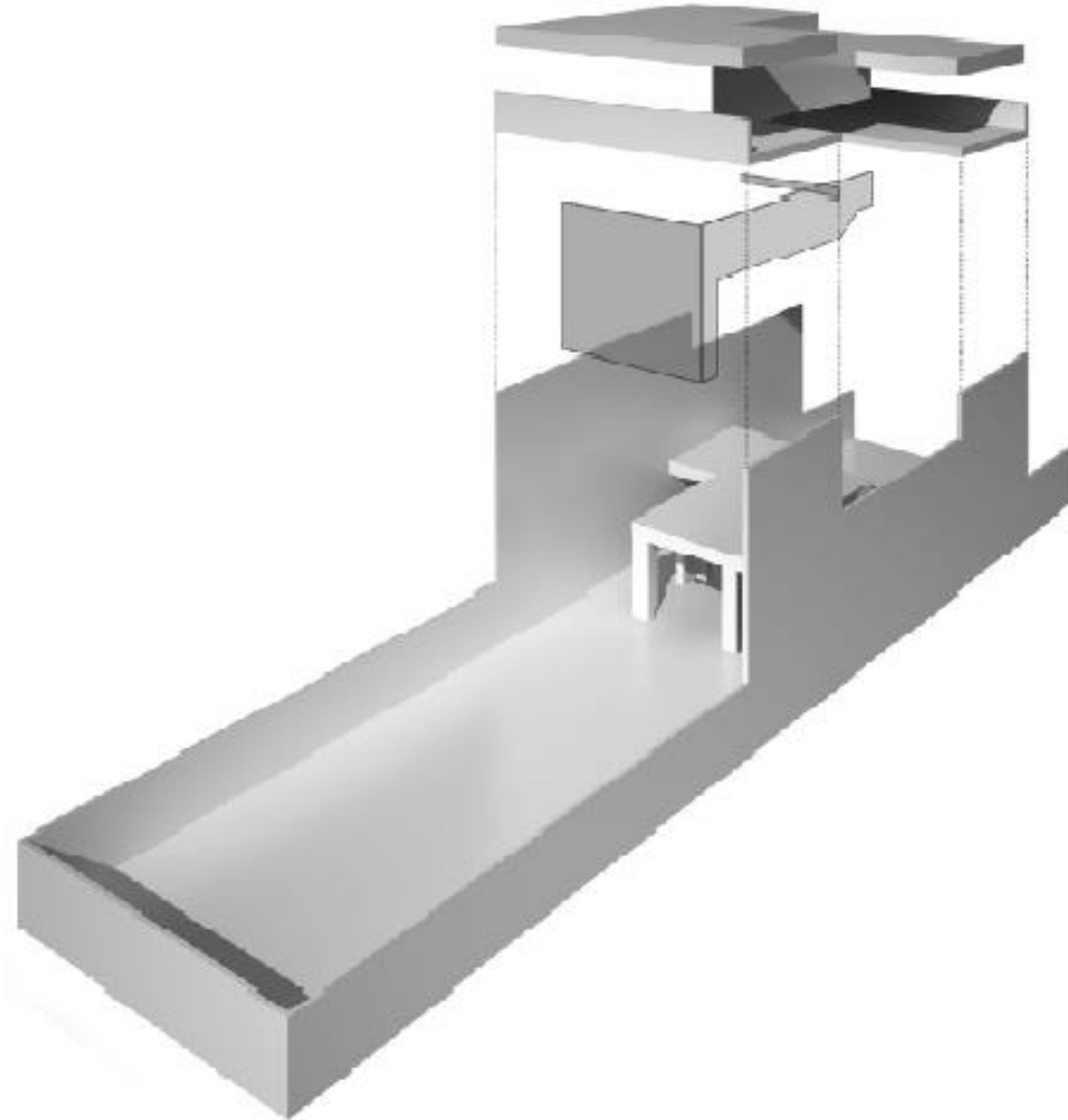
Despiece espacial
