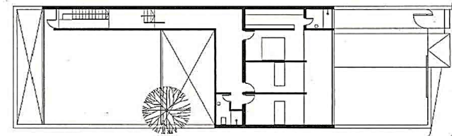
Planta alta
