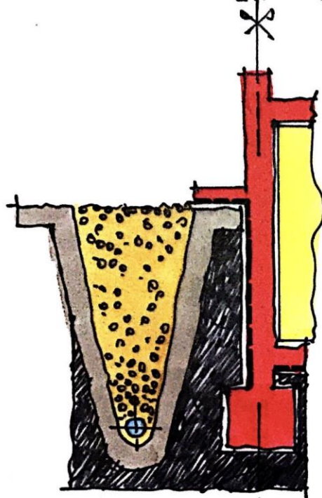
1 CUNA DRENANTE.
