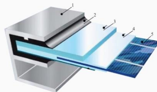
Fig. 09 - Detalle panel fotovoltaico con componentes.
