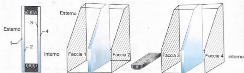
Fig. 10 - Esquematización de la numeración convencional de las caras de un vidrio aislante.
