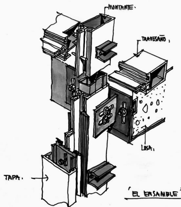
DETALLE DE ANCLAJE A LOSA, ( LATERAL ). UNION MONTANTE/TRAVESANO,
