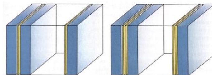
Fig. 12 - Esquema general de vidrios laminados.
