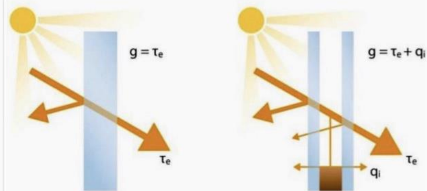
Fig. 07 - Factor solar g para vidrios simples o aislantes.
