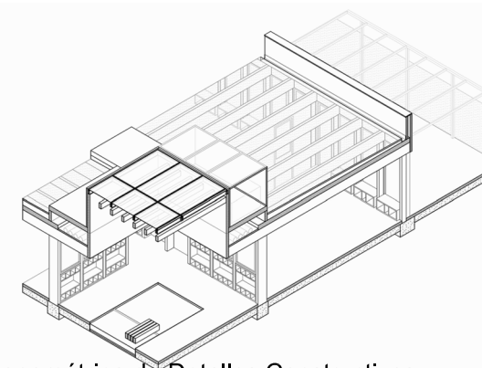
Axonométrica de Detalles Constructivos
