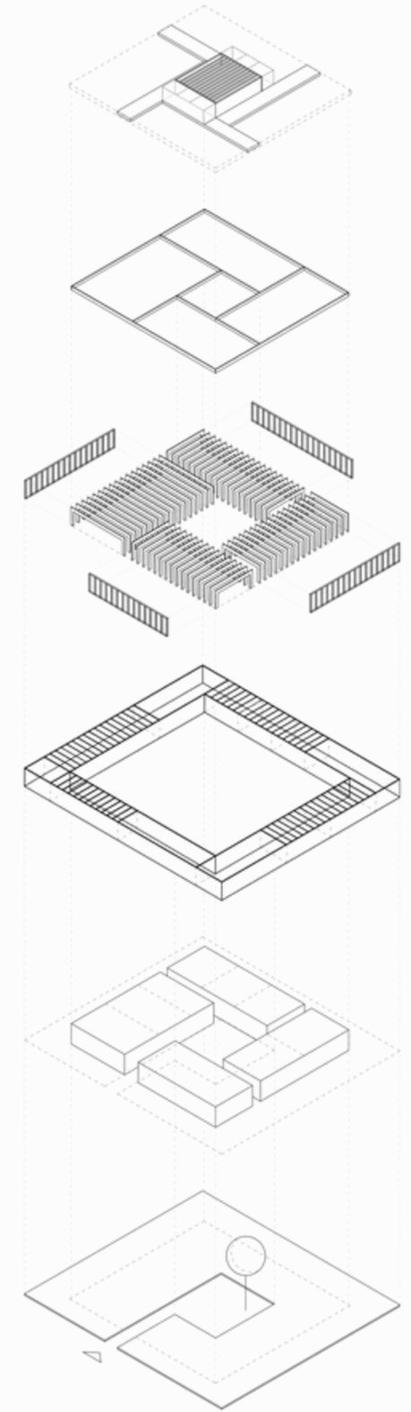
Despiece Axonométrico
