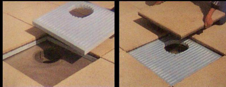
CUBIERTA INVERTIDA TRANSITABLE
