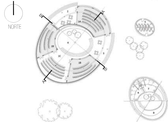
PLANTA BAJA
