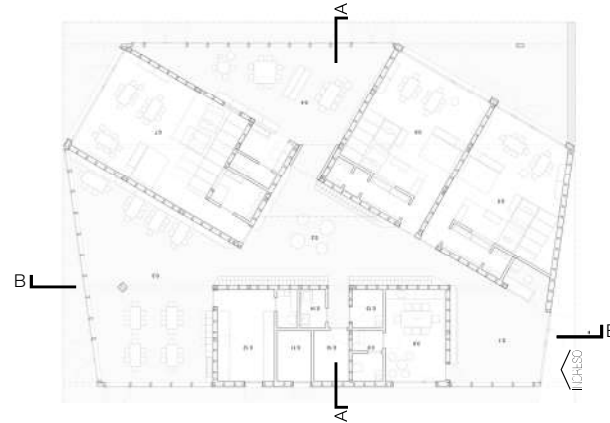
PLANTA BAJA
