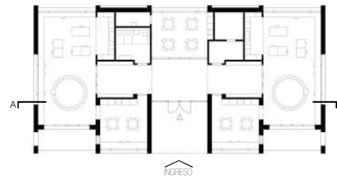
PLANTA BAJA
