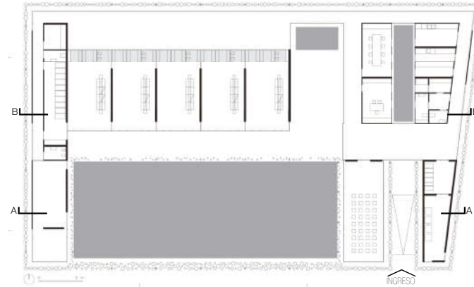
PLANTA BAJA
