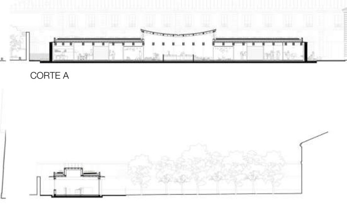
CORTE B
