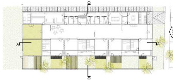
PLANTA BAJA
