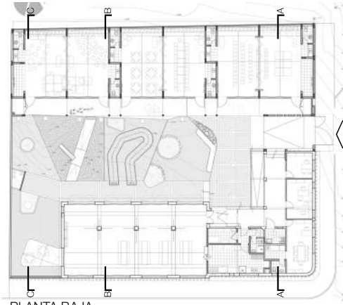
PLANTA BAJA
