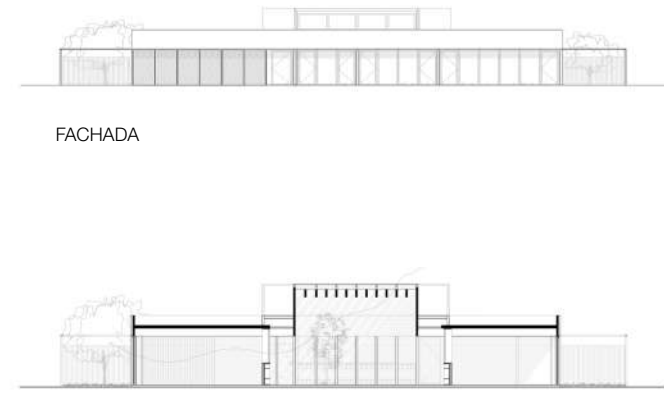
CORTE A
