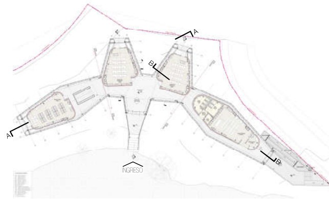
PLANTA BAJA
