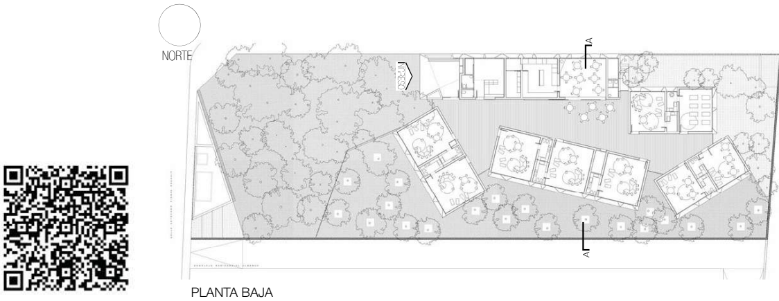
PLANTA BAJA
