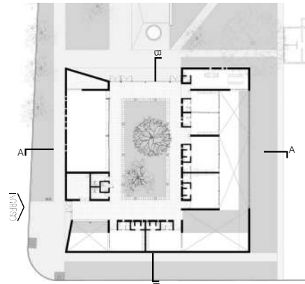
PLANTA BAJA
