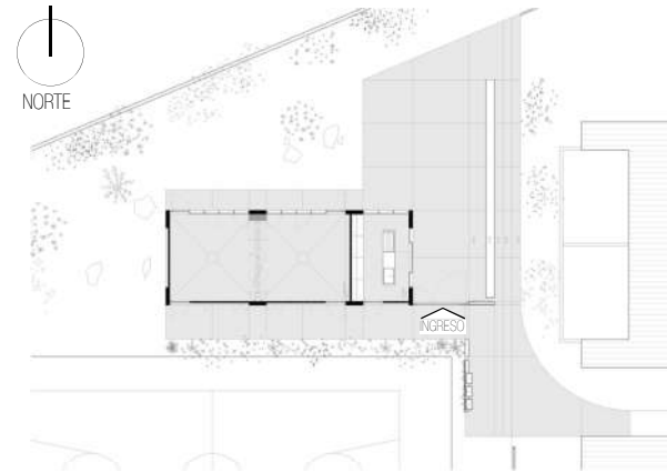
PLANTA BAJA y de EMPLAZAMIENTO
