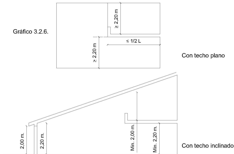
ALTURAS MINIMAS LOCALES CON ENTREPISO
