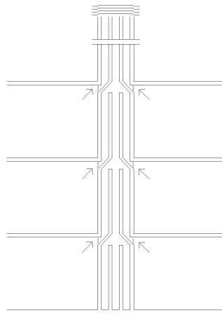
Gráfico 3.2.8.4.3.2.B CONDUCTOS UNIFICADOS
