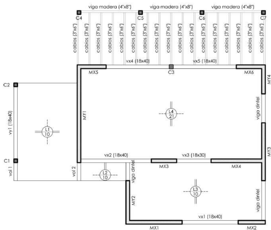
PLANTA ESTRUCTURA esc. 1:100
