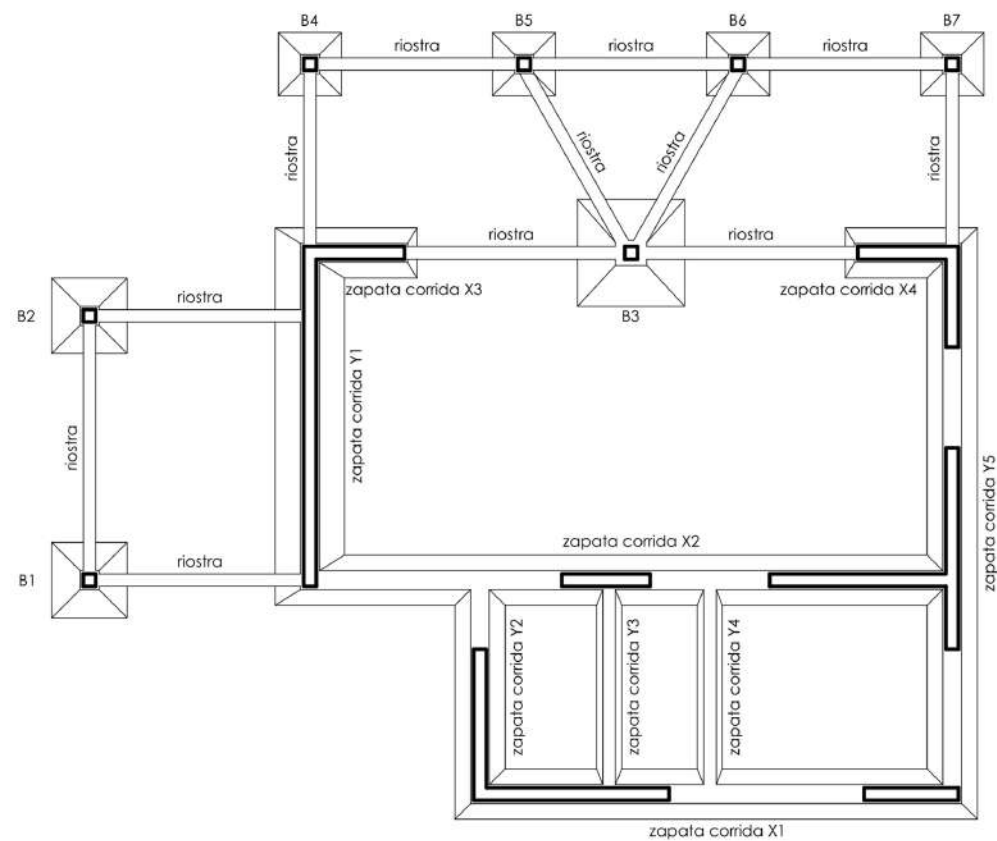
PLANTA FUNDACIONES ESC. 1:100
