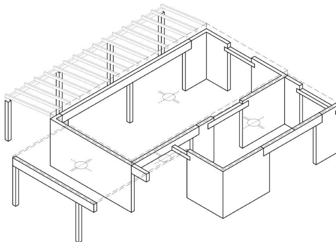
AXONOMÉTRICA DE LA ESTRUCTURA
