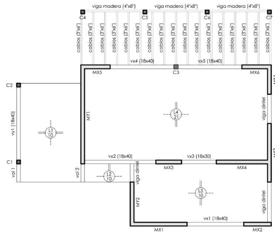
PLANTA ESTRUCTURAS ESC. 1:100
