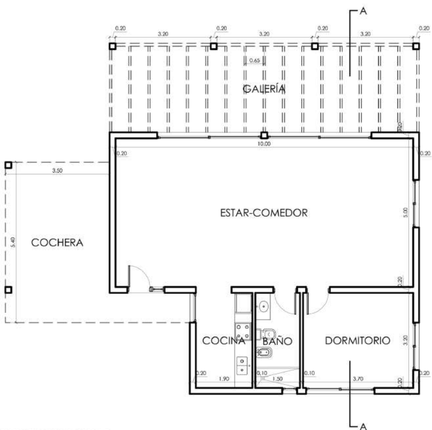
PLANTA ARQUITECTURA ESC. 1:100
