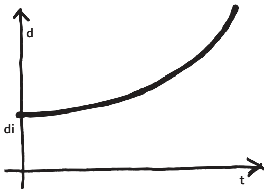
Representación gráfica del espacio recorrido en función del tiempo en un M.R.U.A.
