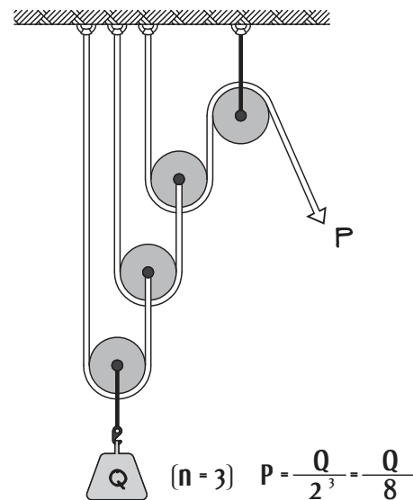
Aparejo Potencial
