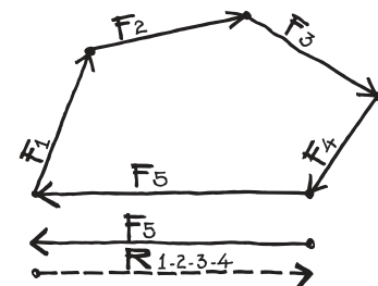
FIG.8- Fuerza Resultante
