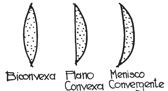
Tipos de Lentes Convergentes
