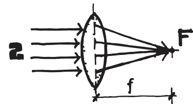
Tipos de Lentes Convergentes
