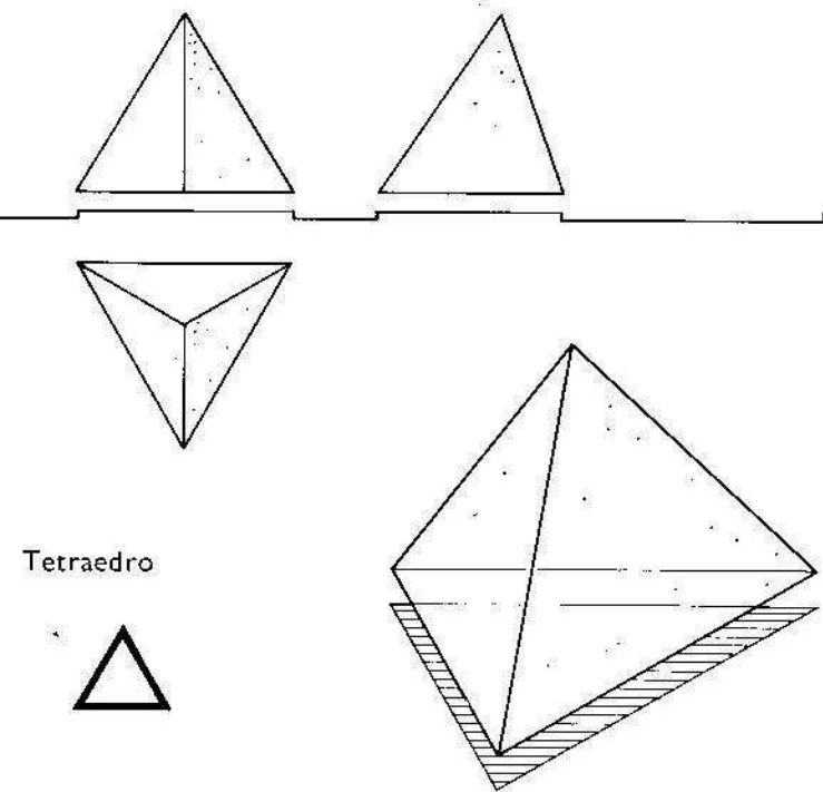
Tetraedro colocado sobre una cara.
