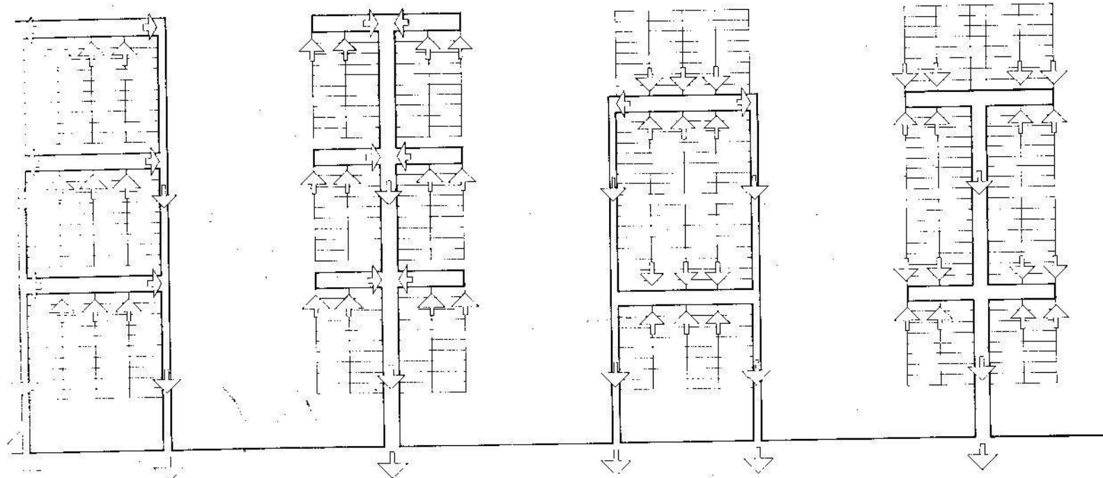
Sistemas para sustentación de pisos agrupados por intermedio de jácenas.
