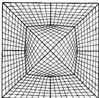
Doce superficies «hypar».
