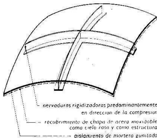
13) Lámina de acero compleja.
