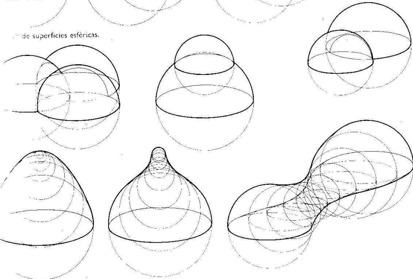
Fusión de superficies esféricas.
