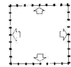
Sistema de tramos libres. Puntos de reunión de cargas en el contorno del edificio.
