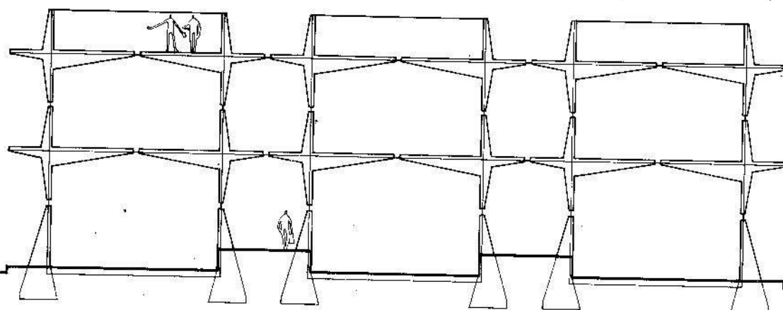
Sistema de pórticos de tres articulaciones con voladizos.
