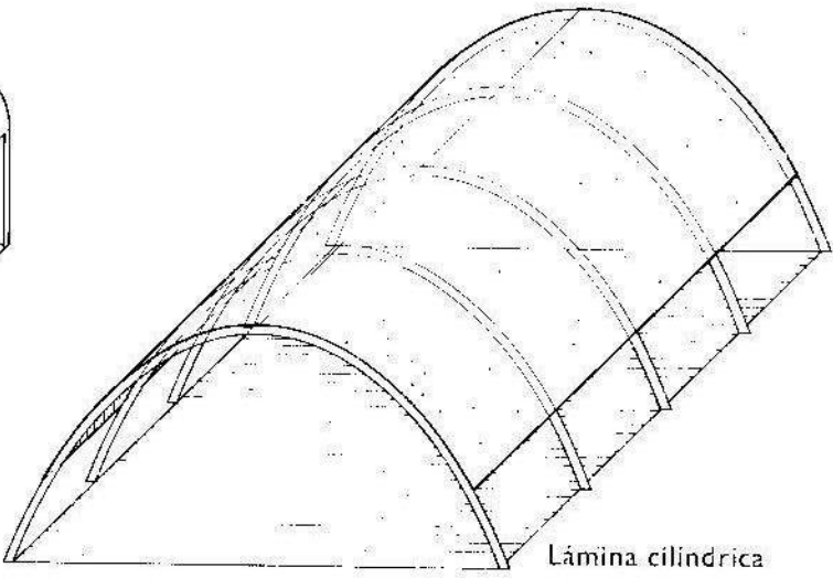
← Dirección de la luz mayor. → Sistema de extensión: continuidad de la unidad existente.
