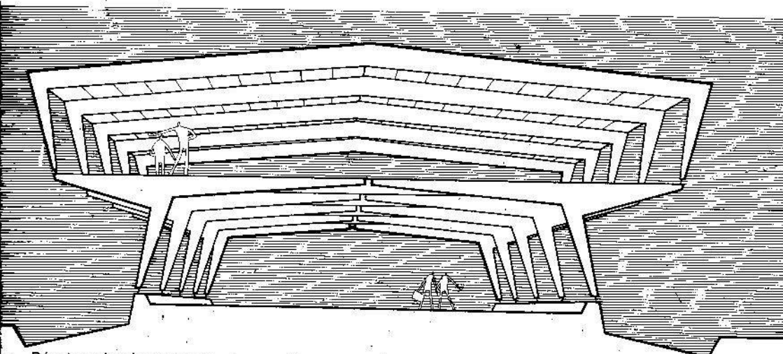
Pórtico de dos articulaciones dispuesto sobre voladizos de un pórtico de tres articulaciones.
