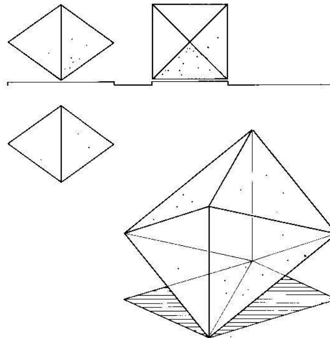
Octaedro colocado sobre una arista.
