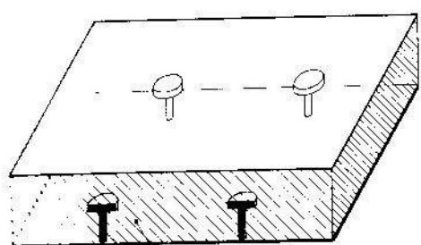
— losa de hormigón — perno soldado conector — chapa de acero actuando como encofrado y refuerzo exterior
