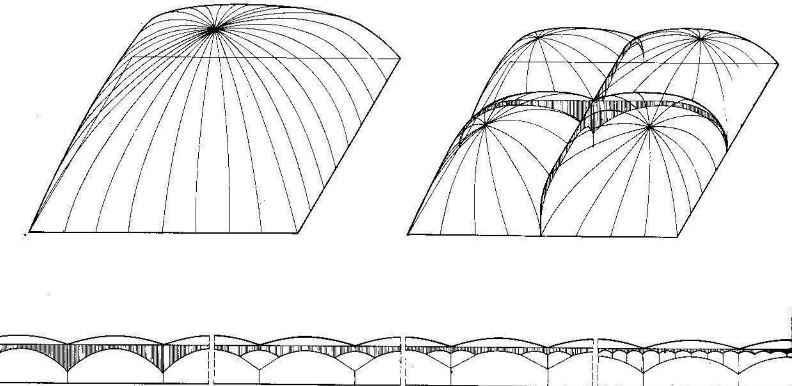
Esquema de nervios de membrana.
