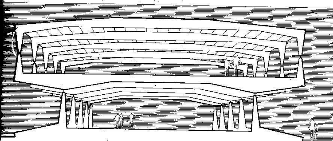
Pórtico de dos articulaciones dispuesto sobre otro pórtico de dos articulaciones invertido y articulado sobre los soportes.
