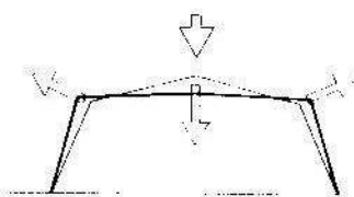
Descenso de la cumbrera.
