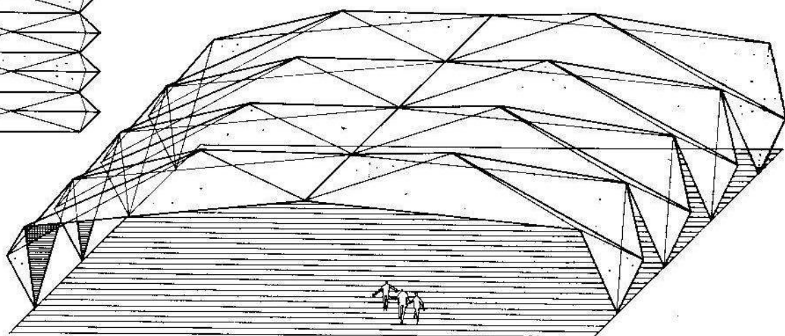
Pórtico de tres articulaciones: pliegue de cumbrera.
