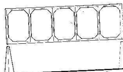
Marco de cinco paneles.
