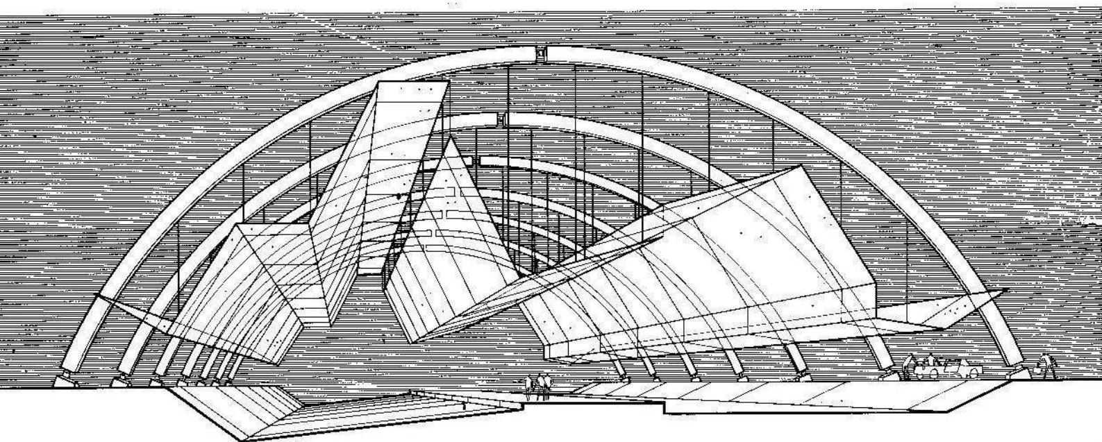
Ságita del arco = \frac{1}{3} de la luz.
