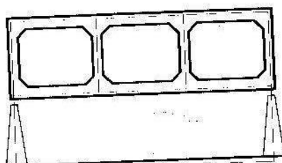
Forma estructural destacando el acartelamiento de los nudos.
