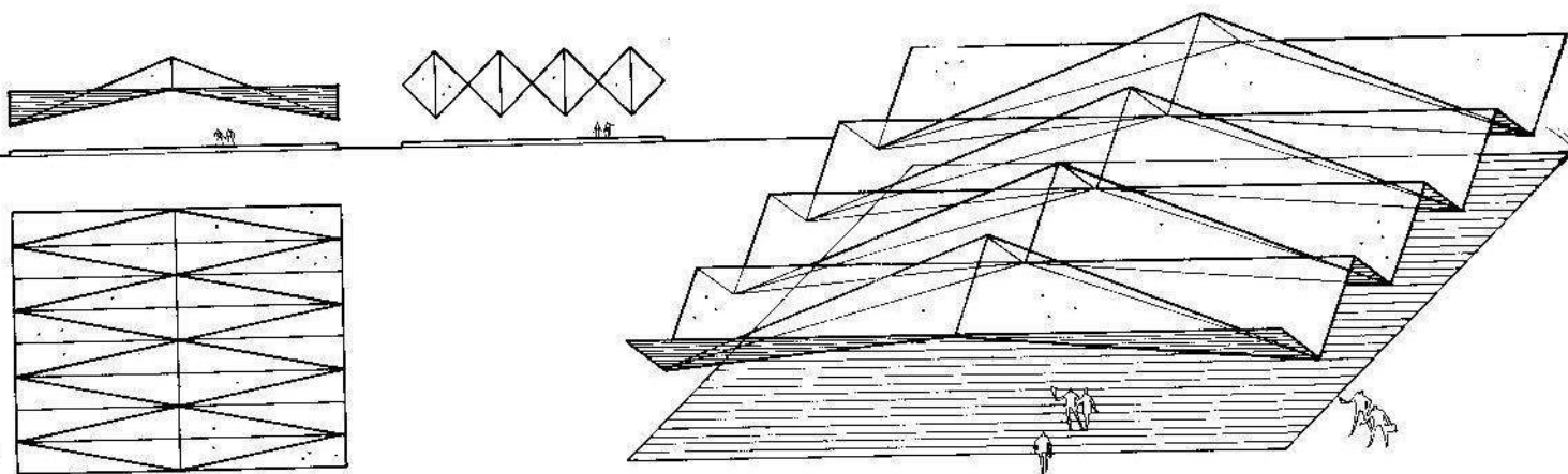
Pliegue de lima-tesa a lima-hoya.
