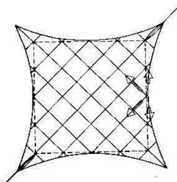
Cables de borde entre pilares venteados.
