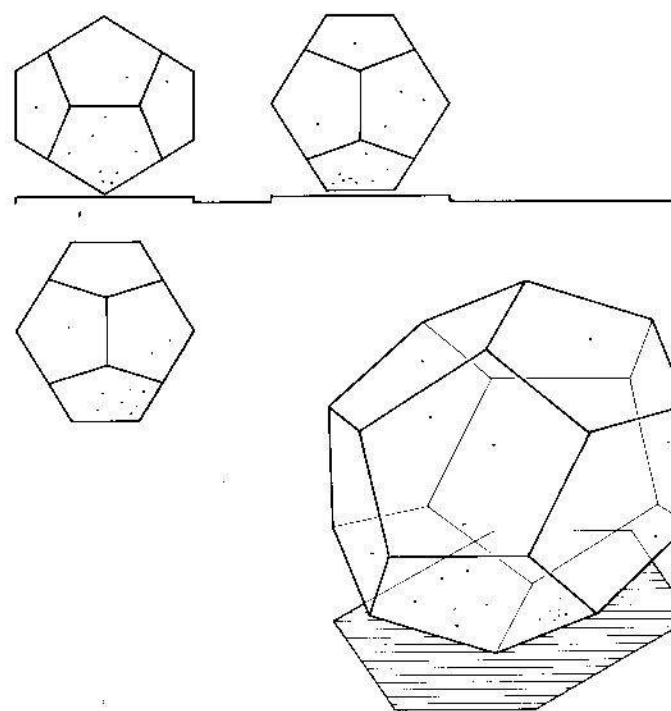
Dodecaedro colocado sobre una arista.
