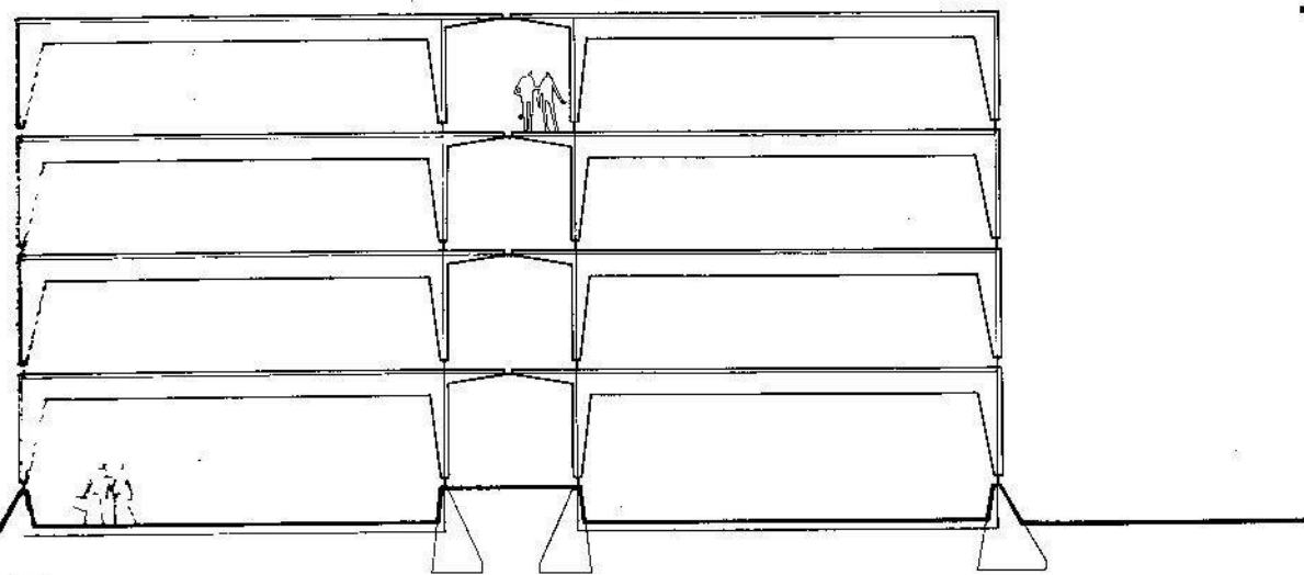
Sistema con pórticos de dos articulaciones.
