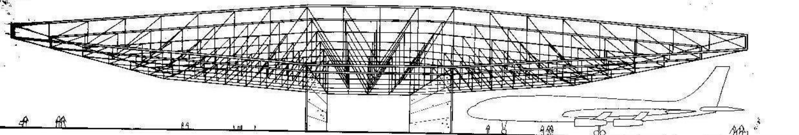
Cerchas con doble soporte en el centro: estructura en voladizo.
