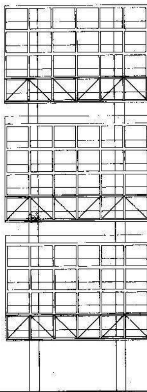
Elementos sustentadores de vector activo. Vigas trianguladas soportando cada una varios pisos.
