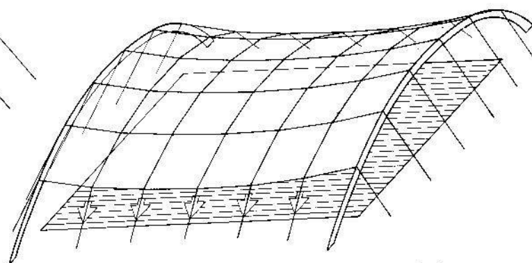
Estabilización mediante cables transversales anclados al suelo, con curvatura opuesta a la del cable portante.
