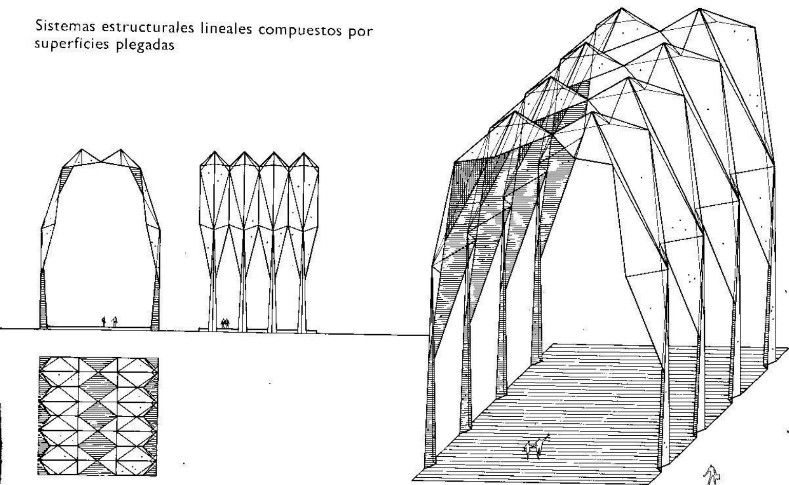
Arco con articulación en la clave.
