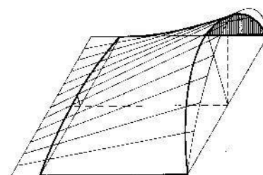
Unidad consistente en un conoide sobre cuatro soportes de esquina.
