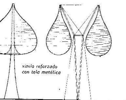
Membrana - depósito de agua.
