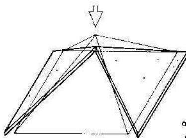
Corrimiento de los bordes inferiores.
