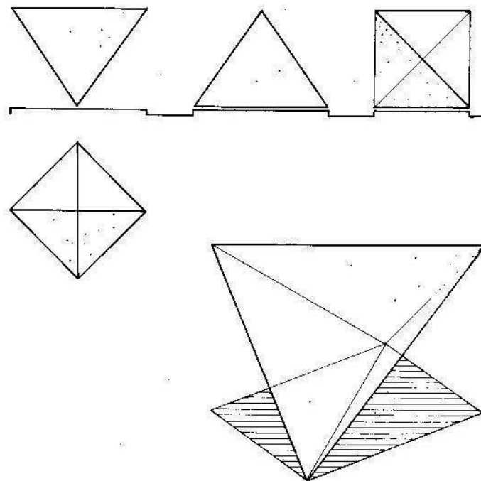
Tetraedro colocado sobre una arista.
