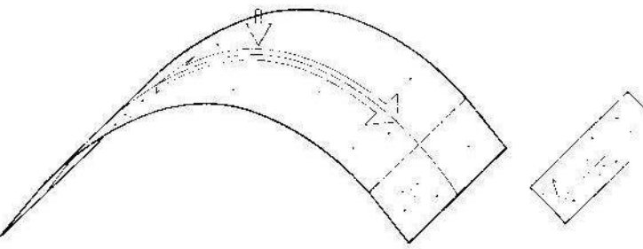
El mecanismo resistente descansa principalmente en la acción de placa. La acción de arco es menor y sirve para recibir cargas asimétricas.
