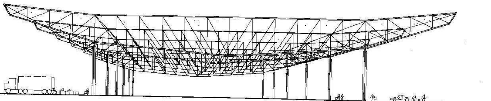
Cerchas con extremos en voladizo: estructura de luz libre, con voladizos.
