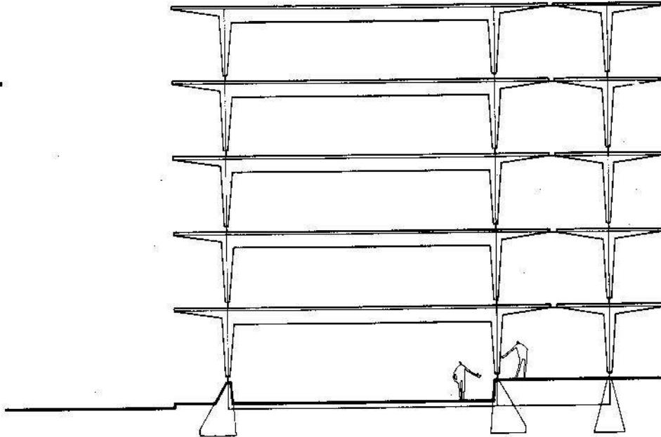
Sistema con pórticos de dos articulaciones y pórticos en T.
