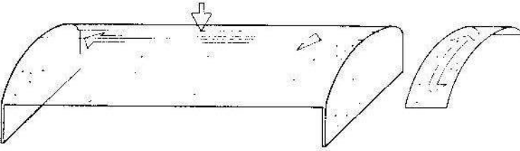
El mecanismo resistente descansa principalmente en la acción de arco (de ahí la forma de catenaria). La acción de placa es menor y sirve para recibir cargas asimétricas.
