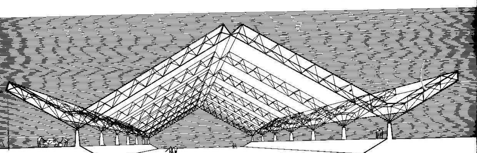
Estructura lineal triarticulada con voladizos.
