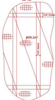
DETALLE DE EMPALME DE MALLAS ESC. 1:50
