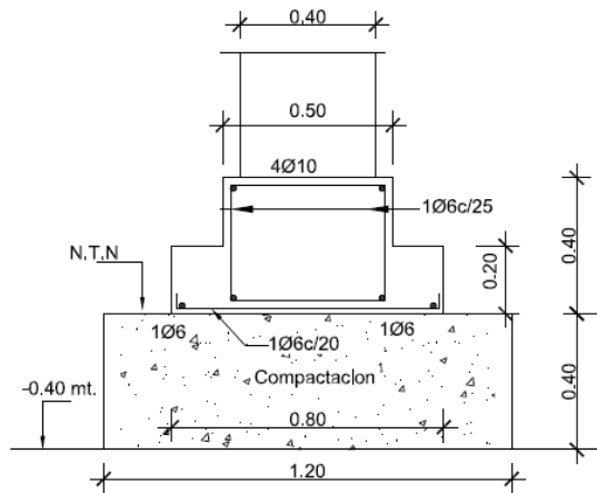
Zapata (ZC1)
