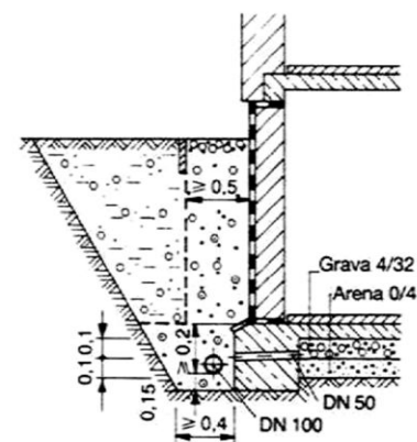
4 Sistema de drenaje con zanja
