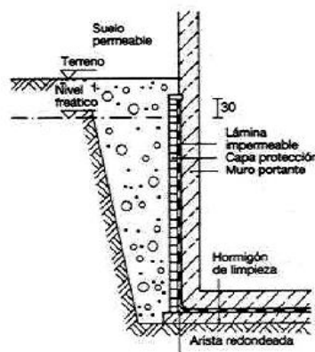
7 Impermeabilización resistente a la presión hidrostática
