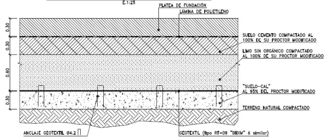
ESQUEMA DE MEJORAMIENTO DE SUELO
