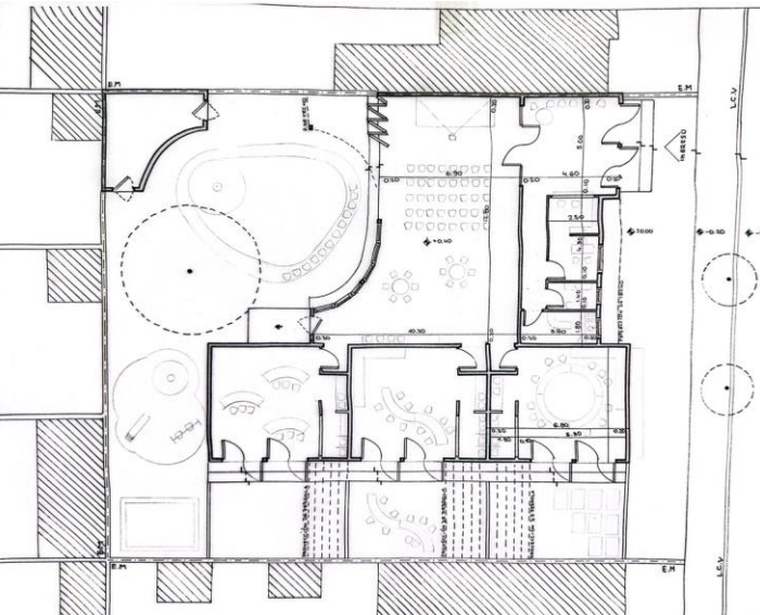
PLANTA esc 1:100
