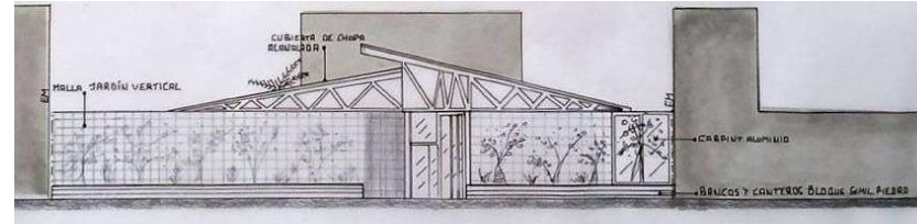
VISTA: FACHADA NOROESTE
