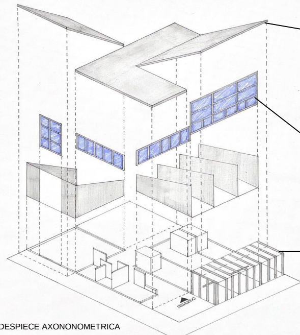
DESPIECE AXONOMETRICA
