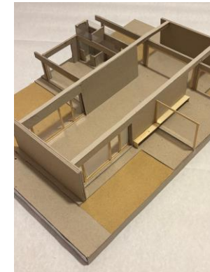
Esc. 1:50
