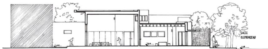
CORTE C-D ESC. 1:100
