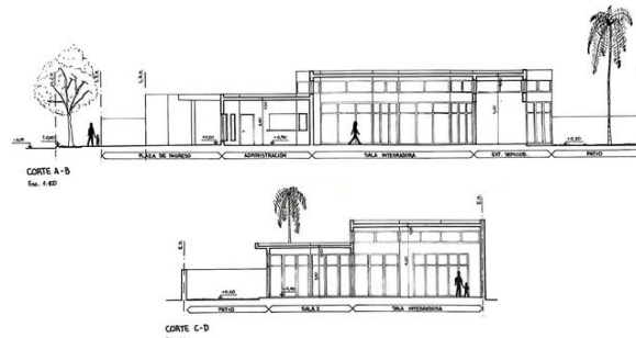
Cortes
