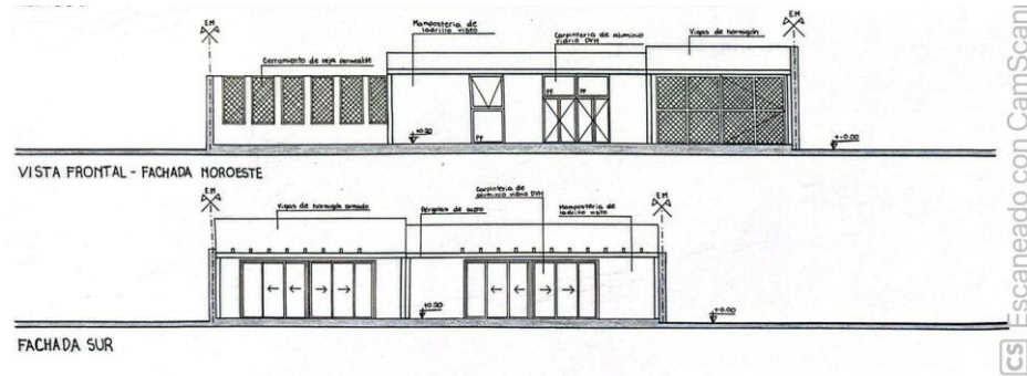
VISTAS
