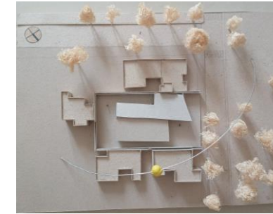
1:200
