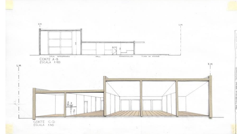
CORTES
