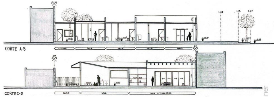
CORTES
