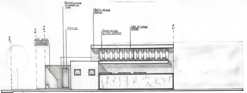
VISTA
