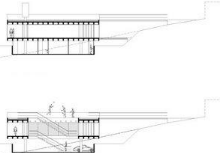
Cortes Transversais
