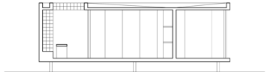
CORTE B
