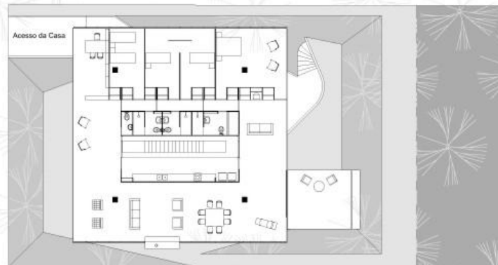
Planta Baixa - 1º Andar
