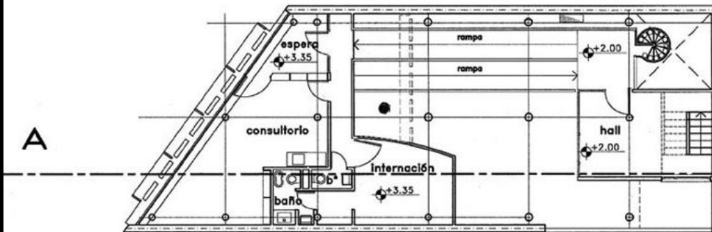
PLANTA ENTREPISO
