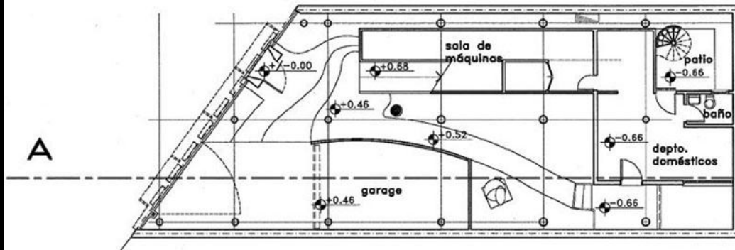
PRIMER PISO
