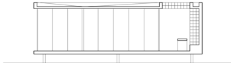
CORTE A
