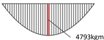
Diagrama de momento flector
