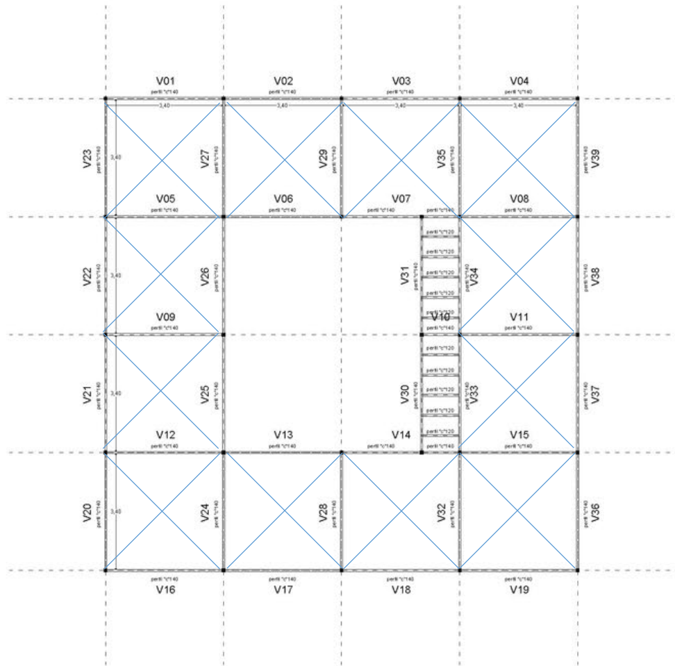
PLANTA ESTRUCTURA CUBIERTA (vigas)
