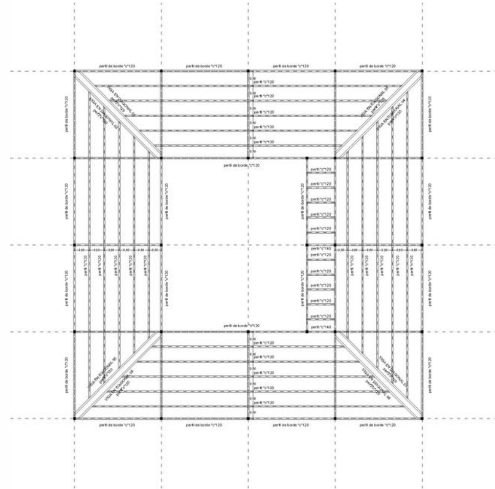
PLANTA ESTRUCTURA CUBIERTA (correas)
