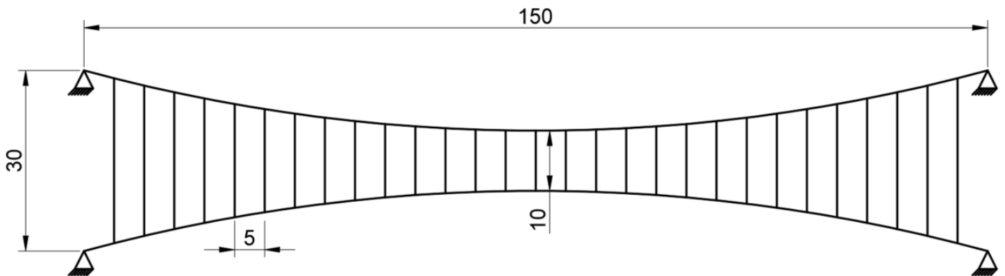
Geometría del doble cableado con cable estabilizante.
