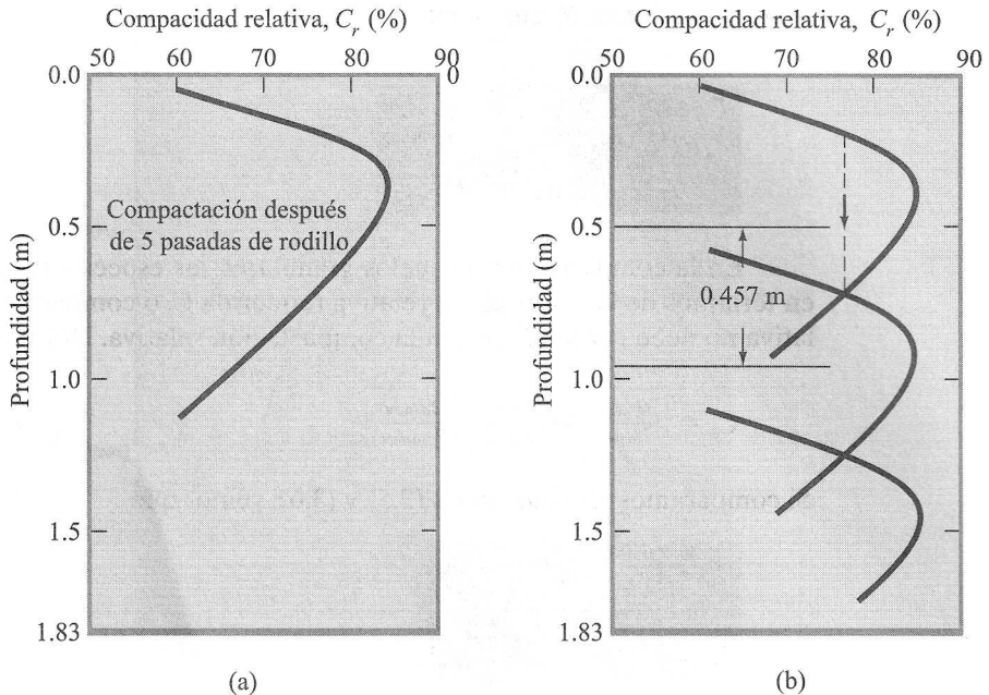
FIGURA 3.16 Estimación del espesor de la capa de compactación para una compacidad relativa mínima requerida de 75% con cinco pasadas de rodillo (según D'Appolonia, Whitman y D'Appolonia, 1969).
