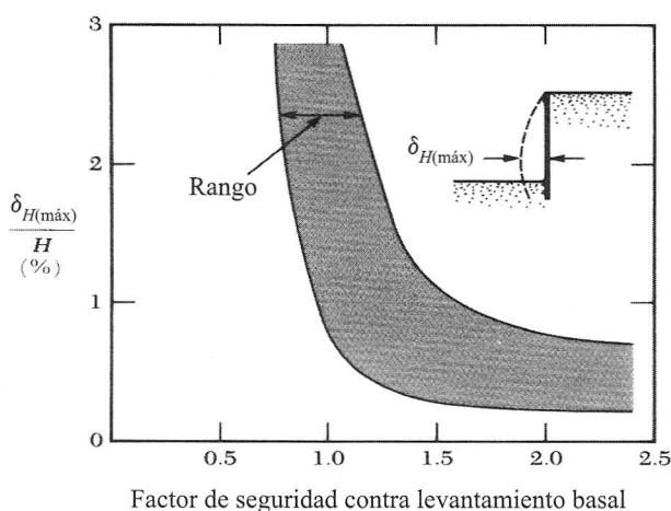
FIGURA 12.27 Rango de variación de \delta_{H(\text{máx})}/H con FS versus levantamiento basal de observaciones de campo (según Mana y Clough, 1981).
