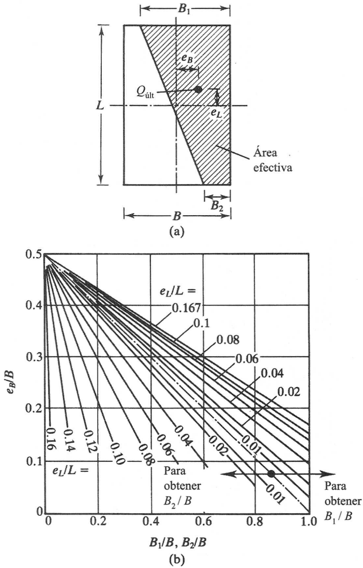
FIGURA 11.11 Área efectiva para el caso e_L/L < \frac{1}{6} y 0 < e_B/B < 0.5 (según Hightler y Anders, 1985).
