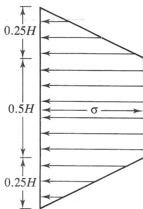
FIGURA 12.17 Envolvente de la presión aparente de Peck (1969) para cortes en arcilla dura.
