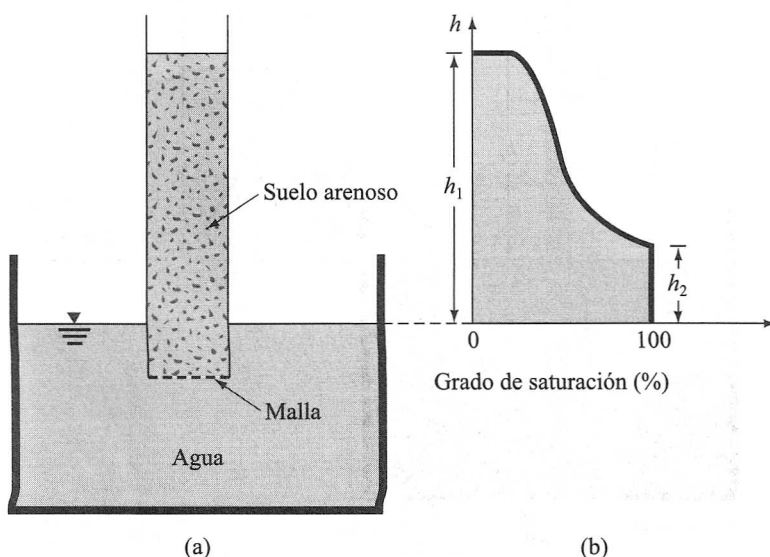
FIGURA 4.19 Efecto de capilaridad en suelo arenoso; (a) una columna de suelo en contacto con agua; (b) variación del grado de saturación en la columna de suelo.
