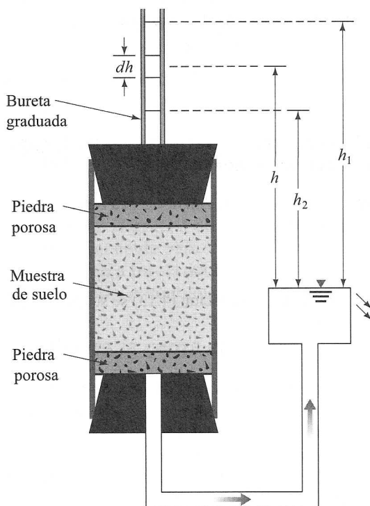
FIGURA 4.5 Prueba de permeabilidad bajo carga variable.
