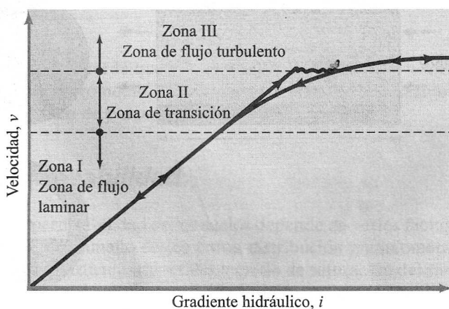
FIGURA 4.2 Naturaleza de la variación de v con el gradiente hidráulico i .
