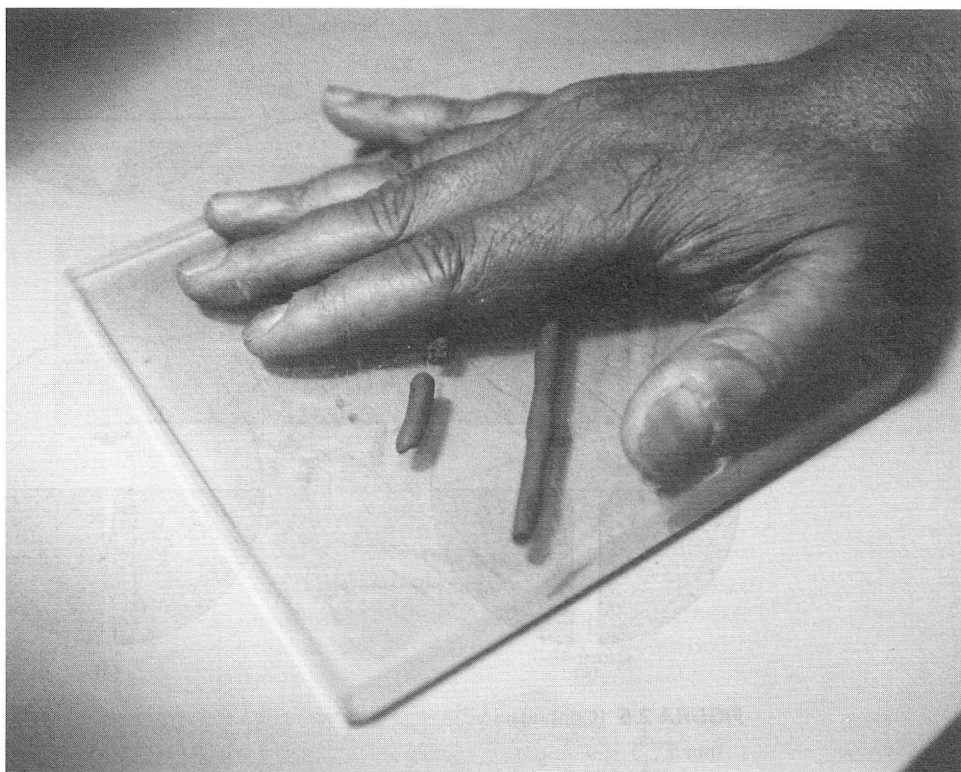
FIGURA 2.7 Prueba del límite plástico.
