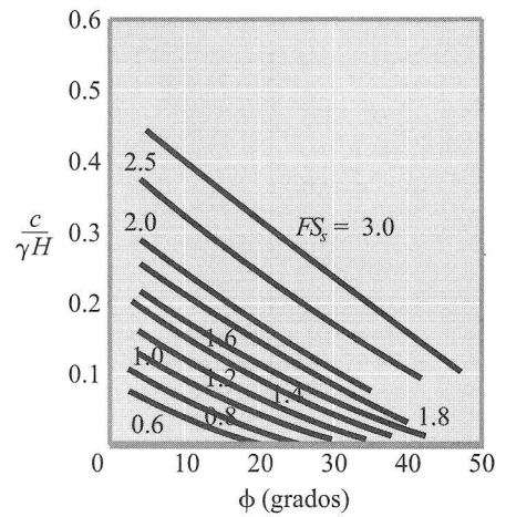
(d) Talud: vertical 1, horizontal 1.5
