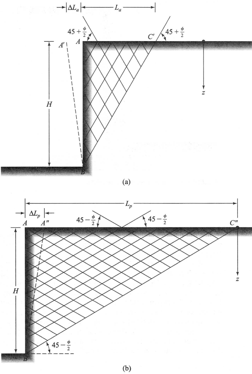
FIGURA 9.7 Rotación de un muro sin fricción respecto al fondo.
