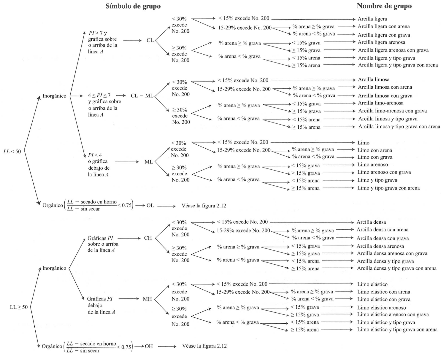
Figura 2.14 Diagrama de flujo para nombres de grupo de suelos limosos, inorgánicos y arcillosos (según ASTM, 1998).
