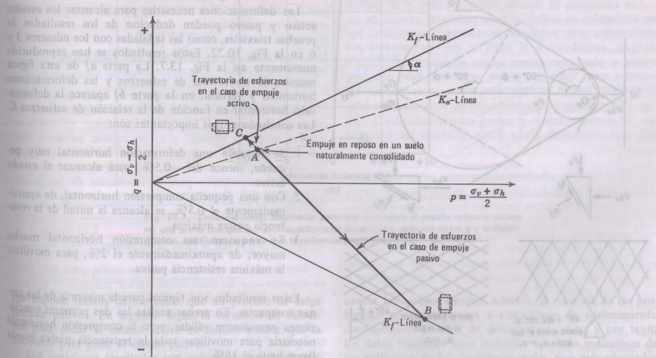
Fig. 13.4. Trayectorias de esfuerzos para los estados activo y pasivo de Rankine.
