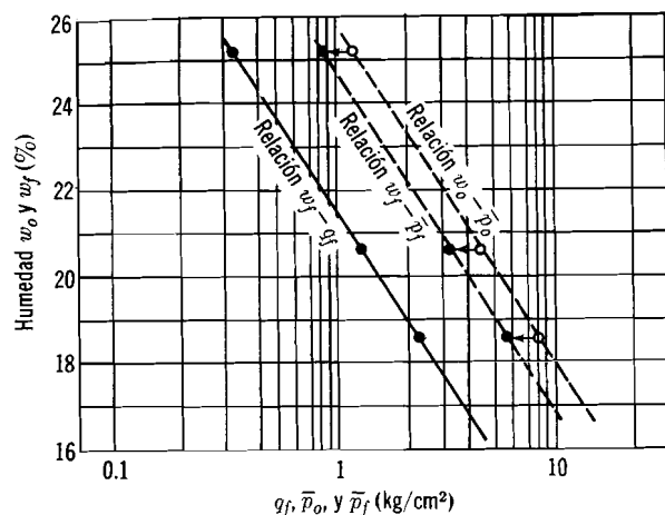
Fig. 28.10. Relación esfuerzo-volumen en arcilla de Weald normalmente consolidada.
