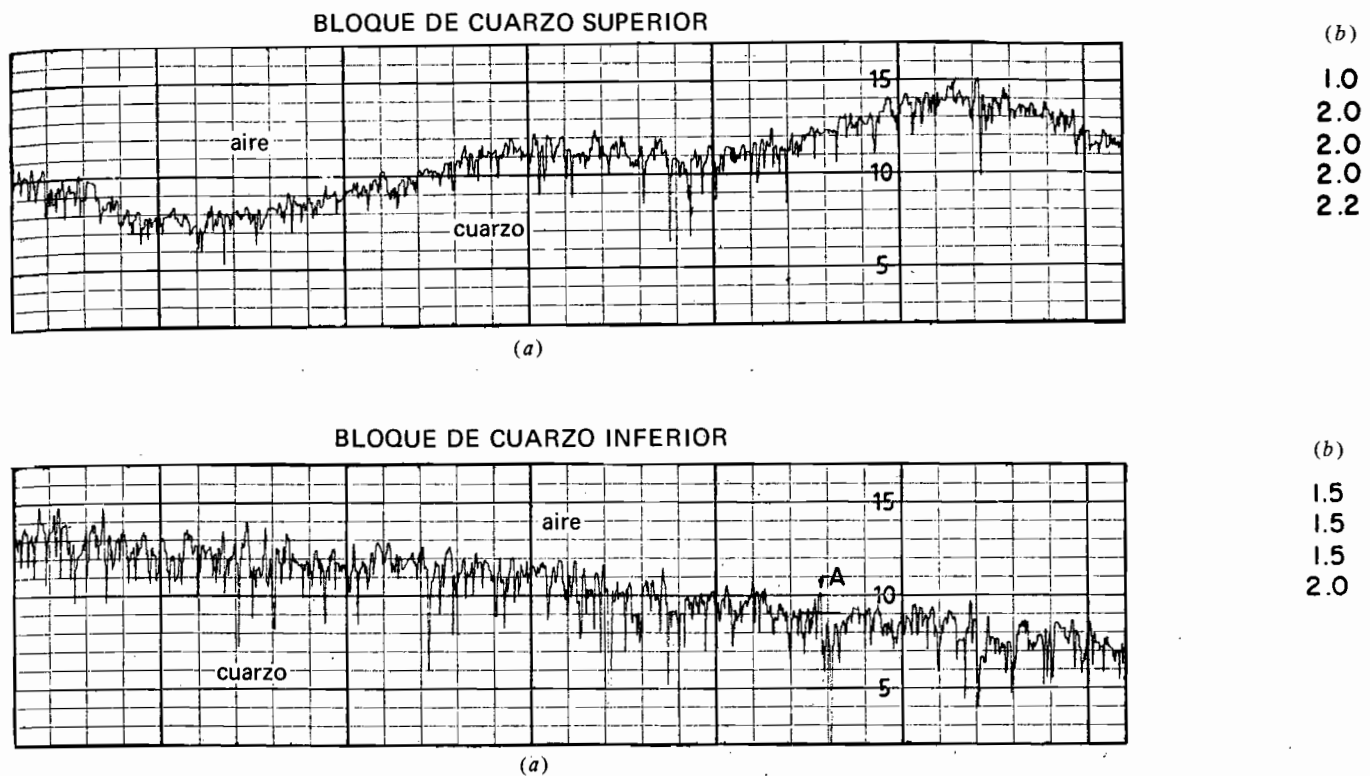
Fig. 6.3. Perfil de superficies de cuarzo "lisas". a) Perfil superficial. Escala vertical: 1 división = 5 \times 10^{-6} cm; horizontal, 1 división = 5 \times 10^{-3} cm. b) Rugosidad media en el eje, en 2.5 \times 10^{-6} cm. (Según Dickey, 1966.)
