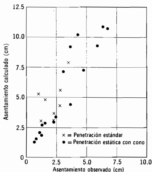
Fig. 14.29. Comparación entre los asentamientos calculados y los observados en zapatas cimentadas sobre arena y grava (Según Meyerhof, 1965).
