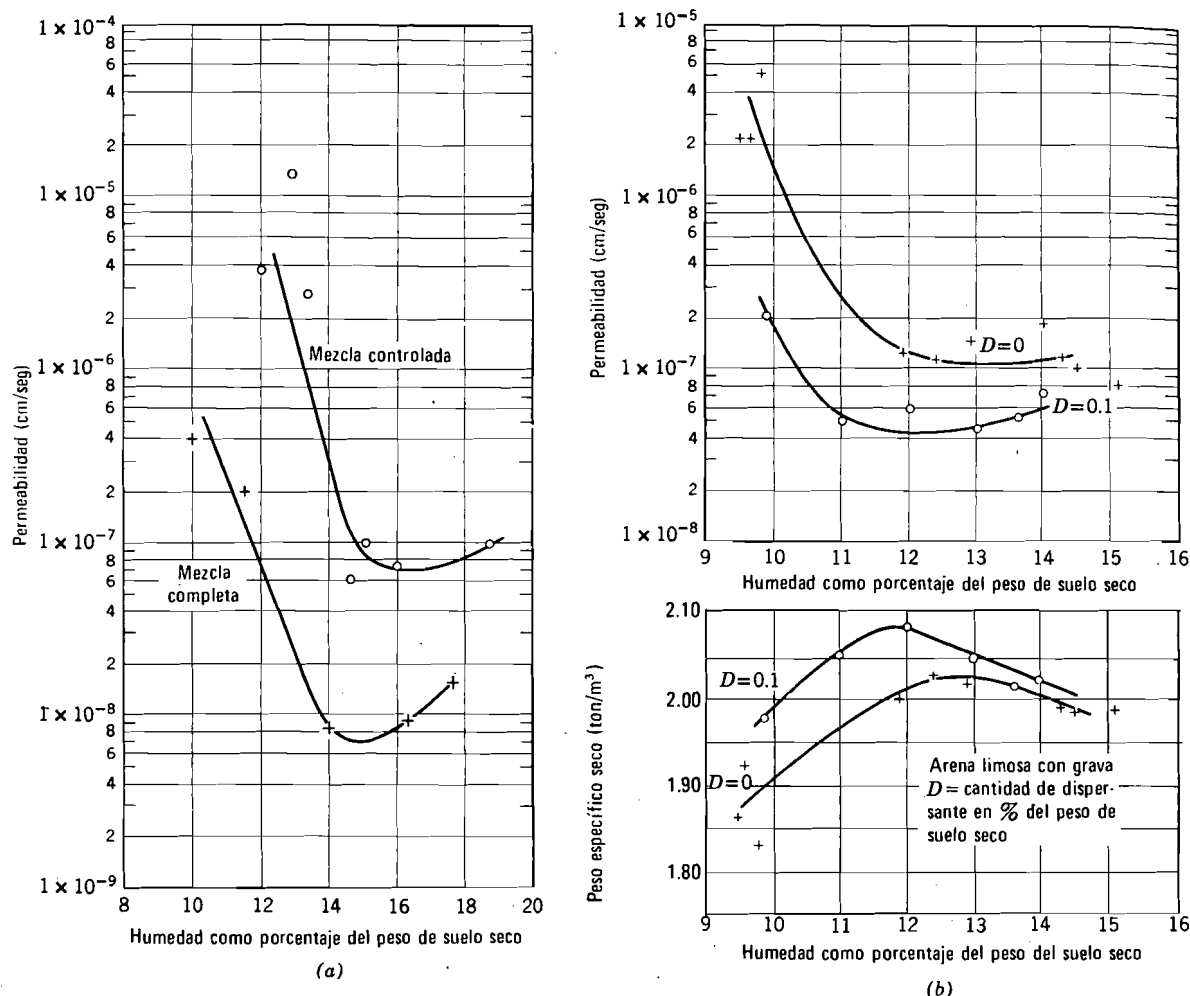
Fig. 19.11. Influencia de la estructura sobre la permeabilidad. a) Influencia del mezclado. Arcilla de Jamaica. b) Influencia de la dispersión. (Según Lambe, 1955).
