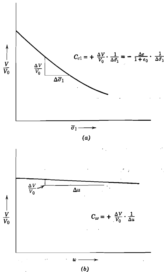
Fig. 26.5. Deformación unidimensional (a) Esqueleto mineral. (b) Agua.
