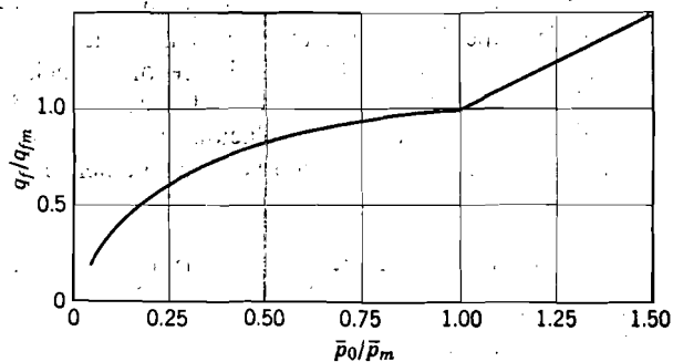
Fig. 29.20. Relación entre la resistencia al corte sin drenaje y la razón de sobreconsolidación.
