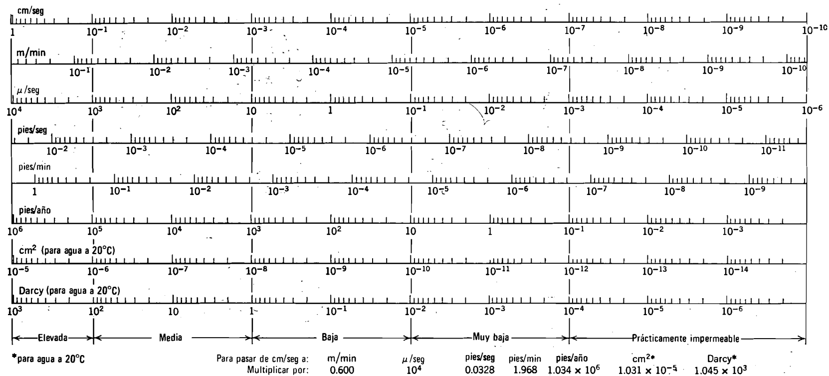
Fig. 19.6. Escalas para transformación de unidades de permeabilidad.
