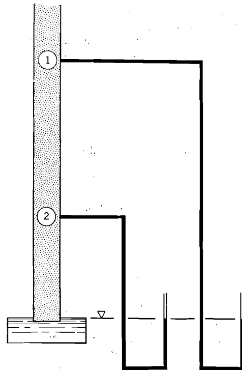
Fig. 16.5. Presiones en el agua capilar.
