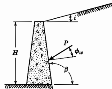
Fig. 13.21. Expresión de Coulomb para el caso de un muro con fricción y terreno de superficie del relleno inclinada.
