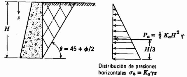
Fig. 13.9. Empuje activo en el caso sencillo de Rankine.
