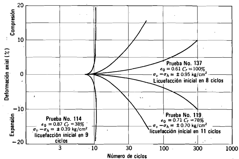
Fig. 29.10. Deformación axial en función del número de ciclos de carga para arenas saturadas con diversas compacidades iniciales, Arena del río Sacramento, \bar{\sigma}_v = 1 \text{ kg/cm}^2 (Según Seed y Lee, 1966).
