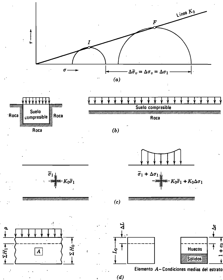
Fig. 25.8. Asentamiento unidimensional. (a) Deformación unidimensional. (b) Asentamiento unidimensional impuesto por las condiciones de contorno. (c) Asentamiento unidimensional bajo esfuerzos K_0 . (d) Asentamiento.
