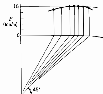
Fig. E23.6-5. Forma adecuada de representar los datos correspondientes a varios \theta .
