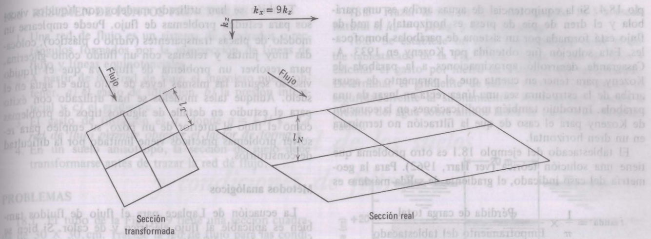
Fig. 18.6. Parte de una red de flujo en un suelo anisótropo.
