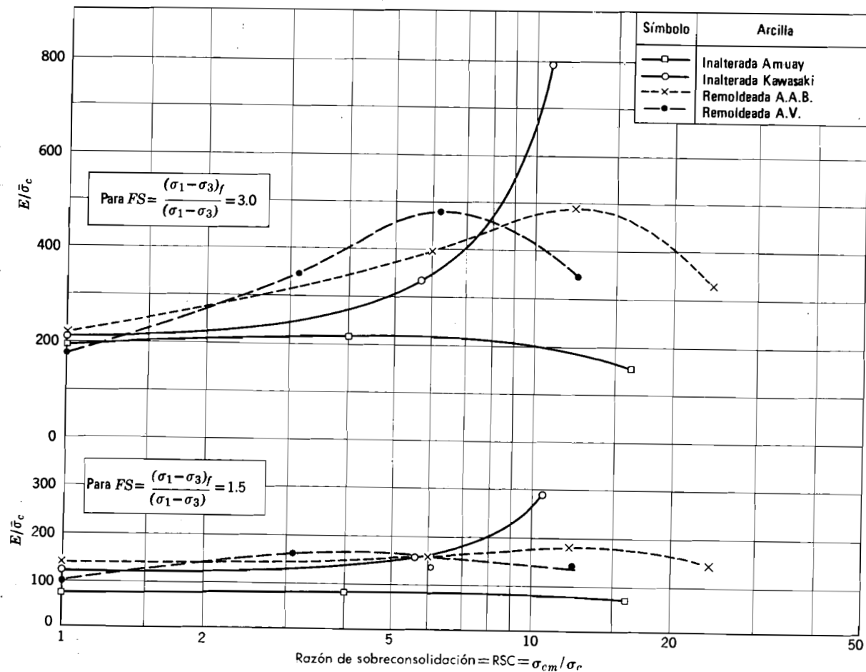
Fig. 30.6. Efecto de la sobreconsolidación sobre el módulo (Según Ladd, 1964).
