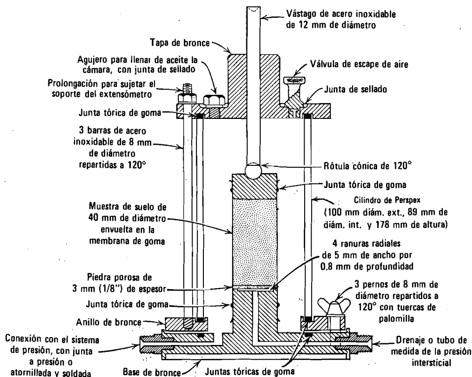
Fig. 9.5. Sección de una cámara triaxial típica. (Según Bishop y Henkel, 1962).
