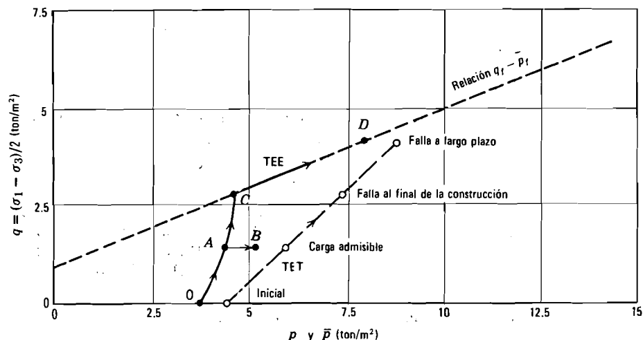
Fig. E31.3-2. Esfuerzos y presiones en z = 2.25 \text{ m} .
