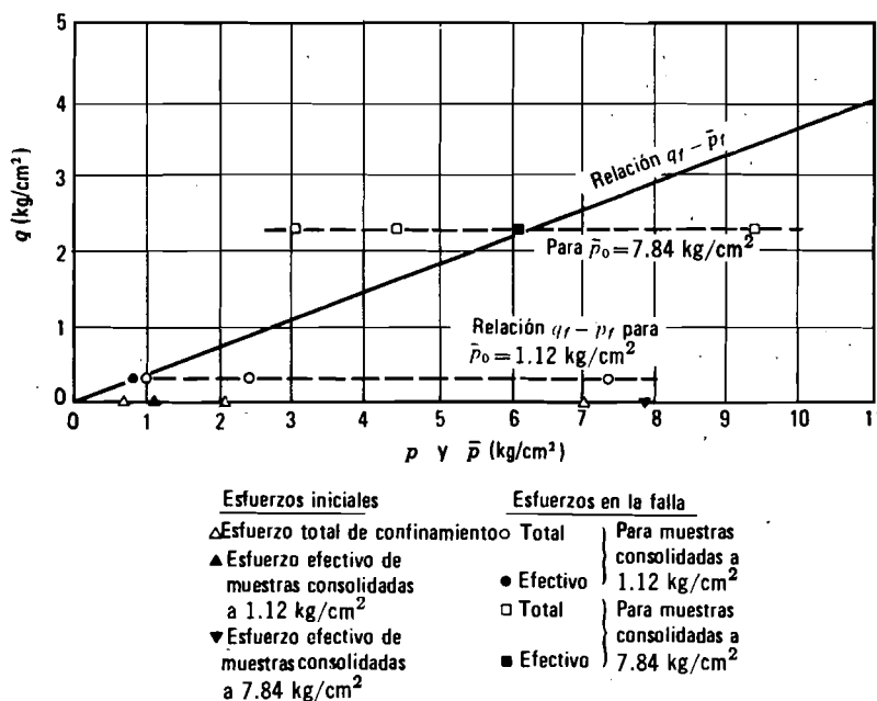
Fig. 28.13. Dos series de pruebas SCSD en arcilla de Weald normalmente consolidada.
