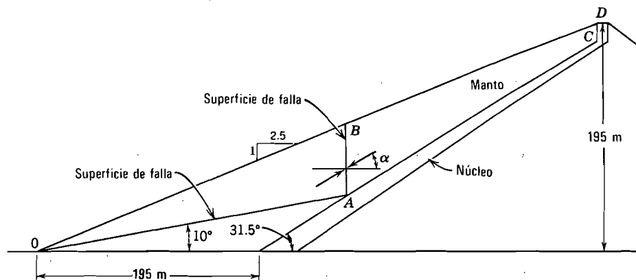
Fig. E24.61. Manto: \phi = 40^\circ , \gamma = 1.75 \text{ ton/m}^3 ; Núcleo: c = 10 \text{ ton/m}^2 ; sin presiones intersticiales.
