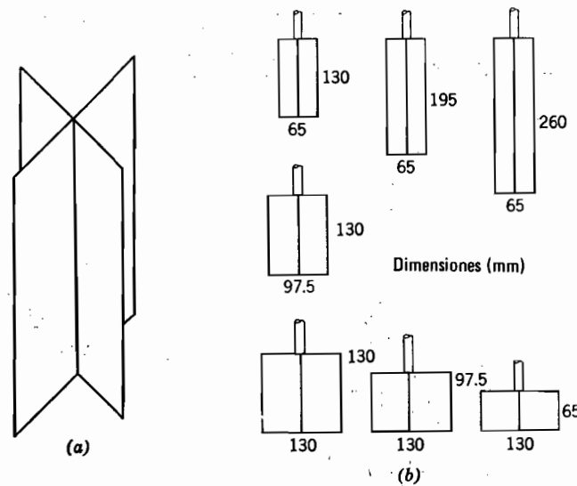
Fig. 7.6. Veletas o Molinetes. a) Sonda de veleta. b) Veletas estudiadas por Aas (1965).
