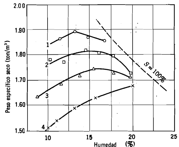
Fig. 34.3. Curvas de compactación estática de una arcilla limosa. (1) 140 kg/cm 2 de carga estática. (2) 70 kg/cm 2 de carga estática. (3) 35 kg/cm 2 de carga estática. (4) 14 kg/cm 2 de carga estática. Nota. Compactación por la cara superior de la muestra solamente. (Según Turnbull, 1950).
