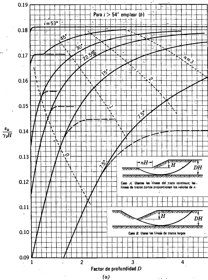
Fig. 31.1. Gráficas de estabilidad para \phi = 0 . (Taylor, 1948).
