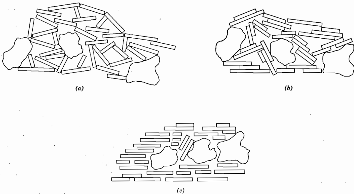
Fig. 7.2. Estructura de un suelo natural a) Depósito inalterado en agua salada. b) Depósito intacto en agua dulce. c) Suelo remoldeado.
