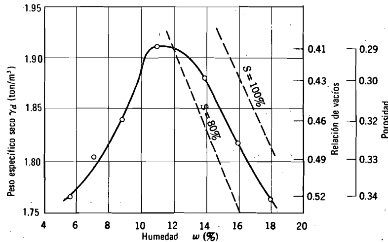
Fig. 34.1. Prueba de compactación Proctor estándar (Según Lambe 1951).
