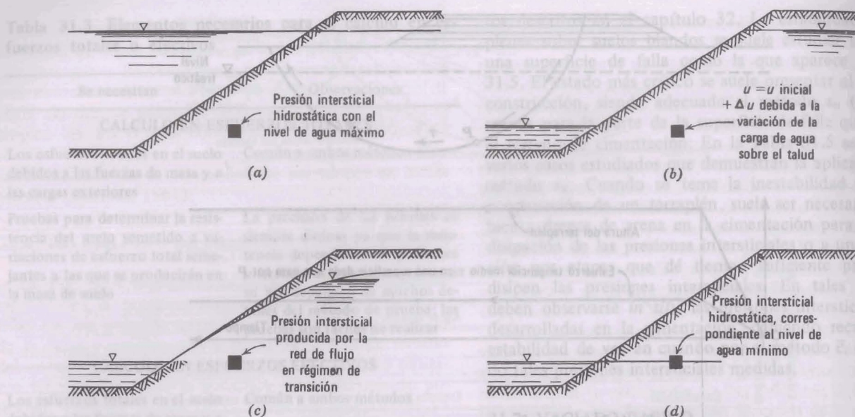
Fig. 31.6. Comportamiento de un talud en un vaciado rápido. a) Estado inicial de equilibrio. b) Después del vaciado pero antes de reajustarse las presiones. c) Después del reajuste de presiones. d) Estado de equilibrio final.
