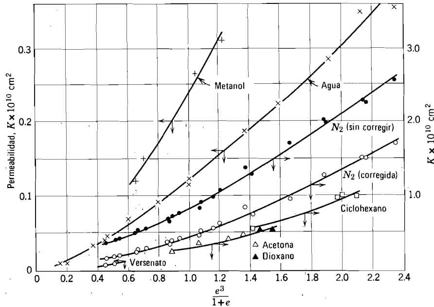
Fig. 19.7. Permeabilidad de la caolinita a distintos fluidos en función de e^3/(1+e) siendo e = relación de vacíos. (Según Michaels y Lin, 1954.)
