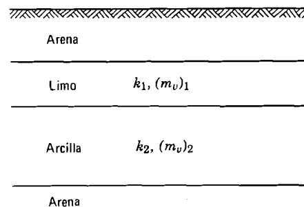
Fig. 27.8. Problema de consolidación con dos estratos compresibles.
