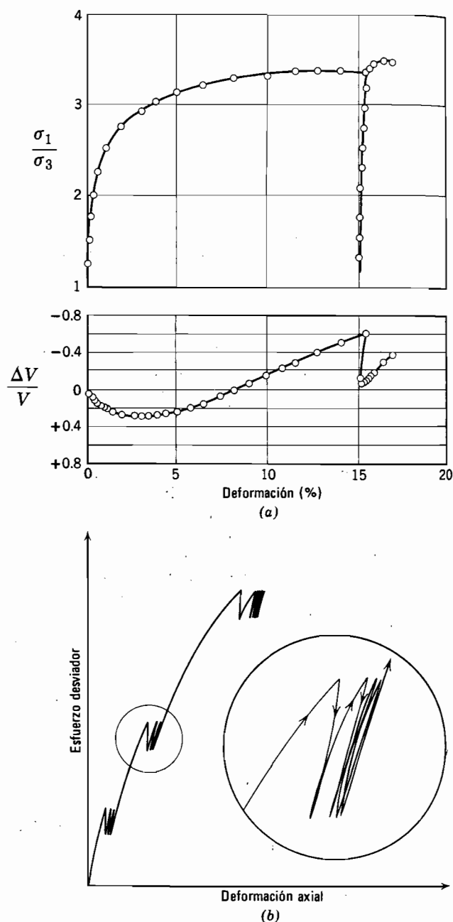
Fig. 10.19. Comportamiento en diversos ciclos de carga durante la prueba triaxial. a) Según Rowe, 1962. b) Según Shannon y Col., 1959.
