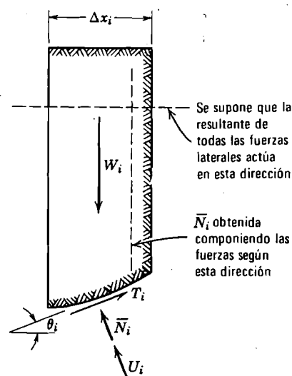
Fig. 24.13. Fuerzas consideradas en el método de Bishop simplificado.
