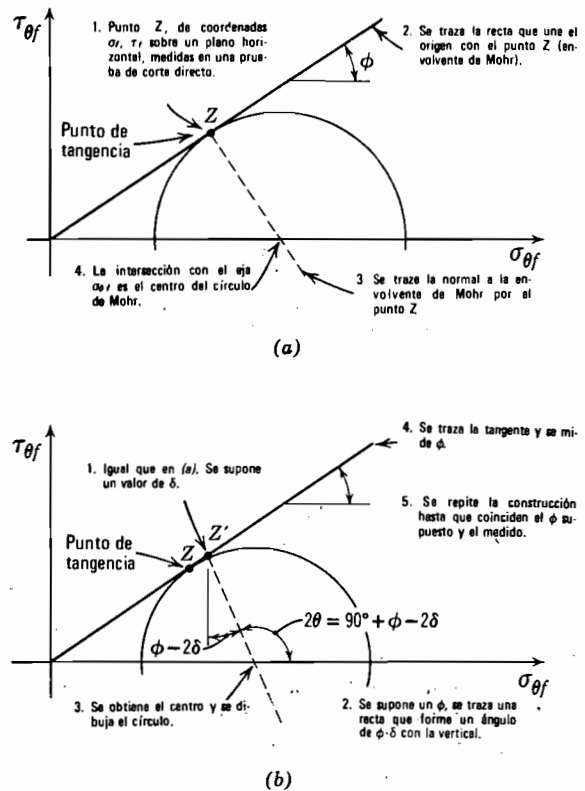
Fig. 11.7. Métodos para calcular el ángulo de fricción a partir de la prueba de corte directo. a) Suponiendo que el plano horizontal es el de falla teórico. b) Suponiendo que el plano horizontal es el de falla observado.
