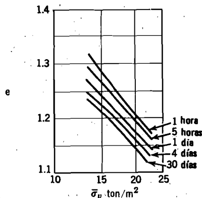
Fig. 27.15. Curvas e - \log \sigma_v en función de la duración de la consolidación secundaria. (Según Bjerrum, 1967).
