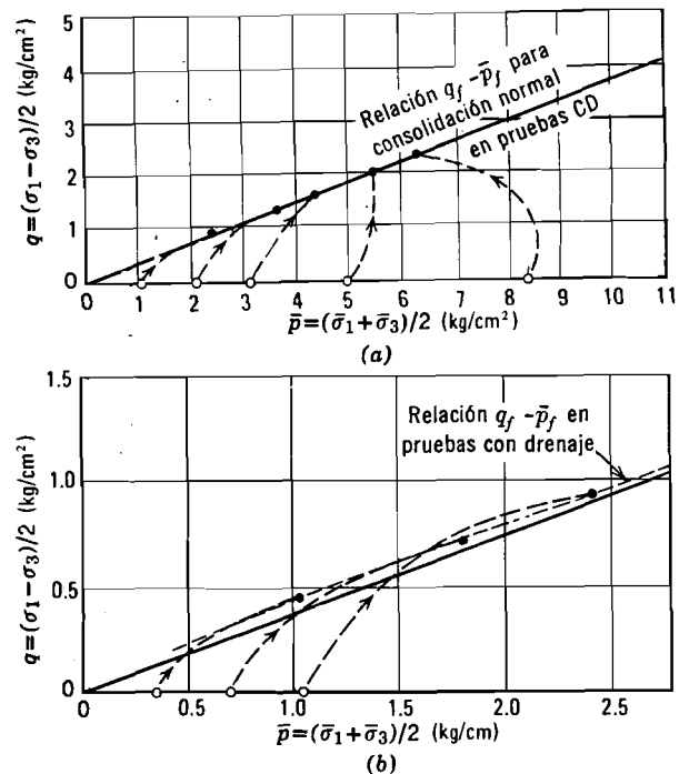
Fig. 28.8. Trayectorias de esfuerzos efectivos en pruebas CSD de arcilla de Weald sobreconsolidada. \bar{P}_m = 8.40 \text{ kg/cm}^2 .
