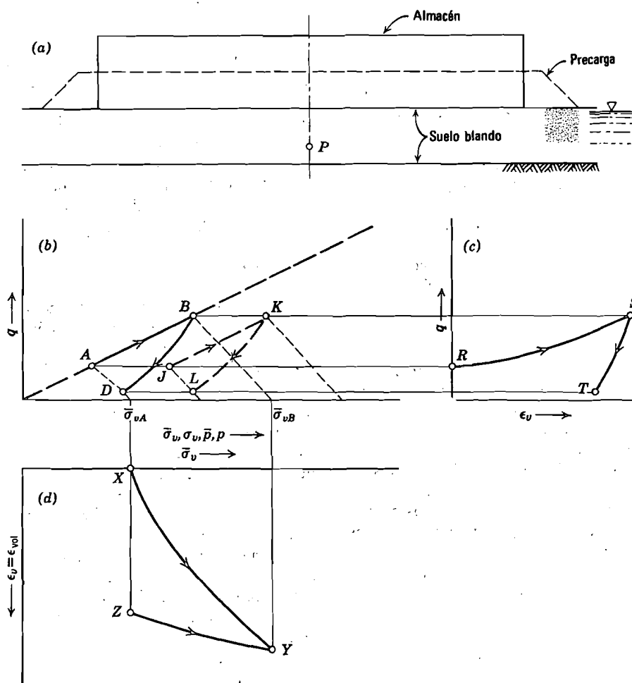
Fig. 34.11. . Esfuerzos y deformaciones en un terreno cargado previamente.
