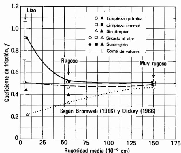
Fig. 6.8. Fricción del cuarzo [según Bromwell (1966) y Dickey (1966)].
