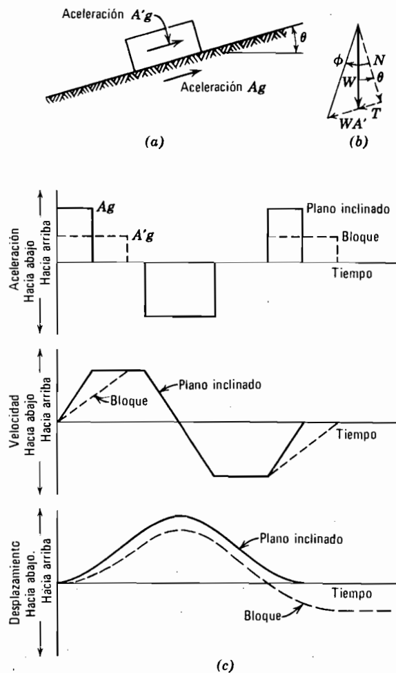
Fig. 15.17. Movimiento relativo entre un bloque y un plano inclinado bajo una sollicitación dinámica.
