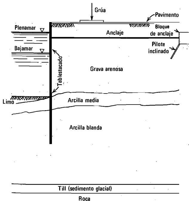
Fig. 1.15. Tablestacado anclado.
