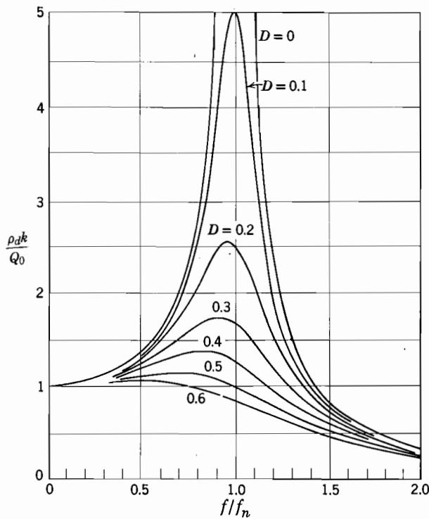
Fig. 15.2. Curvas de respuesta de un sistema masa-muelle-amortiguador.
