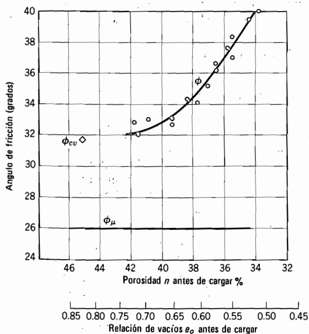
Fig. 11.8. Relación entre el ángulo de fricción y la porosidad inicial en arena fina a media (Según Rowe, 1962).
