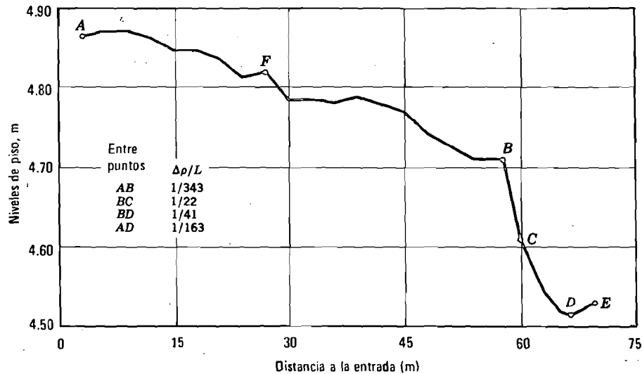
Fig. 25.5. Perfil del piso del corredor de la primera planta de un edificio de estructura metálica de tres plantas.
