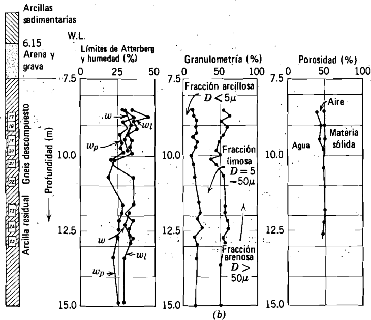
Fig. 7.16. Arcilla residual brasileña. a) Arcilla porosa residual (Campinas) procedente de la descomposición de una arenisca arcillosa. Variación de la consistencia, granulometría y porosidad con la profundidad. b) Arcilla residual (Belo Horizonte) procedente de la descomposición de un gneis. Variación de la consistencia, granulometría y porosidad con la profundidad. c) Presiones virtuales de preconsolidación en función de la profundidad de las muestras. (Según Vargas, 1953).
