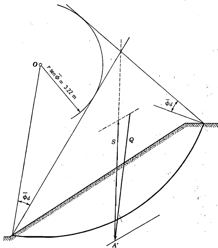
Fig. E24.3-6. Solución correspondiente al límite superior de estabilidad. Se supone \phi_d = 21^\circ , F_\phi = 1.63 , R_c/F = 3.15 t, F_c = 5/3.15 = 1.59 . Haciendo más tanteos se obtiene F = 1.61 .
