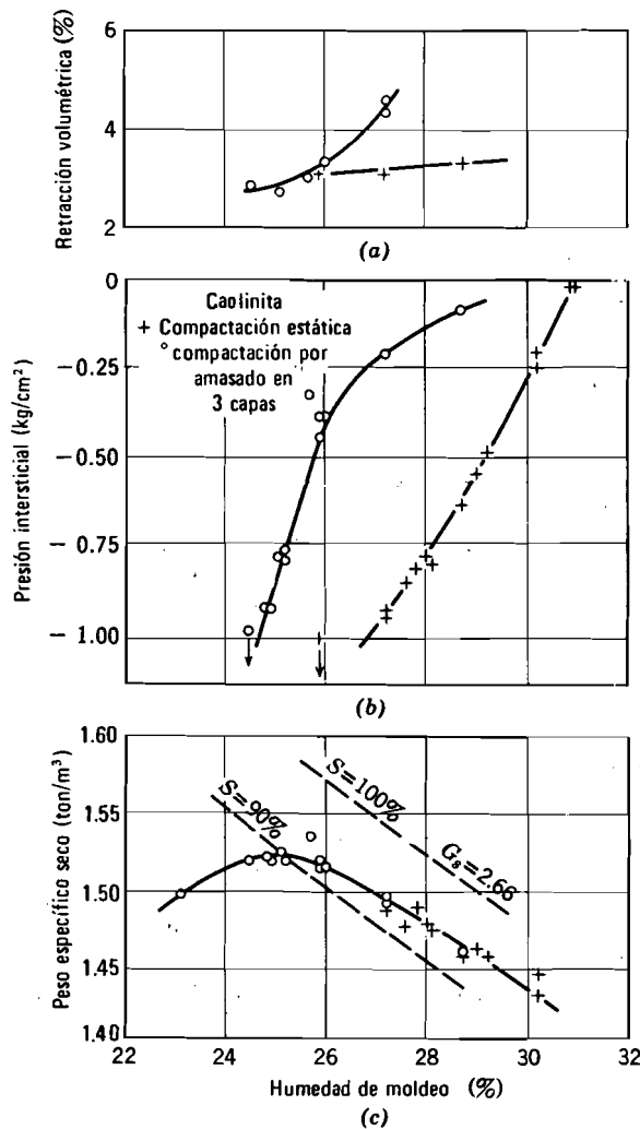
Fig. 34.7. Presiones intersticiales en caolinita compactada. (Según Lambe, 1961).
