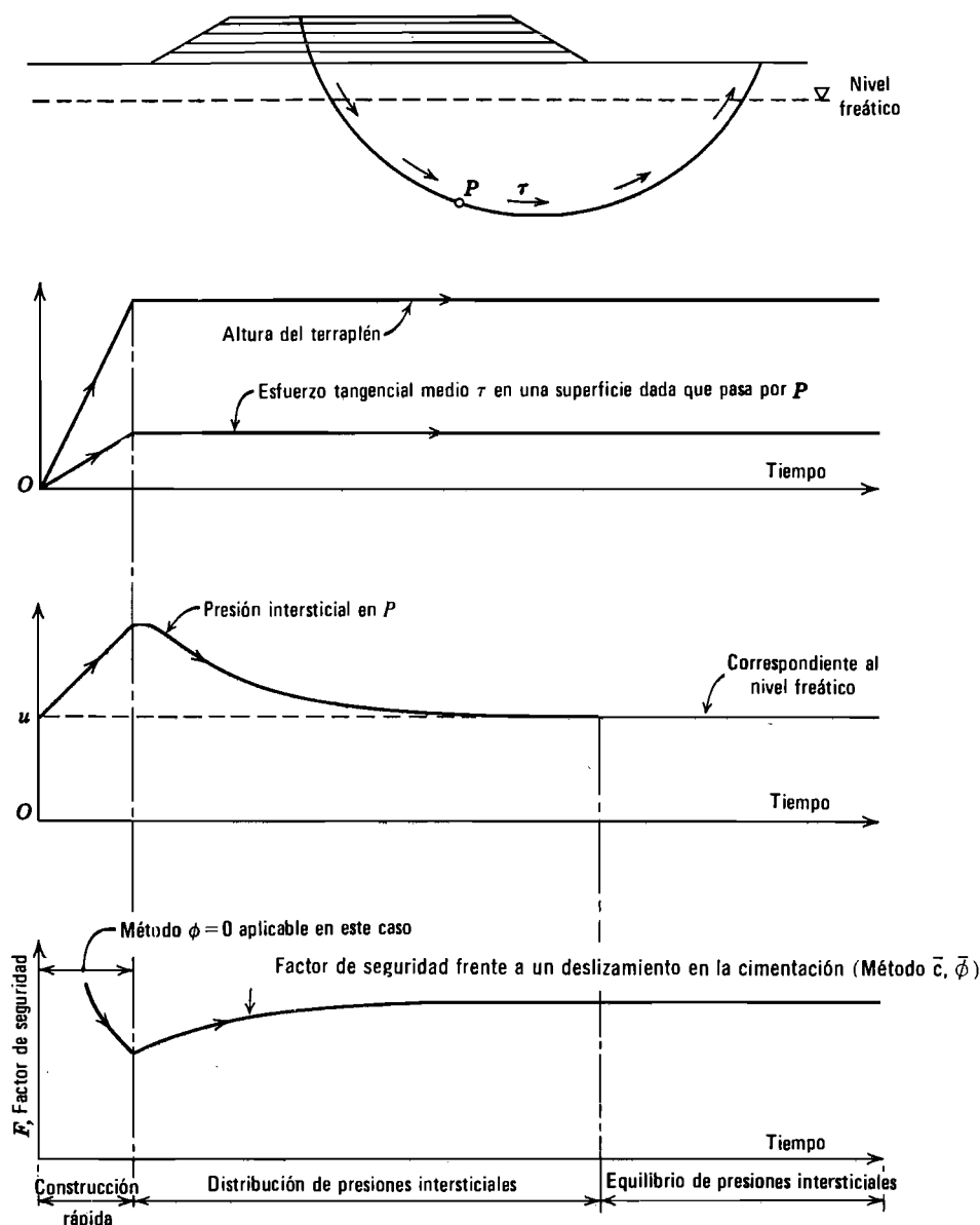
Fig. 31.5. Variación de los esfuerzos tangenciales, presiones intersticiales y factor de seguridad durante y después de la construcción de un terraplén (Según Bishop y Bjerrum, 1960).
