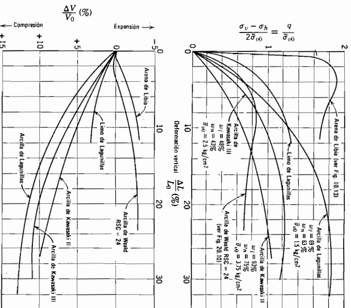
Fig. 22.3. Resultados de pruebas triaxiales con drenaje (presión horizontal constante).
