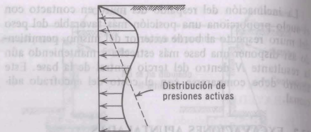
Fig. 13.26. Distribución típica de presiones sobre una entibación.
