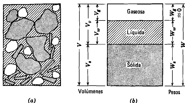
Fig. 3.1. Relaciones entre las fases de un suelo. a) Elemento de suelo natural. b) División de un elemento en fases.
