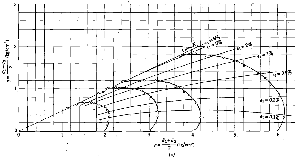
Fig. 30.3. Líneas de igual deformación de tres arcillas normalmente consolidadas. (a) Arcilla de Amuay. (b) Arcilla de Lagunillas. (c) Arcilla azul de Boston remoldada. (Según Lambe, 1964).
