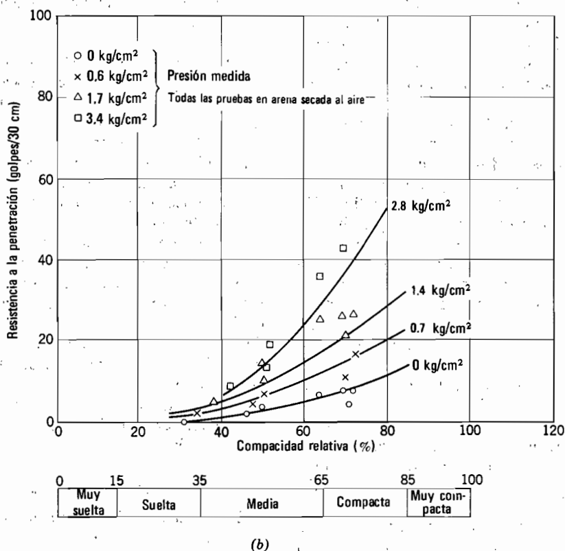
Fig. 7.5. Resultados de pruebas de penetración estándar. a) Arena gruesa. b) Arena fina. (De Gibbs y Holtz, 1957).
