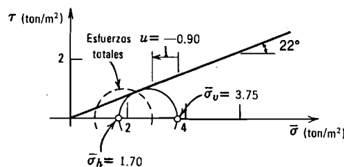
Fig. E23.12-3. Estado de esfuerzos a media altura.
