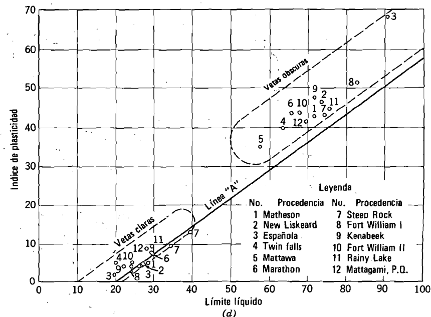
Fig. 7.12. Arcillas canadienses finamente estratificadas ( varved clays ). a) Variación de la humedad en una muestra de arcilla estratificada (según De Lory 1960). b) Humedades, límites y fracciones arcillosas en una muestra de arcilla estratificada (según De Lory, 1960). c) Muestras de arcillas estratificadas. d) Situación de algunas arcillas estratificadas en la carta de plasticidad de Casagrande. (Según Milligan, Soderman y Rutka, 1962).
