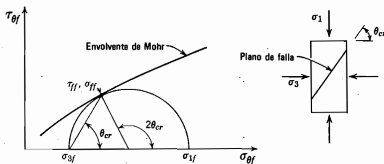
Fig. 11.2. Esfuerzos en la falla.
