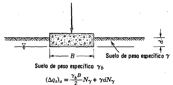
Fig. 25.6. Zapatas sobre arena saturada.
