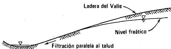
Fig. 24.4. Filtración en un talud natural.
