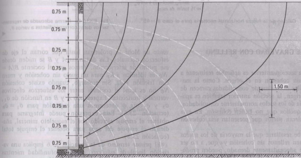
Fig. E23.6-2. Red de flujo en el caso de lluvia en régimen establecido.
