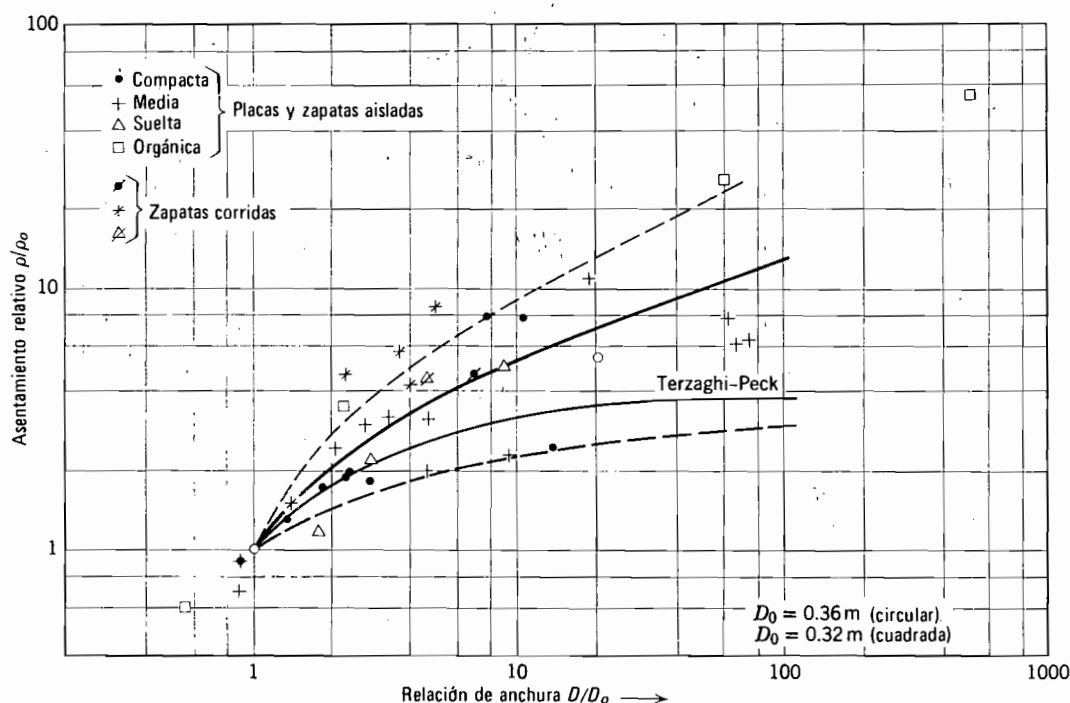
Fig. 14.26. Relación entre el asentamiento y las dimensiones de la superficie cargada según datos recogidos de casos reales (Según Bjerrum y Eggstad, 1963).
