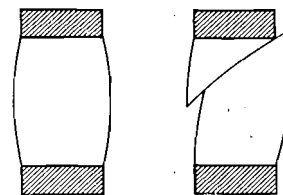
Fig. 9.6. Formas típicas de probetas rotas en una prueba triaxial con bases rígidas.
