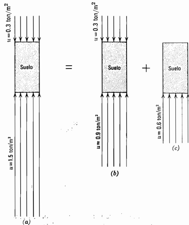
Fig. 17.14. Presiones de agua en un elemento de suelo. a) Presiones periféricas. b) Presiones hidrostáticas. c) Presión consumida en la filtración.
