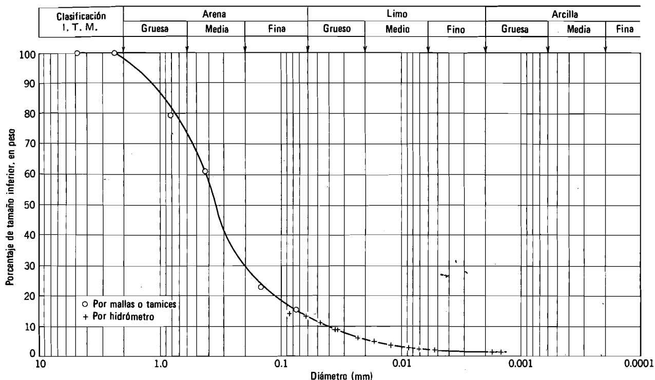
Fig. 3.3. Curva granulométrica de un suelo (Según Lambe, 1951).
