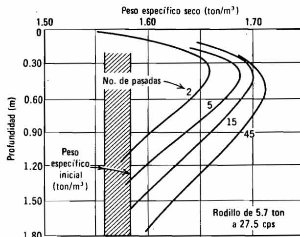
Fig. 15.13. Compactación producida por un rodillo vibratorio (Según D'Appolonia y Col., 1968).
