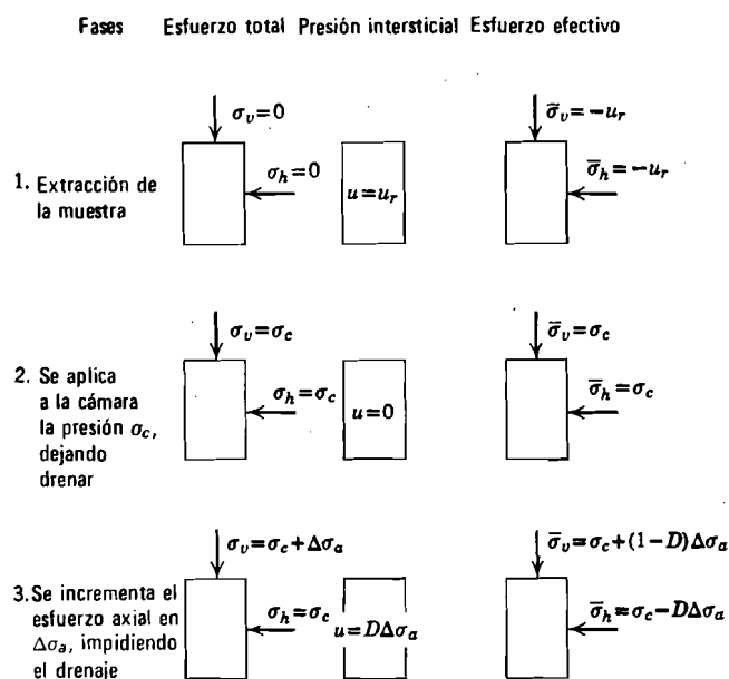
Fig. 28.5. Prueba triaxial con consolidación y sin drenaje (CSD).
