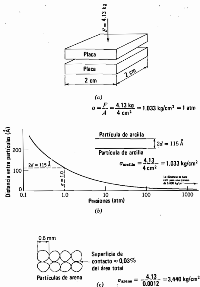
Fig. 5.16. Transmisión de presiones a través de un suelo.
