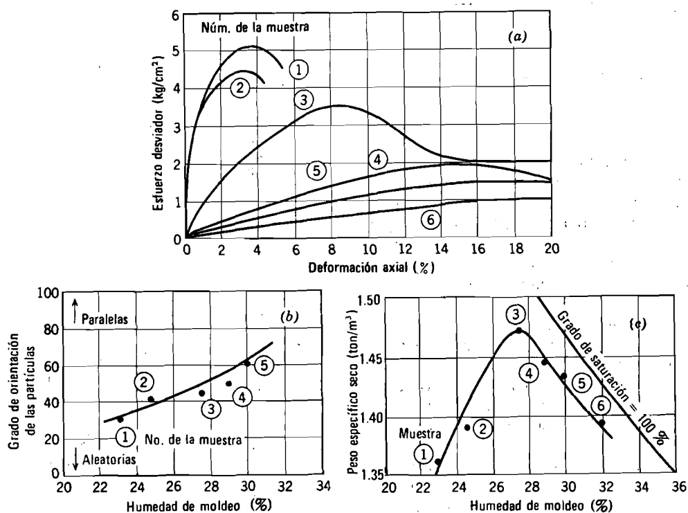
Fig. 34.10. Influencia de la humedad de moldeo sobre la estructura y la relación esfuerzo-deformación en muestras compactadas de caolinita. (a) Curvas esfuerzo-deformación de muestras compactadas. (b) Grado de orientación de las partículas en función de la humedad. (c) Peso específico en función de la humedad (Según Seed y Chan, 1959).
