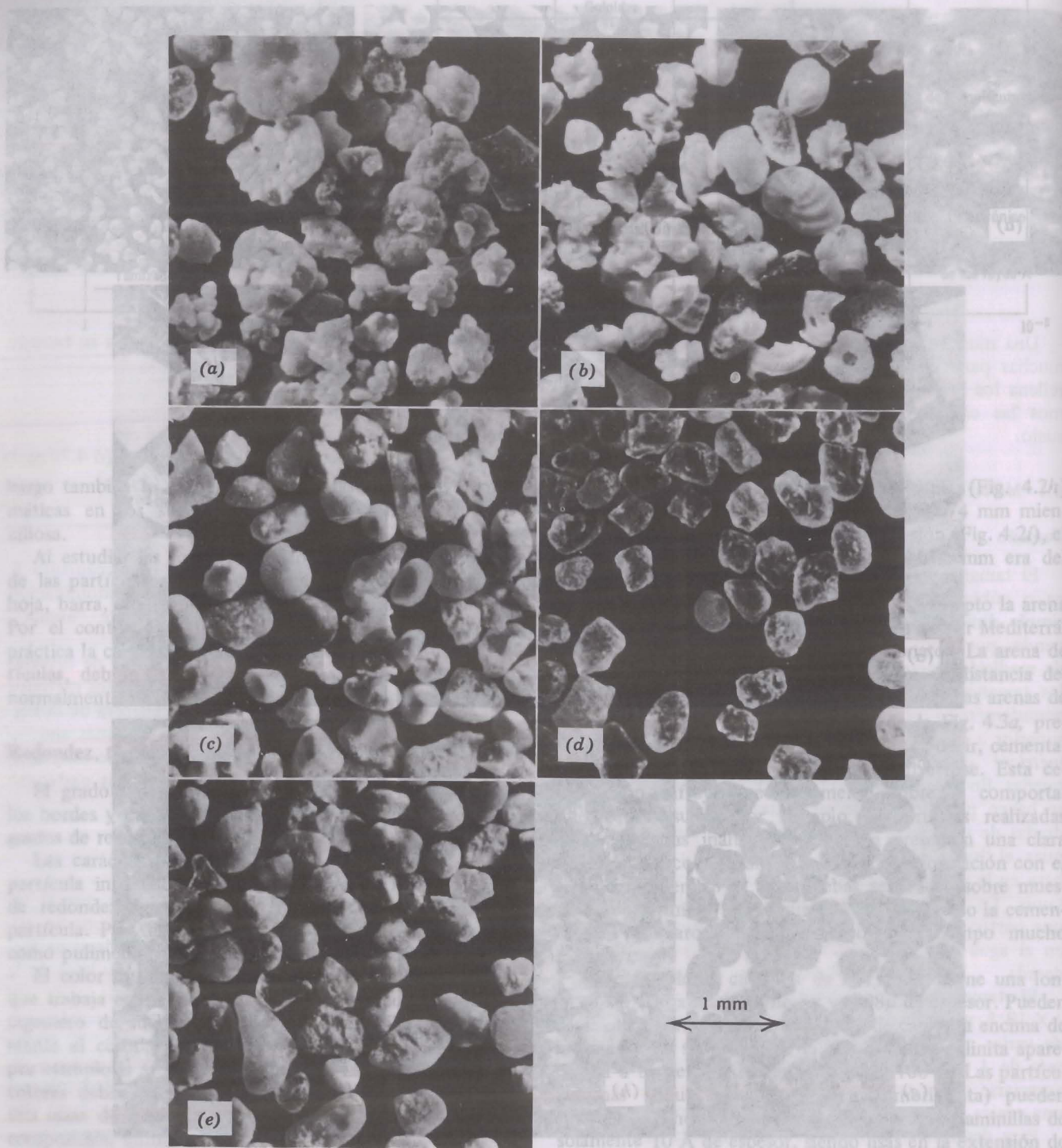
Fig. 4.3. Arenas de Libia (fracción de 0,15 a 0,25 mm). a) Terreno de una factoría, Brega. b) Fondo del puerto, Brega. c) Planta de gas natural. d) Brega Raguba. e) Recinto de depósitos de crudo, Brega. (Arenas facilitadas por ESSO, Libia; Fotos de R. T. Martín, M. I. T.).
