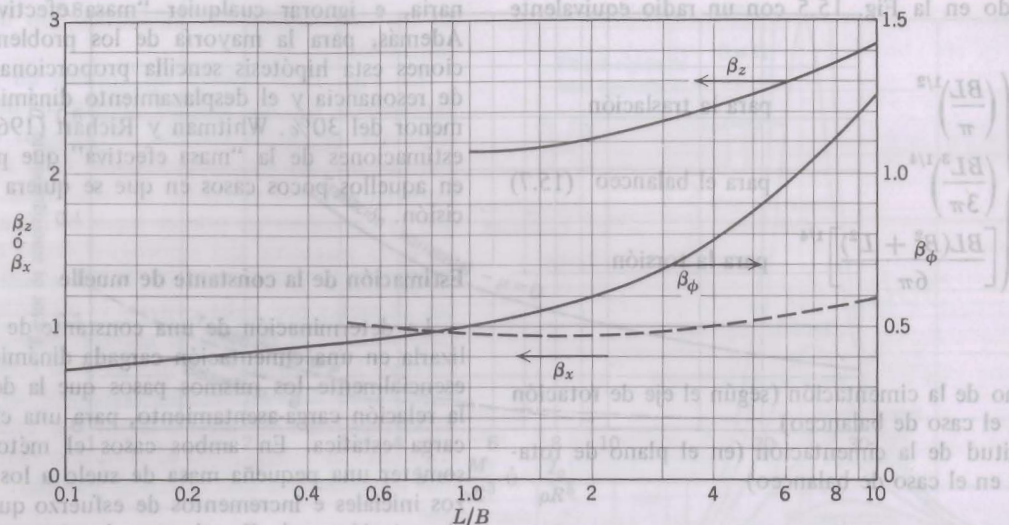
Fig. 15.6. Coeficientes de las constantes elásticas para cimentaciones rectangulares.
