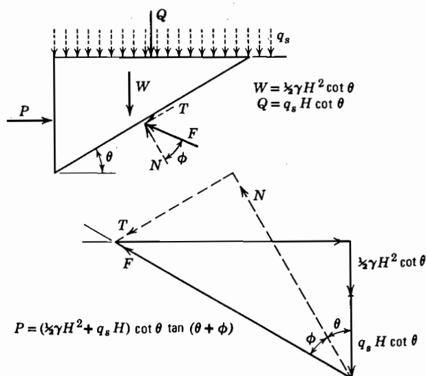
Fig. 13.14. Equilibrio de una cuña de suelo sobre un muro de retención en condiciones sencillas: empuje pasivo.
