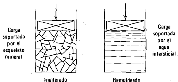
Fig. 29.17. Mecanismo de la transmisión de cargas durante el remoldeo.
