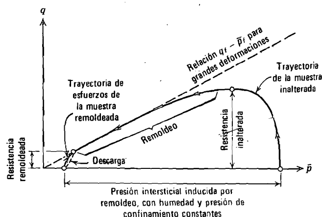
Fig. 29.16. Trayectorias de esfuerzos de suelos inalterados y remodelados.
