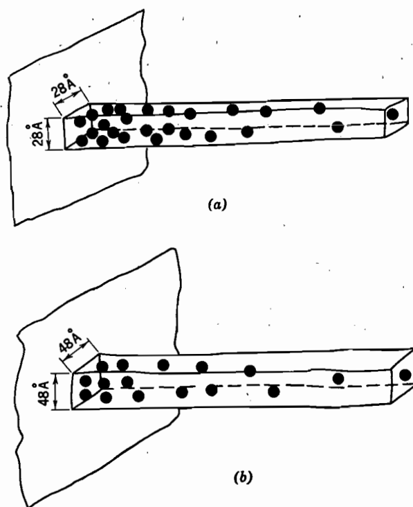
Fig. 5.10. Superficies de partículas con agua e iones. a) Caolinita sódica. b) Montmorilonita sódica.
