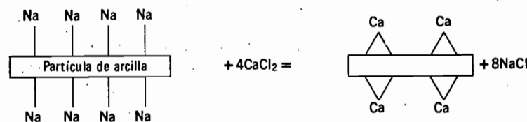
Fig. 5.12. Reacción de cambio iónico.
