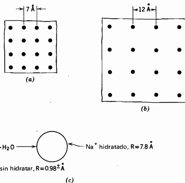
Fig. 5.7. Superficie de suelos con iones de cambio. a) Superficie de caolinita seca + iones de sodio. b) Superficie de montmorilonita seca + iones de sodio. c) Hidratación del ión de sodio.
