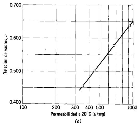
Fig. 19.9. Resultados de pruebas de permeabilidad con carga variable.
