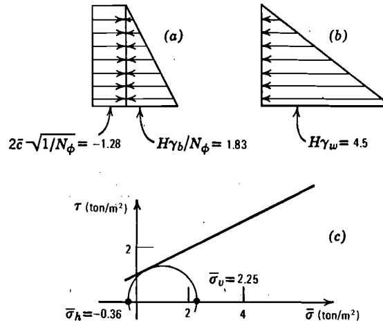
Fig. E23.10-2. a) Presiones sobre el muro producidas por el esqueleto mineral. (ton/m 2 ). b) Presiones producidas por el agua intersticial. c) Esfuerzos a media altura.
