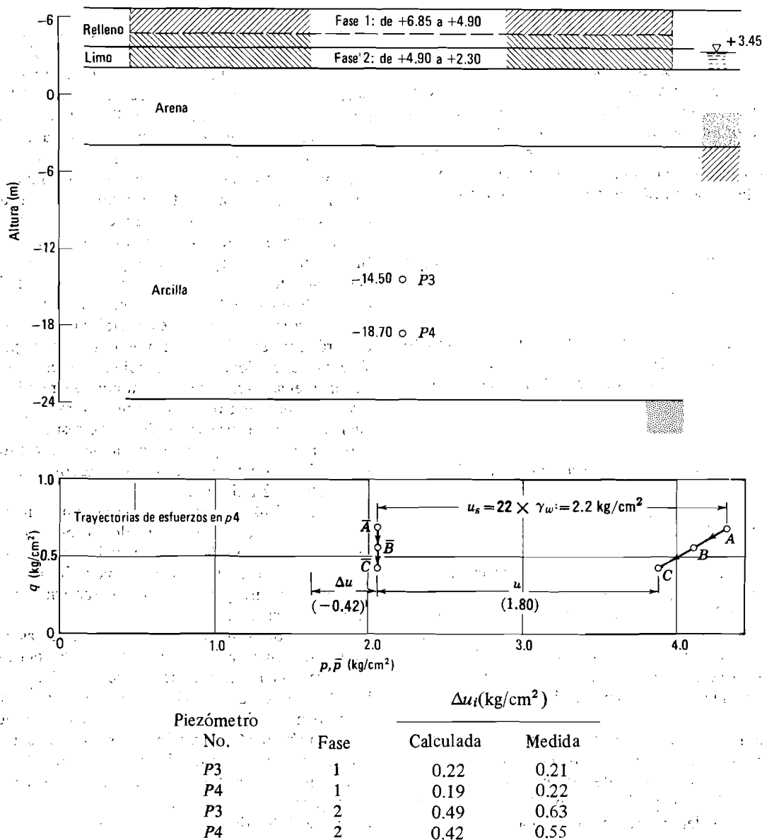
Fig. 26.15. Determinación de \Delta u_i al suprimir la carga.
