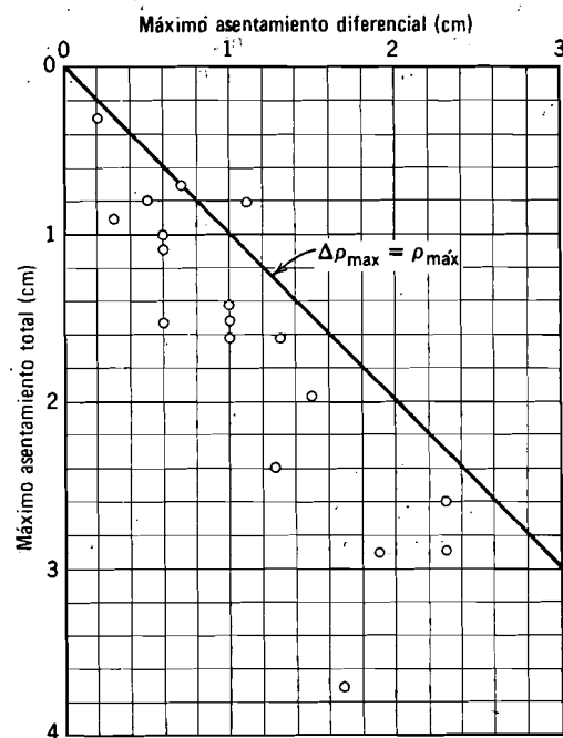
Fig. 25.2. Asentamiento de depósitos sobre arena de Libia.
