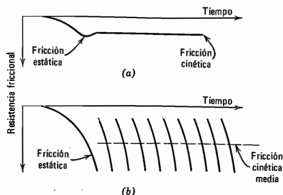
Fig. 6.6. Fricción estática y cinética. a) Deslizamiento suave. b) Deslizamiento intermitente. Nota: La célula de carga aplica el desplazamiento tangencial con cierta flexibilidad; las superficies en contacto sólo se desplazan a velocidad constante cuando deslizan suavemente.
