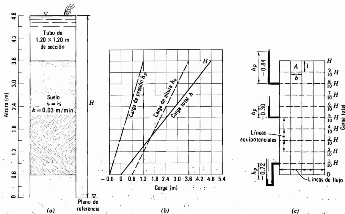
Fig. 18.1. Flujo unidimensional.
