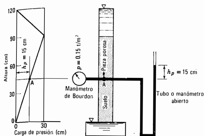
Fig. 17.5. Piezómetro de corriente.
