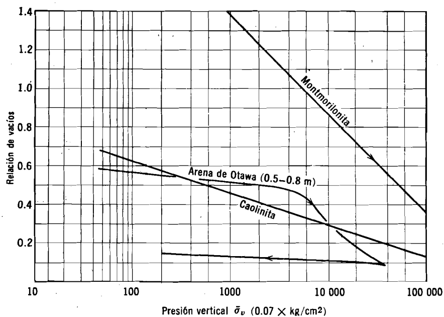
Fig. 20.4. Resultados de pruebas edométricas (Según Roberts, 1964).
