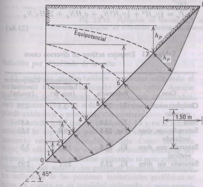
Fig. E23.6-3. Presiones intersticiales para \theta = 45^\circ
