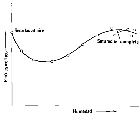
Fig. 34.5. Curva típica de compactación de arenas y gravas arenosas sin cohesión. (Según Foster, 1962).
