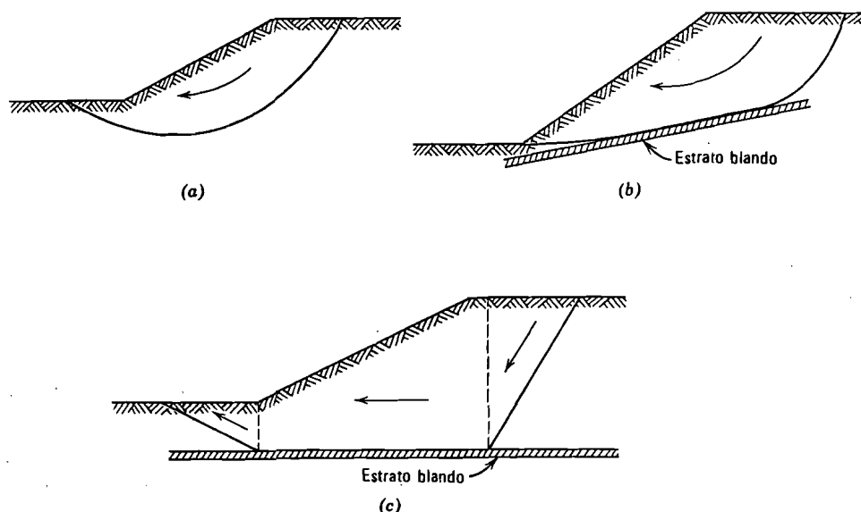
Fig. 24.8. Tipos de superficies de deslizamiento. a) Superficie circular. b) Superficie curva no circular. c) falla por deslizamiento de bloques.
