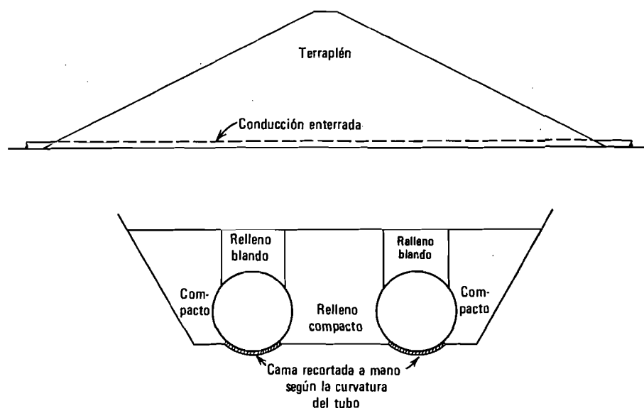
Fig. 1.16. Tuberías enterradas.
