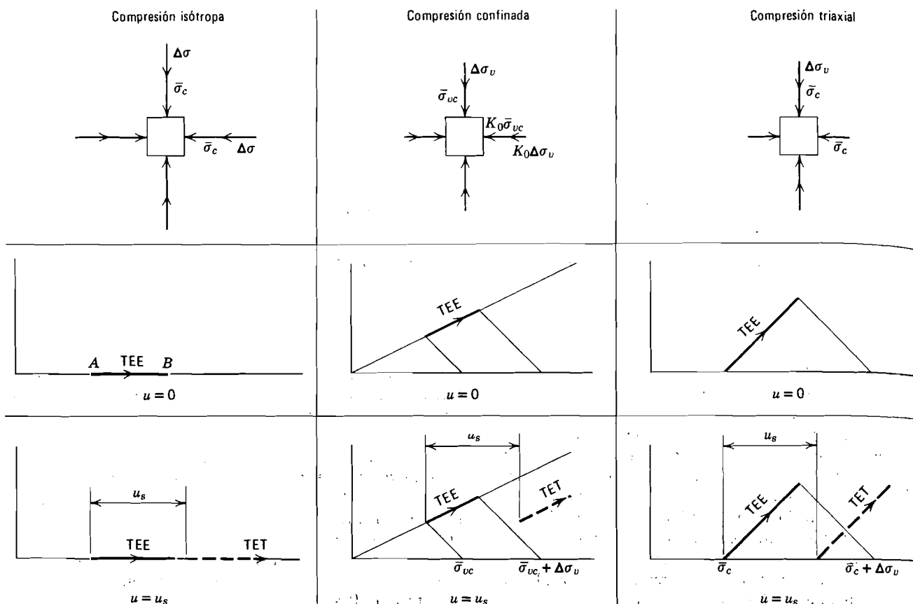
Fig. 20.1. Trayectorias de esfuerzos en pruebas de compresión.
