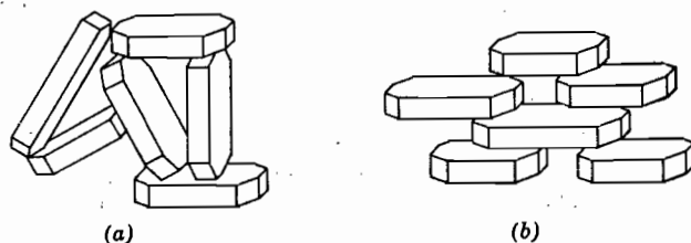
Fig. 7.1. Tipos de estructuras de un suelo. a) Floculada ; b) Dispersa .
