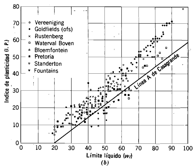
Fig. 7.15. Arcillas de África del Sur. a) Variación de las humedades medidas directamente bajo una losa impermeable. b) Resultados de pruebas de identificación de suelos sudafricanos en los que se han observado características expansivas. (Según Jennings, 1953).
