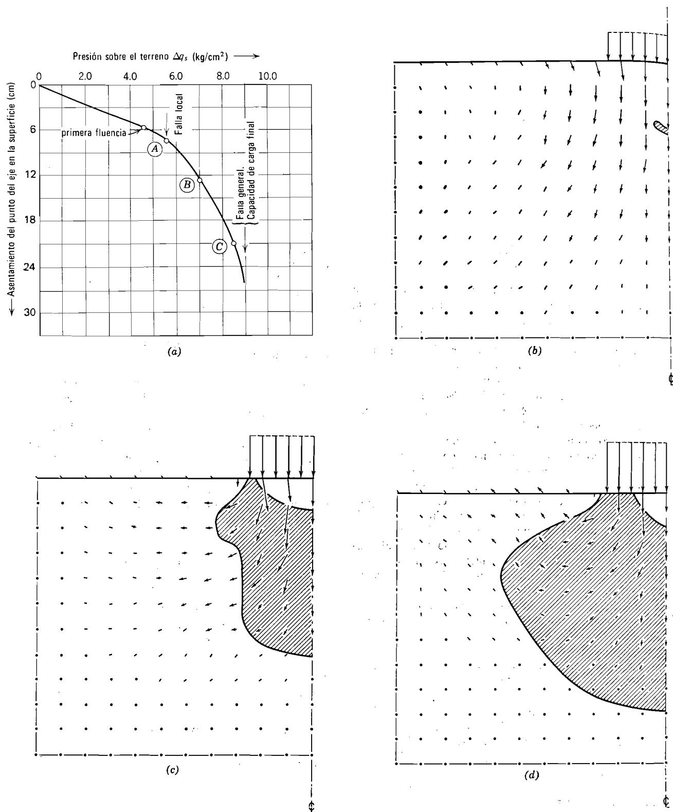
Fig. 14.2. a) Curva carga-asentamiento en el eje de un problema hipotético. b) Desplazamiento y primera fluencia bajo una carga de 4.40 kg/cm 2 . c) Extensión de la zona plastificada y campo de desplazamientos para una carga de 6.8 kg/cm 2 . d) Extensión de la zona plastificada y campo de desplazamientos para una carga de 8.30 kg/cm 2 .
