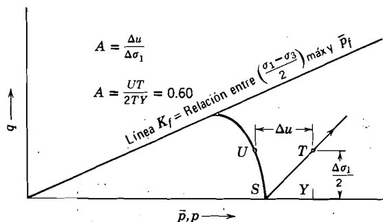
Fig. 26.10. Determinación de A en una prueba triaxial.
