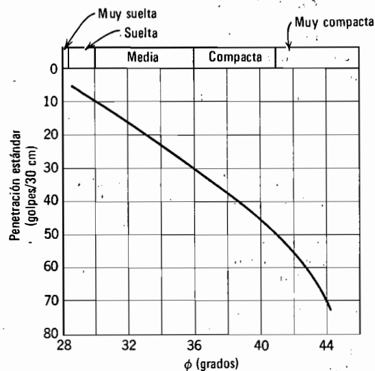
Fig. 11.14. Correlación entre el ángulo de fricción y la resistencia a la penetración (Según Peck, Hanson y Thornburn, 1953).
