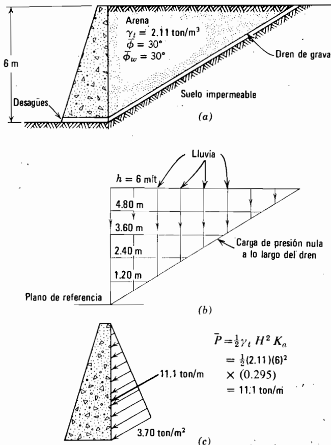
Fig. 23.8. Cálculo de un muro con dren inclinado en el relleno. a) Disposición del dren. b) Red de filtración del agua de lluvia en el relleno. c) Presiones producidas sobre el muro por el esqueleto mineral.
