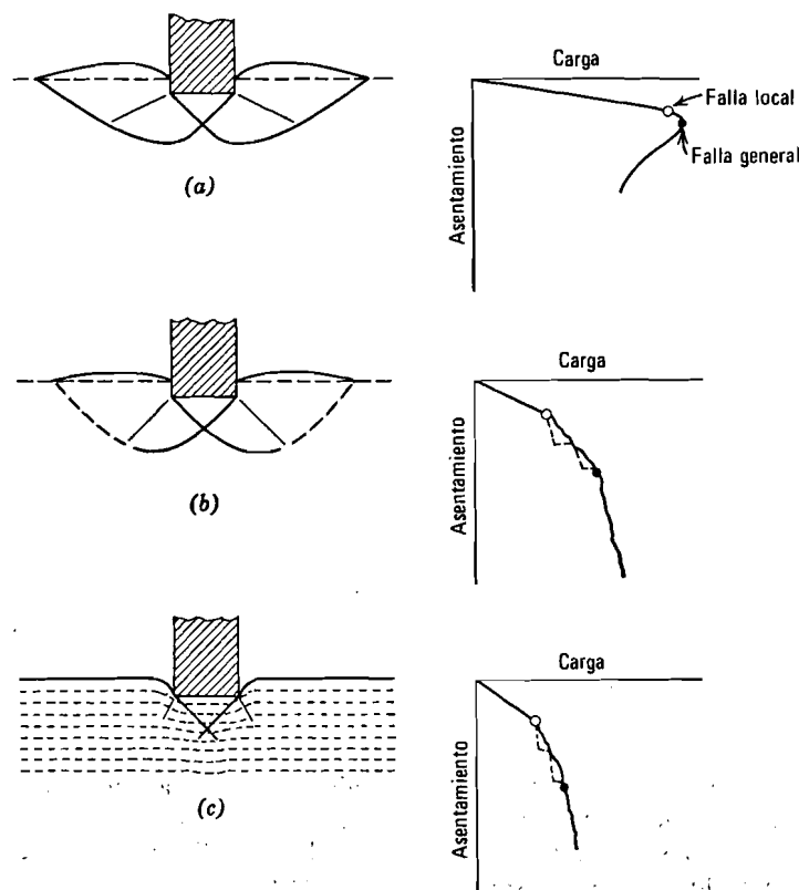
Fig. 14.4. Curvas carga-asentamiento y zonas de falla observadas en pruebas en modelo sobre arena. a) Arena compacta. b) Arena de compacidad media. c) Arena muy suelta, (Según Vesic, 1963).
