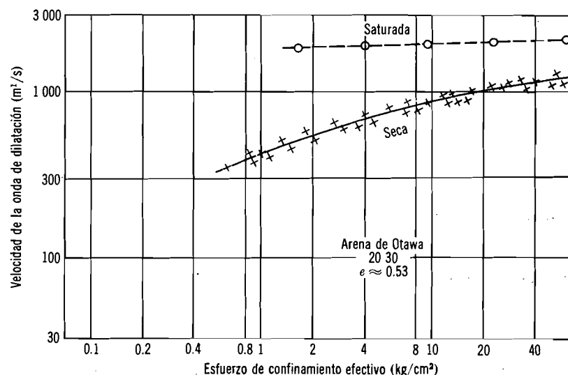
Fig. 30.1. Velocidades de dilatación medidas en arena seca y saturada (datos obtenidos por el Laboratorio Shell de Investigación y Desarrollo por técnicas de impulso).
