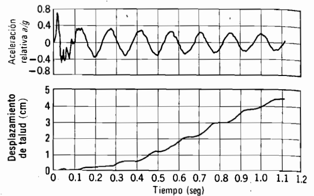
Fig. 15.18. Desplazamiento de un talud arenoso sometido a cargas dinámicas. a) Disposición esquemática de la capa de arena para la prueba de sacudidas. b) Aceleración y desplazamiento del talud bajo las sacudidas. Arena de Monterrey No. 20. Talud de 31^\circ . (Según Goodman y Seed, 1966).
