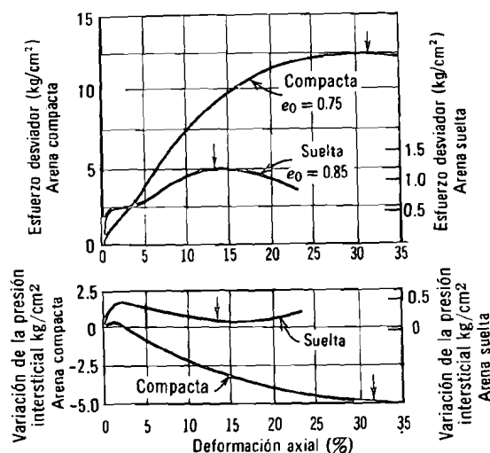
Fig. 29.1. Curvas esfuerzo-deformación en la prueba triaxial sin drenaje de una arena saturada (según Leonards, 1962).
