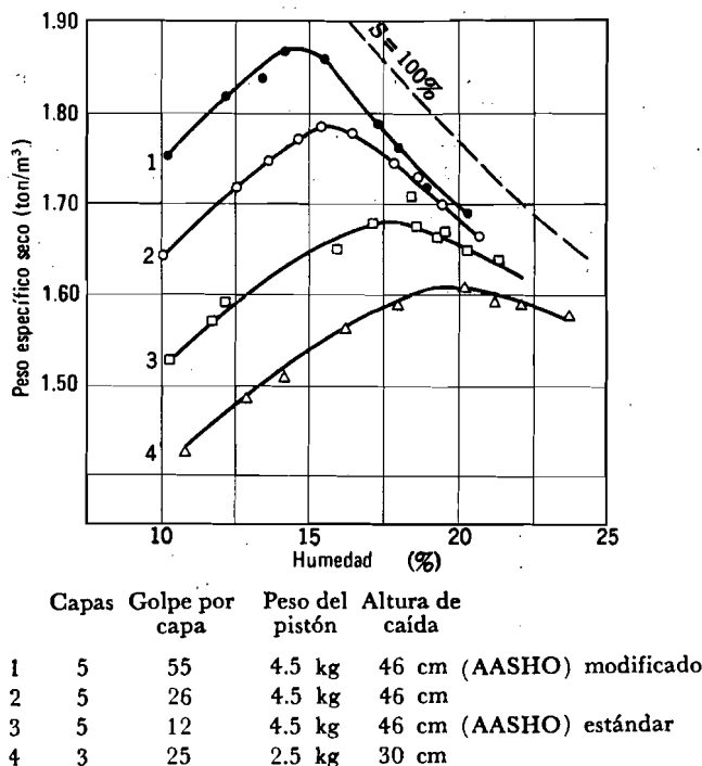
Fig. 34.2. Curvas de compactación dinámica para una arcilla limosa (Según Turnbull, 1950).
