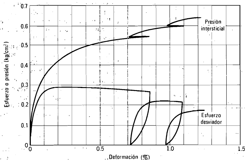
Fig. 29.8. Influencia de la repetición de cargas sobre la resistencia sin drenaje de arena saturada muy suelta. Muestra consolidada a 0.7 kg/cm²; Relación de vacíos = 0.834. (Según Healy, 1963).
