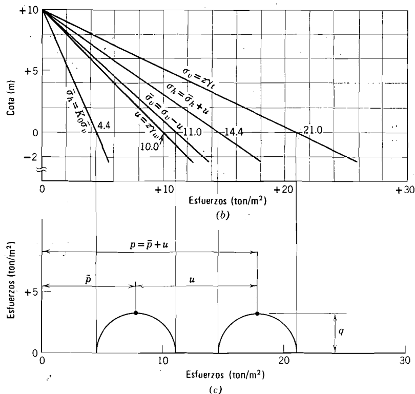
Fig. E16.1. Esfuerzos en el terreno. a) Perfil del terreno. b) Esfuerzos a diferentes profundidades. c) Esfuerzos en A.
