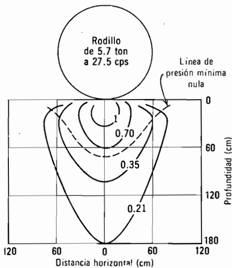
Fig. 15.14. Líneas de igual presión máxima vertical (dinámica) bajo un rodillo vibratorio, en \text{kg/cm}^2 (según D'Appolonia y Col., 1968).
