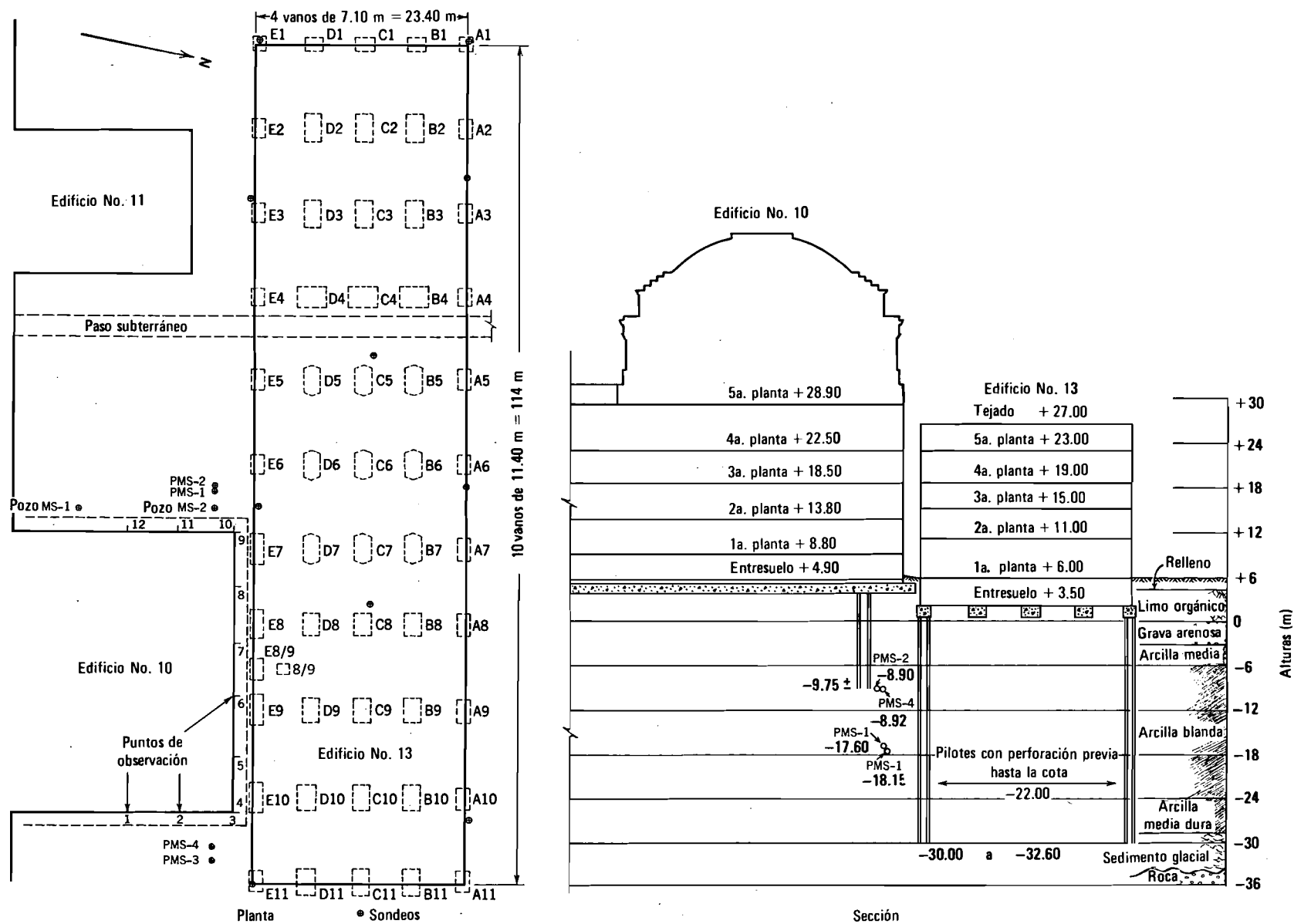
Fig. 33.10. Edificios 10 y 13 del M. I. T.
