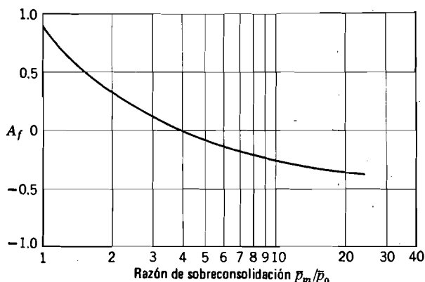
Fig. 28.9. Parámetro de presión intersticial A_f para la arcilla de Weald.
