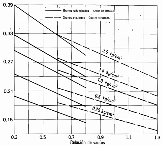
Fig. 12.10. Velocidades de ondas tangenciales en arenas cuarzosas (según Hardin y Richart, 1963).
