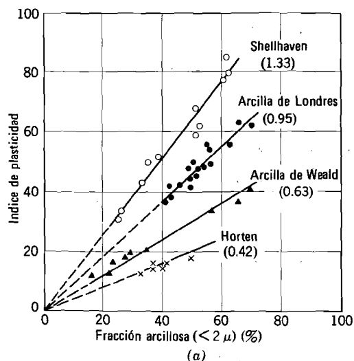
Fig. 3.5. "Relación entre el índice de plasticidad y la fracción arcillosa. Los números entre paréntesis señalan la "actividad" de las arcillas. (Según Skempton, 1933).
