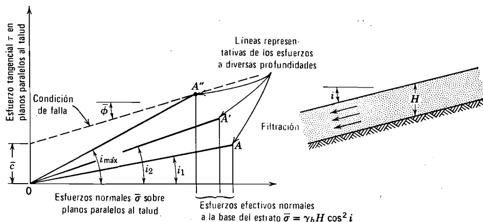
Fig. 24.6. Desarrollo de condiciones de falla al variar gradualmente la inclinación de un estrato.
