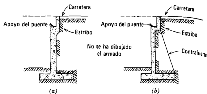
Fig. 13.23. Muros de contención, en ménsula y con contrafuertes. a) En ménsula. b) De contrafuertes. (Según Huntington, 1957).
