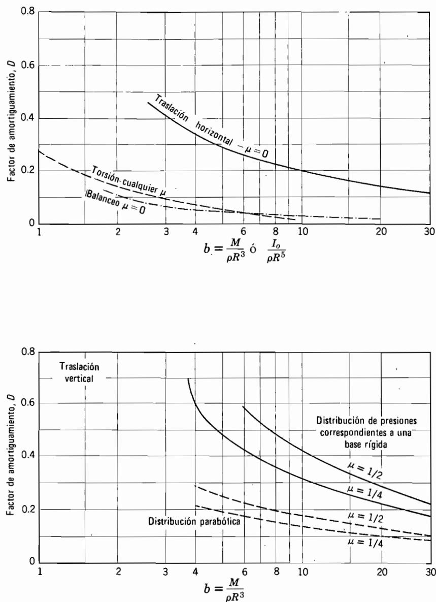
Fig. 15.5. Factor de amortiguamiento equivalente de cimentaciones circulares.
