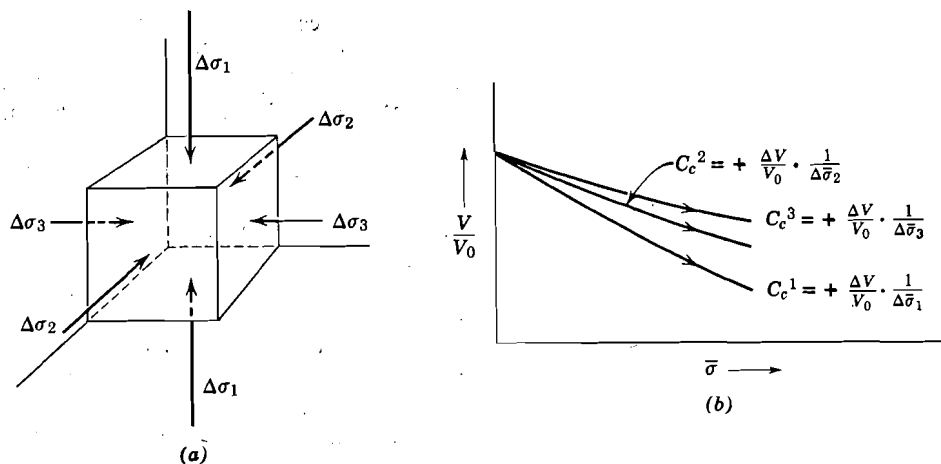
Fig. 26.6. Carga tridimensional. (a) Carga. (b) Deformación.
