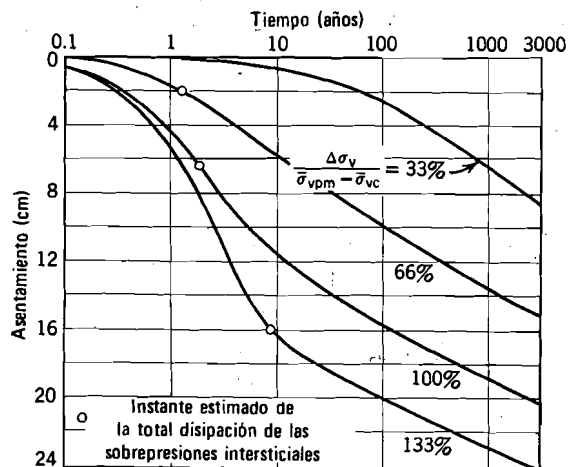
Fig. 27.18. Curvas de consolidación para diferentes incrementos de presiones \bar{\sigma}_{vpm} es una presión de preconsolidación virtual. (Según Bjerrum, 1967).
