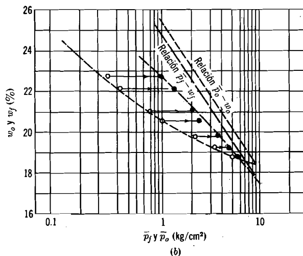
Fig. 28.11. Relaciones esfuerzo-volumen para una arcilla de Weald sobreconsolidada. \bar{p}_m = 8.40 \text{ kg/cm}^2 .
