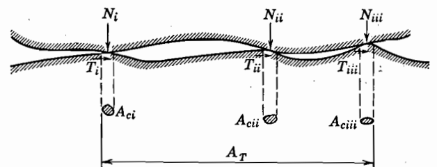
Fig. 6.2. Interpretación microscópica de la resistencia por fricción.
