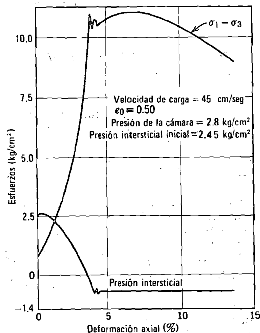
Fig. 29.3. Cavitación en la prueba triaxial sin drenaje de una arena compacta (Según Whitman y Healy, 1962).
