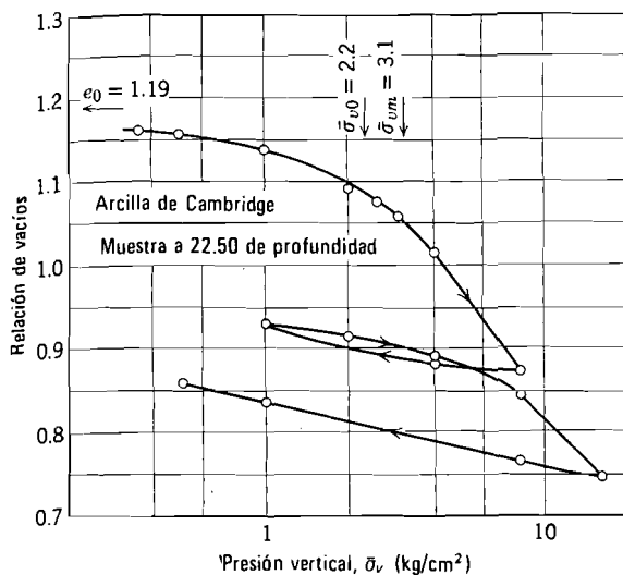
Fig. 20.5. Resultados de una prueba edométrica.
