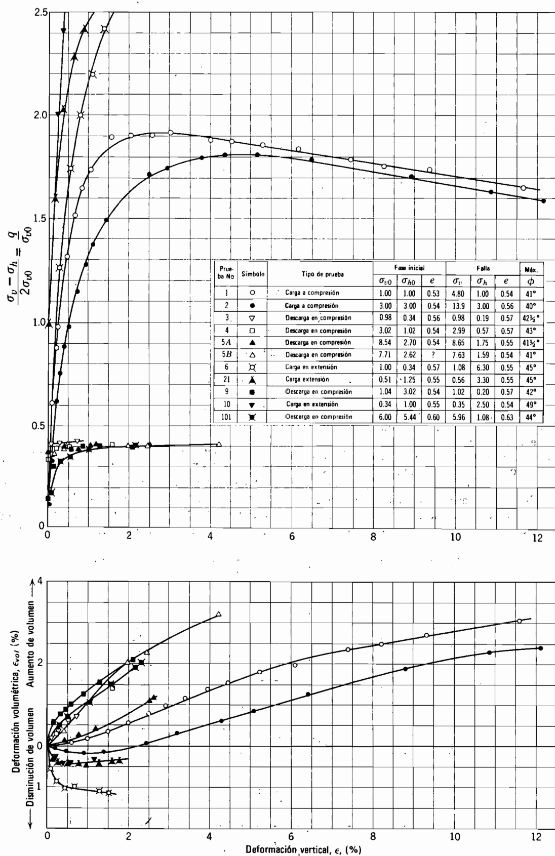
Fig. 10.22. Datos esfuerzo-deformación para diversos estados de carga.
