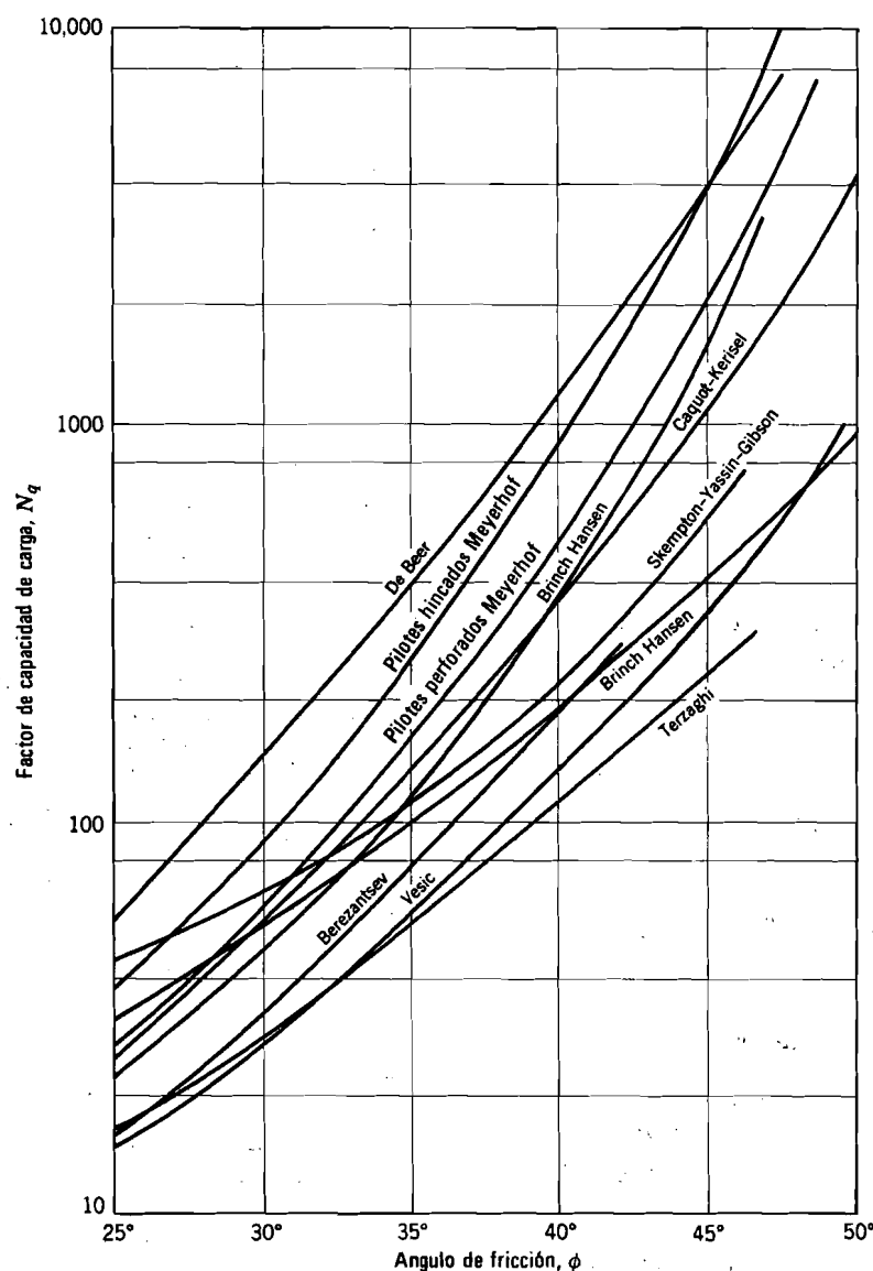
Fig. 33.4. Factores de capacidad de carga para cimentaciones profundas circulares. (Según Vesic, 1967).
