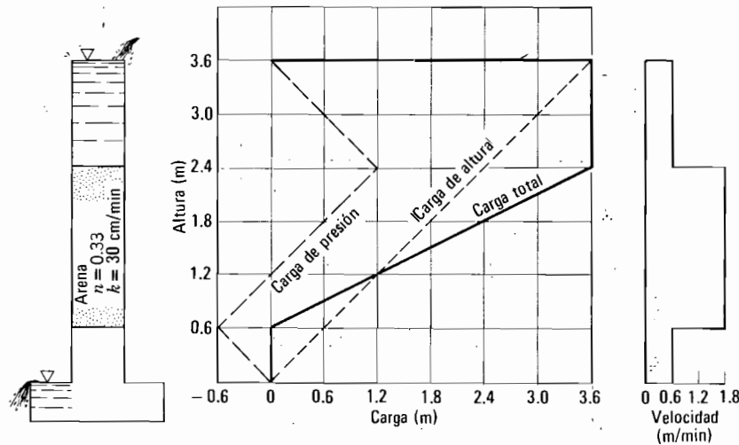
Fig. 17.8. Ejemplo de flujo descendente.
