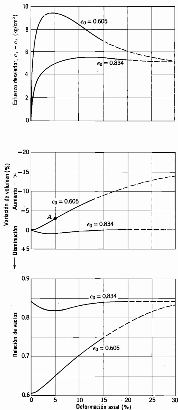
Fig. 10.18. Curvas esfuerzo-deformación para muestras sueltas y compactas de arena fina a media. \sigma_3 = 2.1 kg/cm 2 e_0 = 0.605 \approx 100\% D_r ; e_0 = 0.834 \approx 20\% D_r . Línea continua, datos reales; línea de trazos, extrapolaciones basadas en resultados de otras pruebas. (Según Taylor, 1948).
