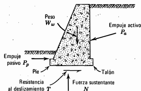
Fig. 13.2. Fuerzas actuantes sobre un muro de gravedad.
