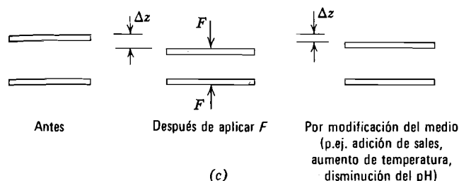
Fig. 20.2. Mecanismos de deformación. a) Deformación de partículas de mica. b) Reorientación de partículas. c) Reducción de la distancia entre partículas.
