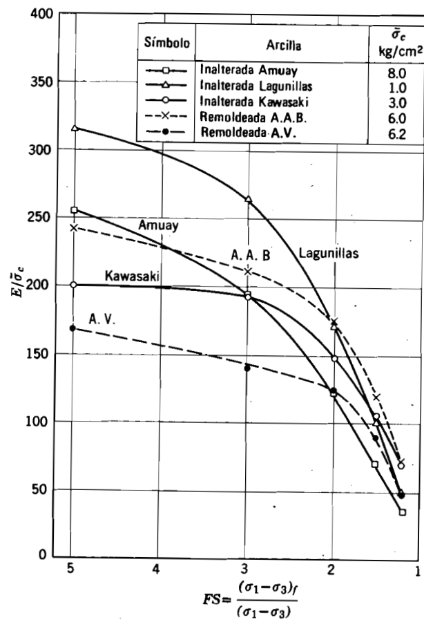
Fig. 30.5. Módulo sin drenaje de cinco arcillas normalmente consolidadas (Según Ladd, 1964).
