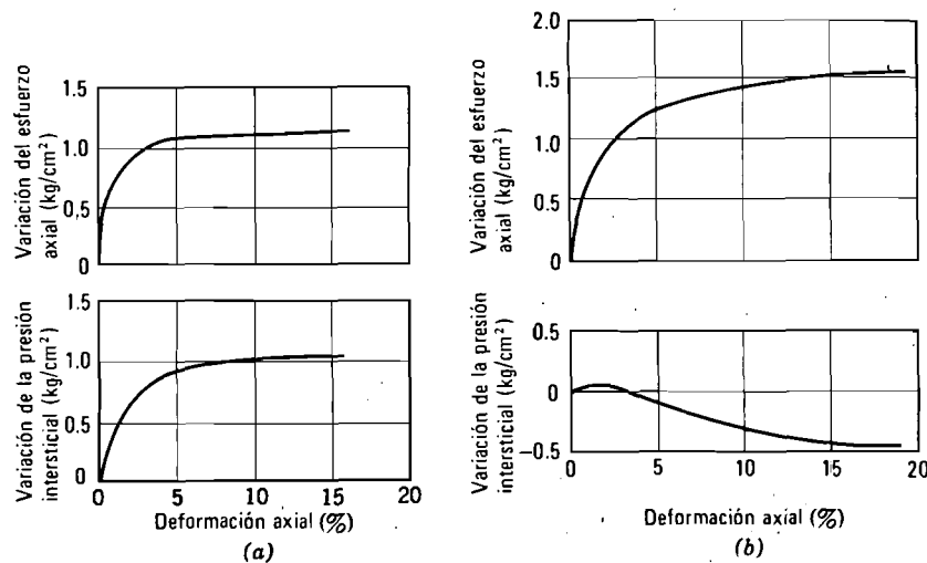
Fig. 28.6. Curvas típicas esfuerzo-deformación de pruebas CSD en arcilla de Weald (a) Muestras normalmente consolidadas a 2.1 \text{ Kg/cm}^2 . (b) P_m = 8.40 \text{ kg/cm}^2 P = 0.7 \text{ kg/cm}^2
