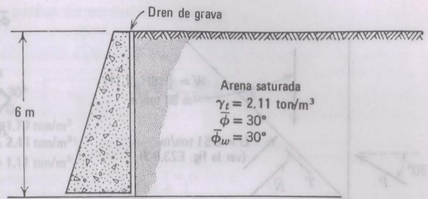
Fig. E23.6-1. Muro de retención con dren.
