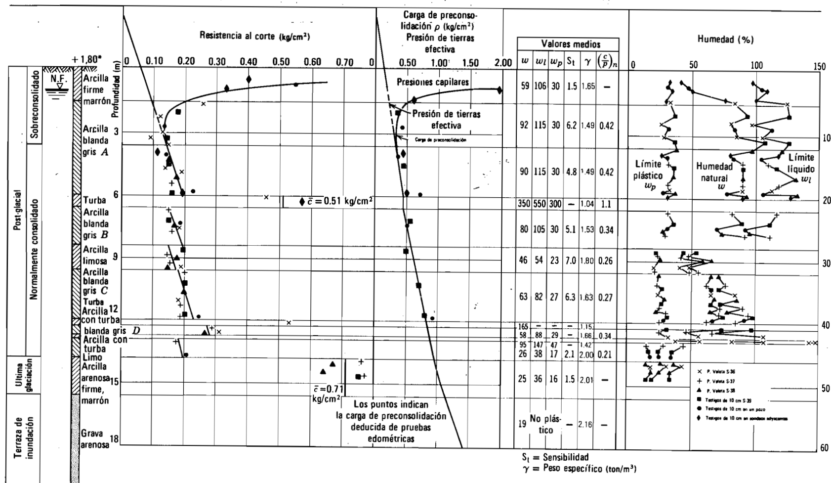
Fig. 7.10. Arcilla del estuario del Támesis (Según Skempton y Henkel, 1953).
