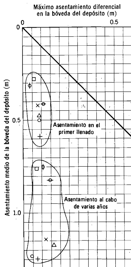
Fig. 25.4. Asentamiento de los depósitos de Kawasaki.
