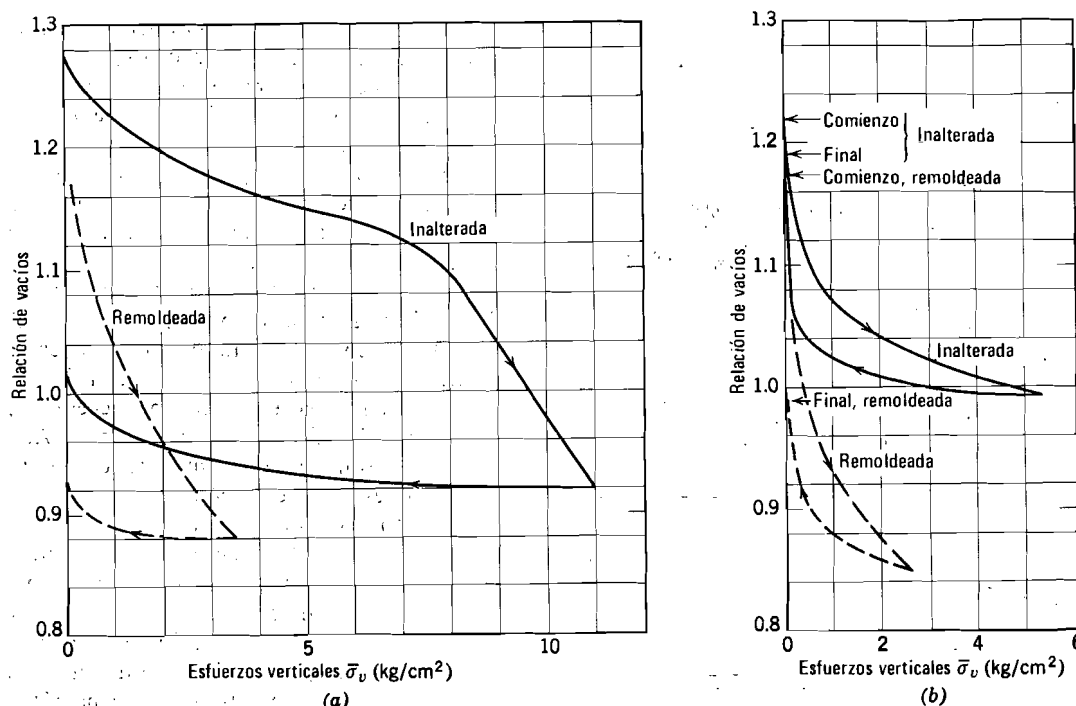
Fig. 20.9. Influencia de la perturbación sobre el comportamiento esfuerzo-deformación. (a) Arcilla de San Lorenzo. (b) Arcilla de Boston. (Datos de Casagrande, 1932).
