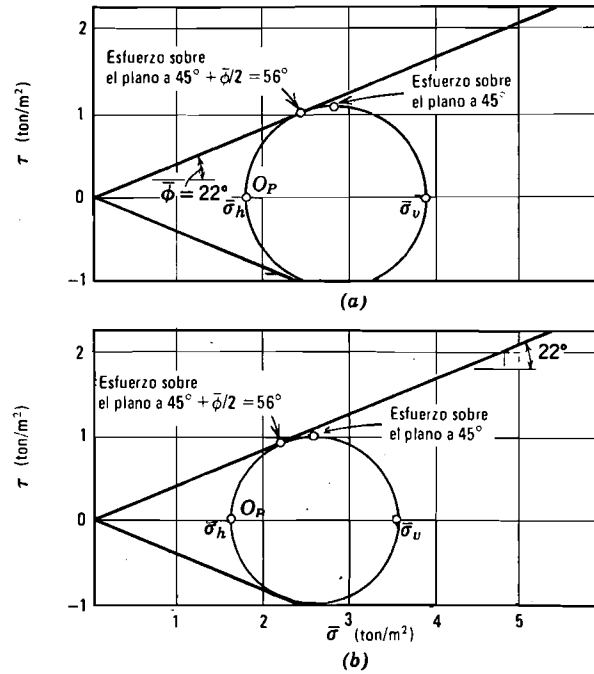
Fig. E31.5-1. (a) Al final de la construcción. (b) A largo plazo.
