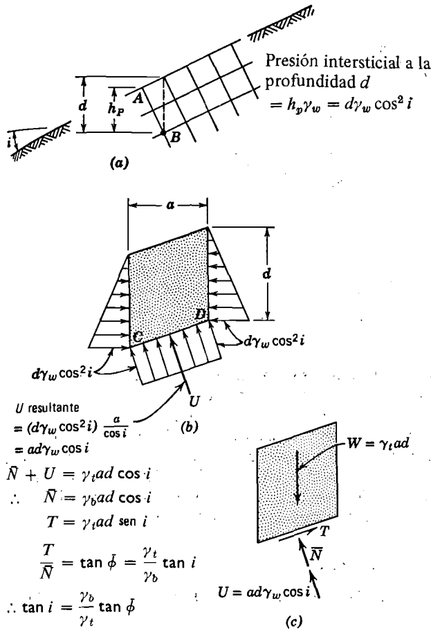
Fig. 24.3. Estudio de un talud infinito con filtración paralela al talud. (a) Red de flujo. (b) Presiones intersticiales periféricas. (c) Cálculo del equilibrio de fuerzas (momentos equilibrados por las fuerzas laterales).
