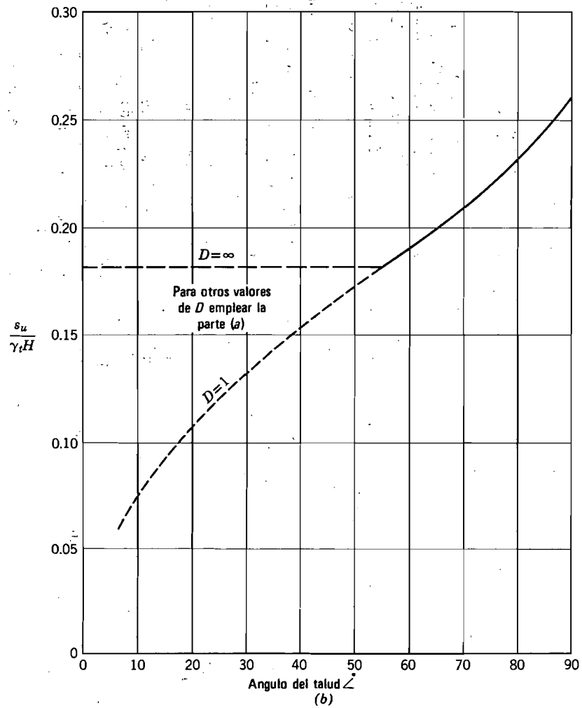
Fig. 31.1. Gráficas de estabilidad para \phi = 0 . (Taylor, 1948).
