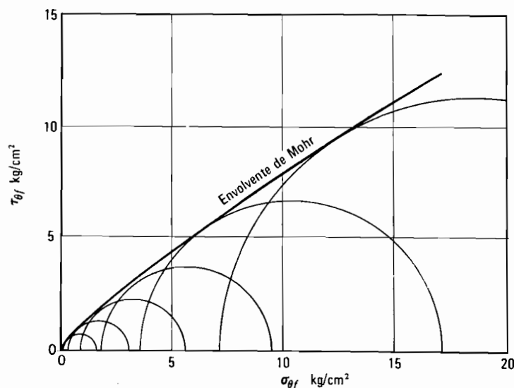
Fig. 11.1. Envolvente de Mohr de una mezcla de arena y grava (datos de Hóltz y Gibbs, 1956).
