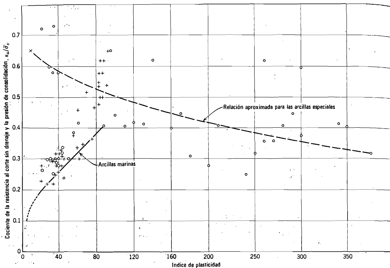
Fig. 29.19. Variación de la relación s_u / \bar{\sigma}_v con el índice de plasticidad (según Osterman, 1959).
