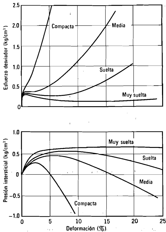
Fig. 29.6. Curvas esfuerzo-deformación en pruebas triaxiales sin drenaje en arenas saturadas con cuatro compacidades. Muestras consolidadas a 0.7 \text{ kg/cm}^2 . (Según Healy, 1963).
