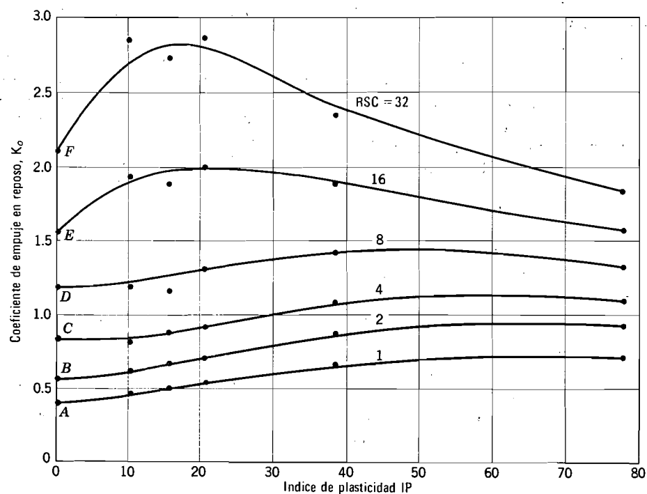
Fig. 20.8. Relación entre K_0 , la razón de sobreconsolidación y el índice de plasticidad. Los puntos A a F se han interpolado a partir de los datos de Hendron, RSC = razón de sobreconsolidación (Según Brooker e Ireland, 1965).
