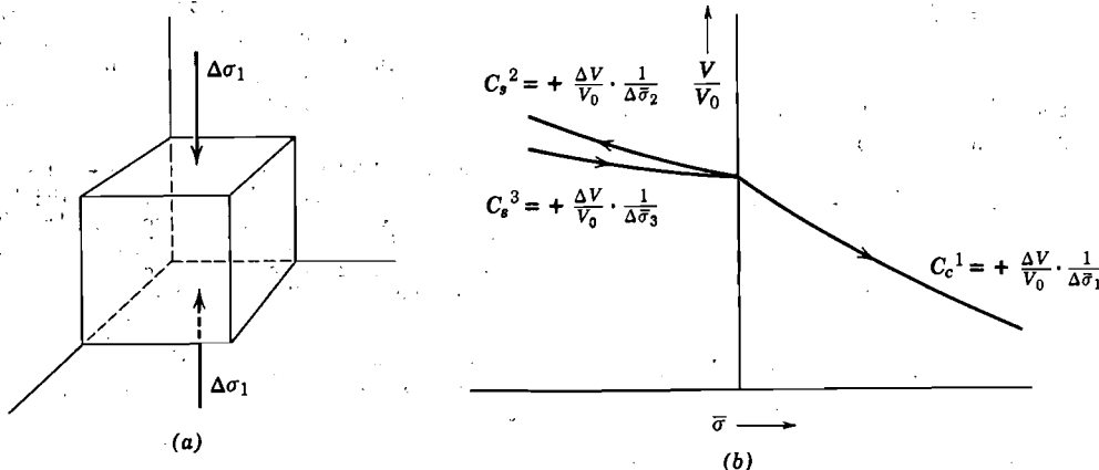
Fig. 26.7. Carga axial. a) Cargas. b) Deformaciones.
