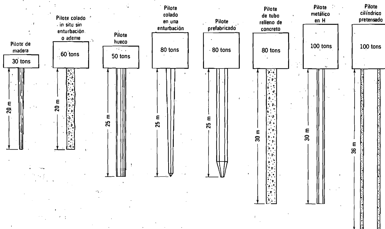
Fig. 33.2. Longitud y cargas máximas habituales de distintos tipos de pilotes (valores de proyecto). También son usuales cargas y longitudes mayores. (Según Carson, 1965).
