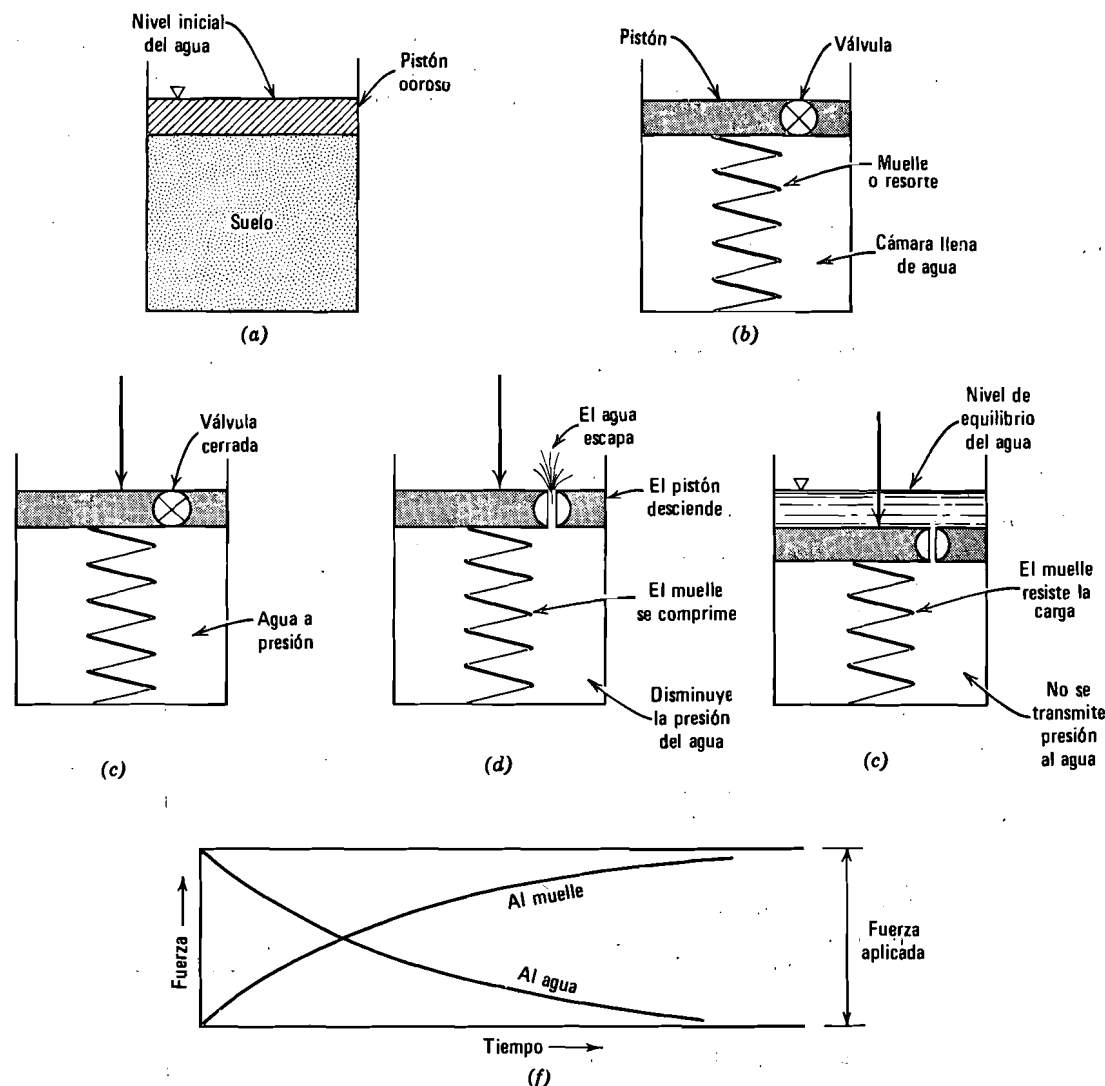
Fig. 2.5. Analogía hidromecánica para ilustrar la distribución de cargas en la consolidación. a) Ejemplo físico. b) Analogía hidromecánica; estado inicial. c) Carga aplicada con la válvula cerrada. d) El pistón descende al ir escapando el agua. e) Equilibrio sin más escape de agua. f) Transferencia gradual de carga.
