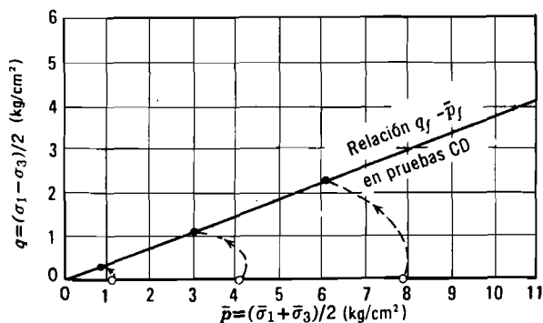
Fig. 28.7. Trayectorias de esfuerzos efectivos en pruebas CSD con arcilla wealdense consolidada.
