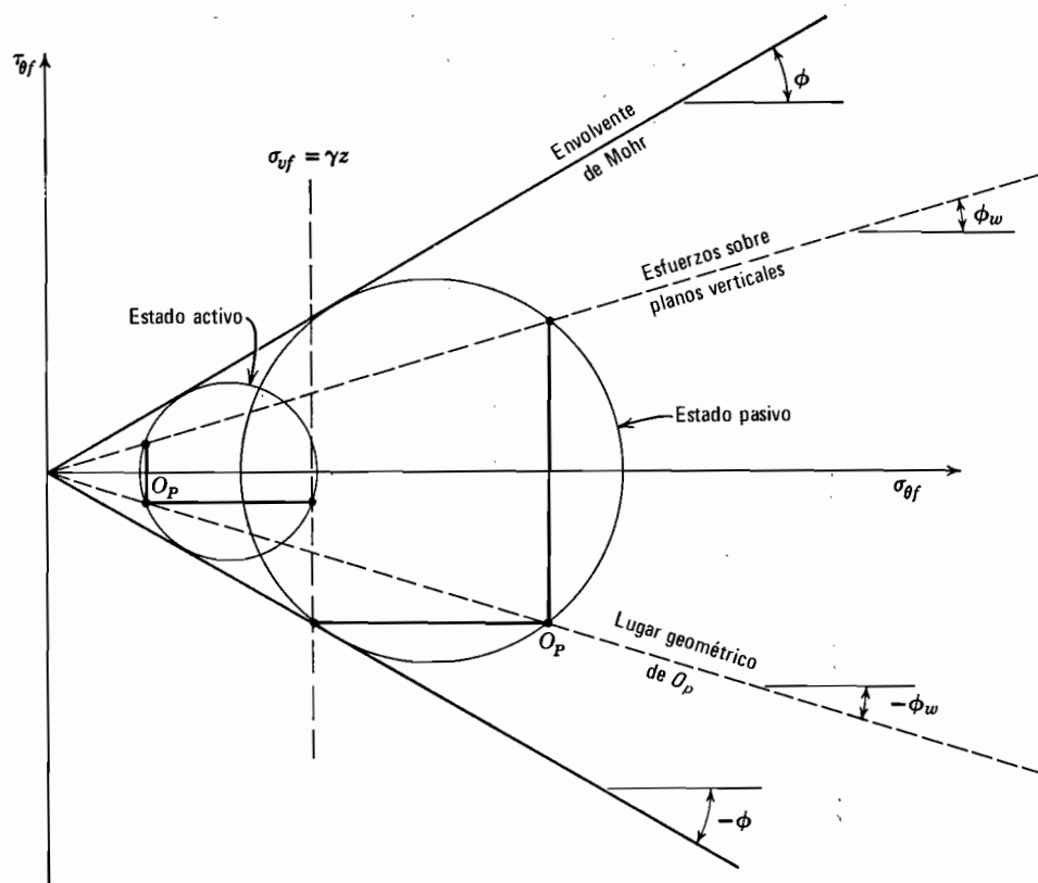
Fig. 13.8. Estados de Rankine en un terreno horizontal con esfuerzos tangenciales sobre superficies verticales.
