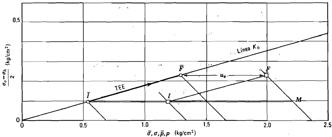
Fig. E25.6-3. Trayectorias de esfuerzos.
