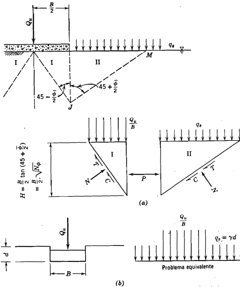
Fig. 25.7. Obtención de la fórmula de capacidad de carga a partir de las cuñas de Rankine. (a) Deducción. (b) Problema equivalente.
