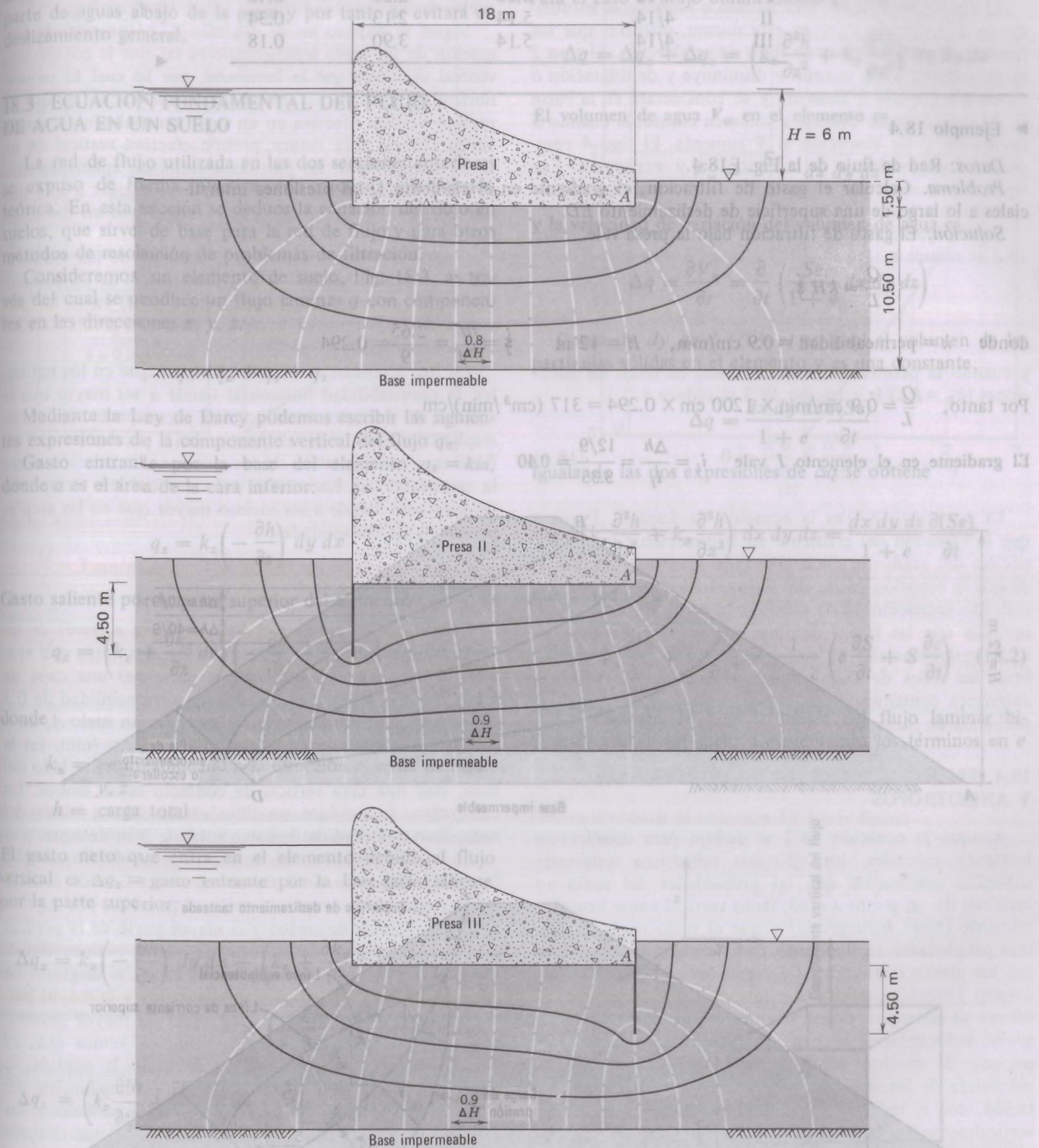
Fig. E18.3. Flujo bajo tres presas.
