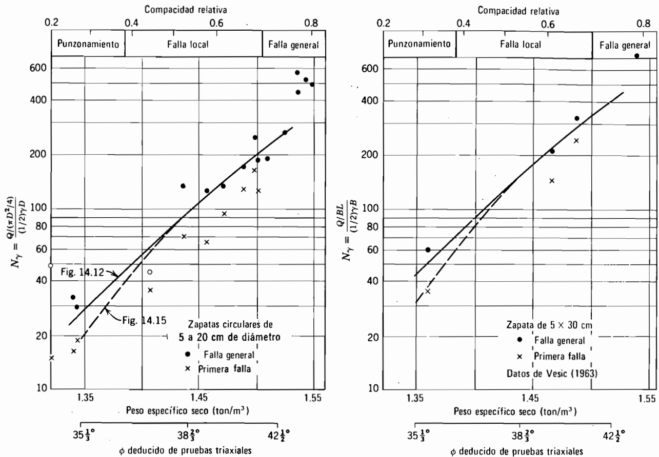
Fig. 14.17. Comparación entre los valores de N_\gamma calculados y medidos.
