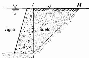
Fig. 23.7. Muro de retención completamente sumergido.
