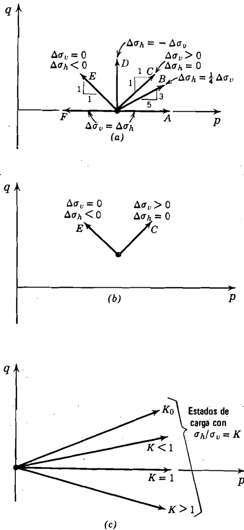
Fig. 8.11. Ejemplos de trayectorias de esfuerzos. a) Inicialmente \sigma_v = \sigma_h . b) Inicialmente \sigma_v > \sigma_h > 0 . c) Inicialmente \sigma_v = \sigma_h = 0 .
