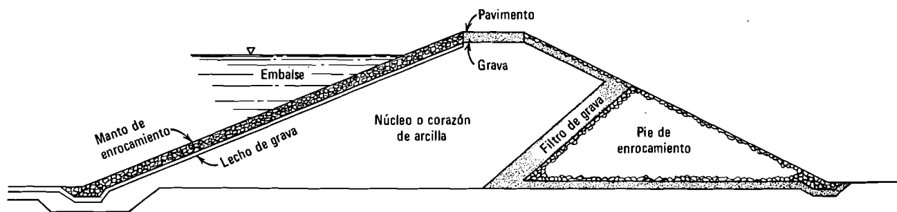
Fig. 1.8. Presa de tierra
