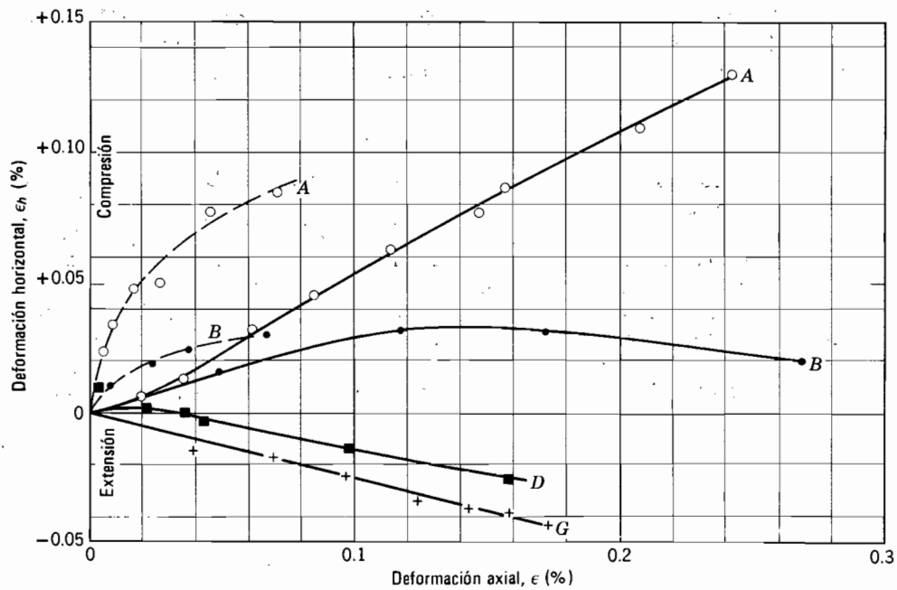
Fig. 10.23. Datos esfuerzo-deformación para cargas sin llegar a la falla.
