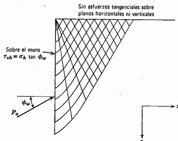
Fig. 13.16. Campo de líneas de deslizamiento y zona en estado de falla para el caso de un muro con fricción. (Deducido por el método de Sokolovski (1965) para \phi = \phi_w = 30^\circ ).
