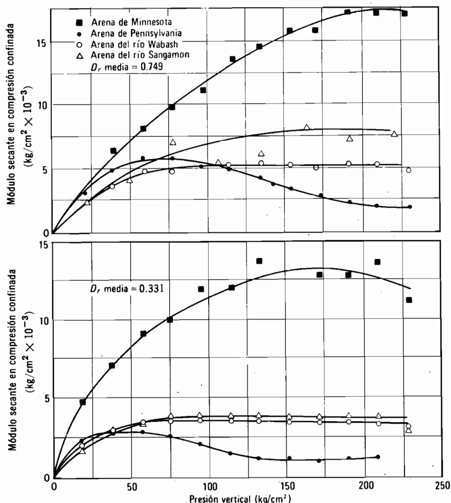
Fig. 12.3. Comportamiento de varias arenas en compresión unidimensional. Módulo secante desde 0 hasta la presión indicada. (Según Hendron, 1963).
