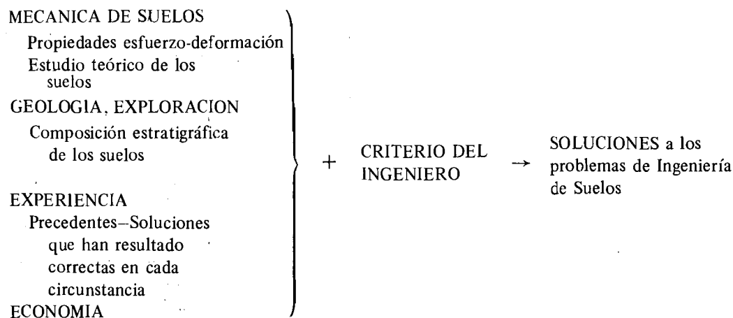
Fig. 1.19. Proceso de resolución de los problemas de Mecánica de Suelos planteados en Ingeniería Civil.
