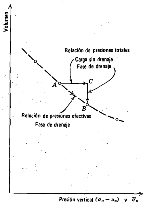
Fig. 28.2. Relación presión-deformación en la prueba edométrica.
