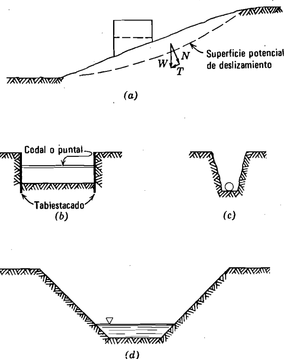
Fig. 1.12. Taludes y excavaciones. a) Talud natural. b) Excavación para un edificio. c) Zanja para una conducción. d) Canal.
