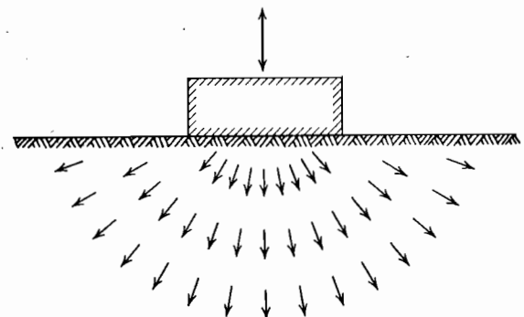
Fig. 15.4. Ondas emitidas por una cimentación en vibración.
