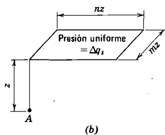
Fig. 8.6. a) Abaco para la determinación de esfuerzos verticales bajo las esquinas de una superficie rectangular con carga uniforme en un material elástico e isotrópico. Del ábaco se obtiene f(m,n) . b) Para el punto A, \Delta\sigma_v = \Delta q_s \times f(m,n) . (Según Newmark, 1942).
