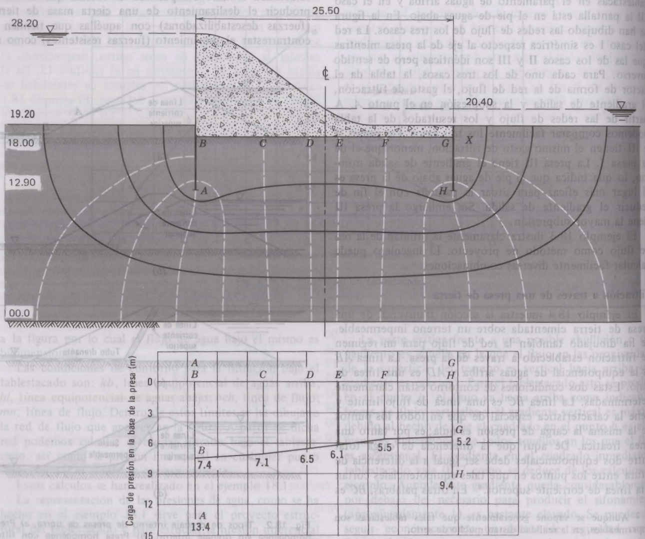
Fig. E18.2. Filtración bajo una presa.
