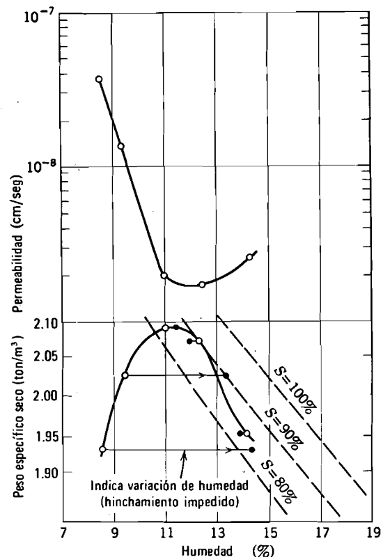
Fig. 34.8. Pruebas de compactación-permeabilidad en arcilla de Siburua. (Según Lambe, 1962).
