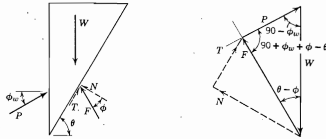
Fig. 13.17. Equilibrio de la cuña deslizante tanteada en el caso de un muro de retención con fricción.
