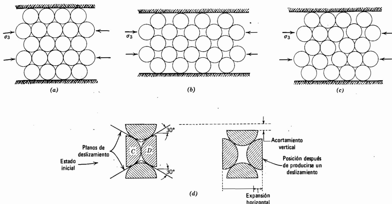
Fig. 10.16. Deformaciones en una agrupación regular de esferas. a) Agrupación inicialmente compacta. b) Estado más suelto posible-deformaciones uniformes. c) Estado suelto-deformaciones no uniformes. d) Comportamiento de unidad elemental.
