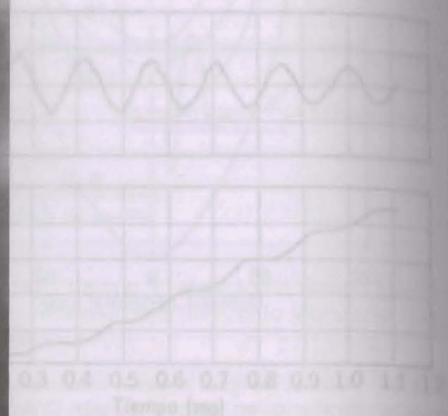
Fig. 15.18. Aceleración y desplazamiento del talud de arena de Monterrey No. 20. Talud de 31°. (Skempton, 1965).
