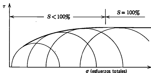
Fig. 28.17. Pruebas sin consolidación ni drenaje de suelos parcialmente saturados.
