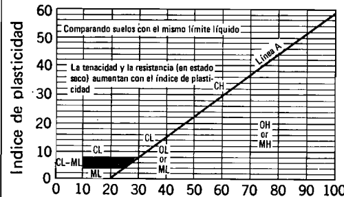
Límite líquido Gráfico de plasticidad para la clasificación en laboratorio de suelos de grano fino
