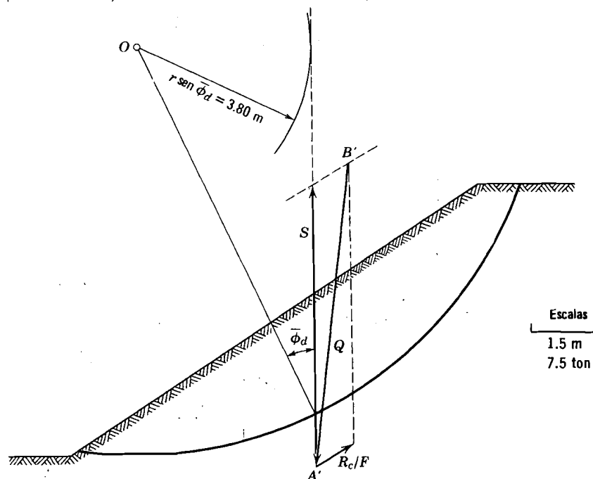
Fig. E24.3-4. Equilibrio de fuerzas.
