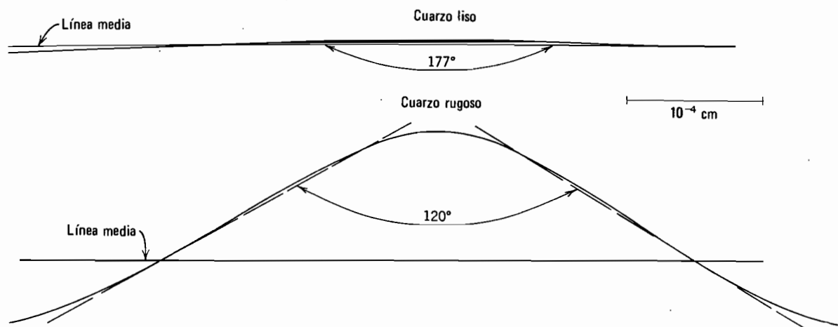
Fig. 6.4. Asperidades típicas de la superficie del cuarzo.
