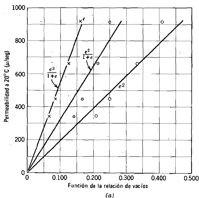
Fig. 19.9. Resultados de pruebas de permeabilidad con carga variable.
