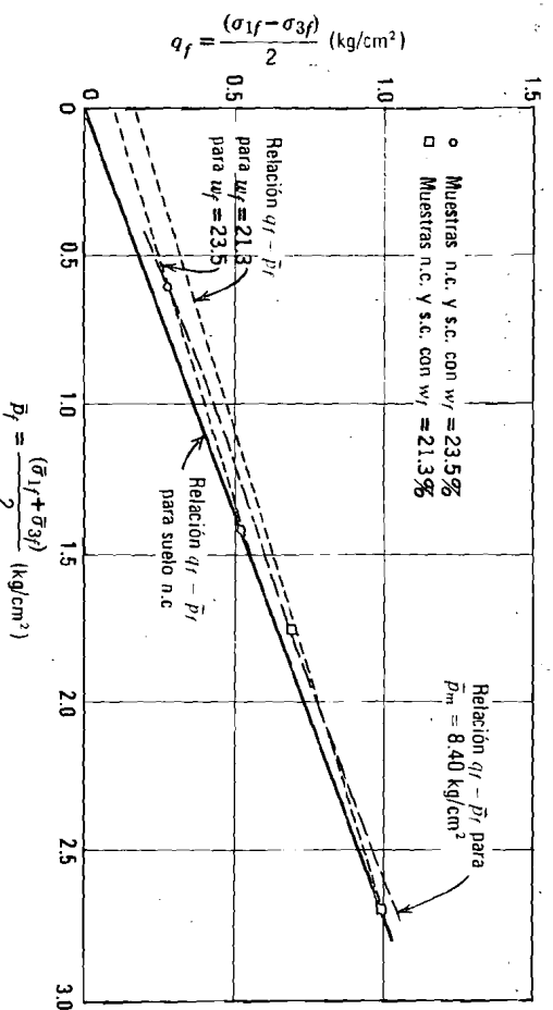
Fig. 21.11. Construcción gráfica para obtener los parámetros de Hvorslev.
