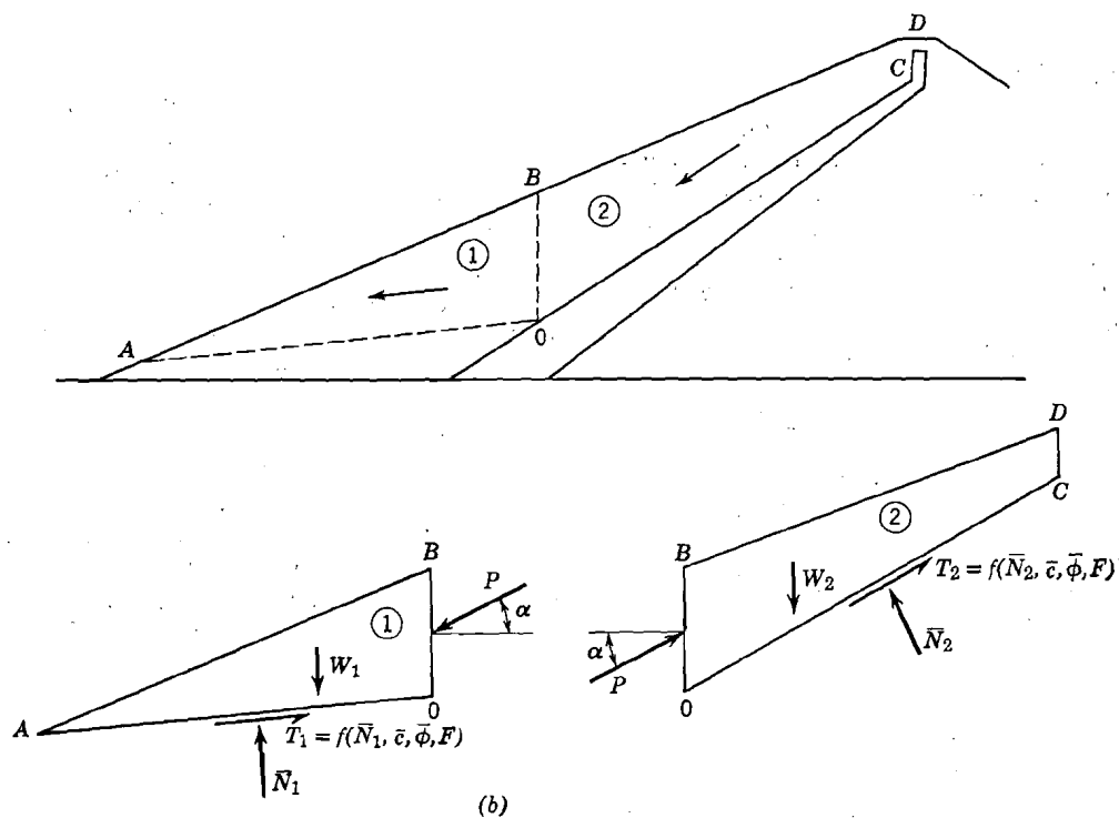
Fig. 24.15. Cálculo de la estabilidad por el método de las cuñas deslizantes. a) Falla de cuña en un modelo de presa con núcleo inclinado (Sultán y Seed, 1967). b) Cuñas y fuerzas.
