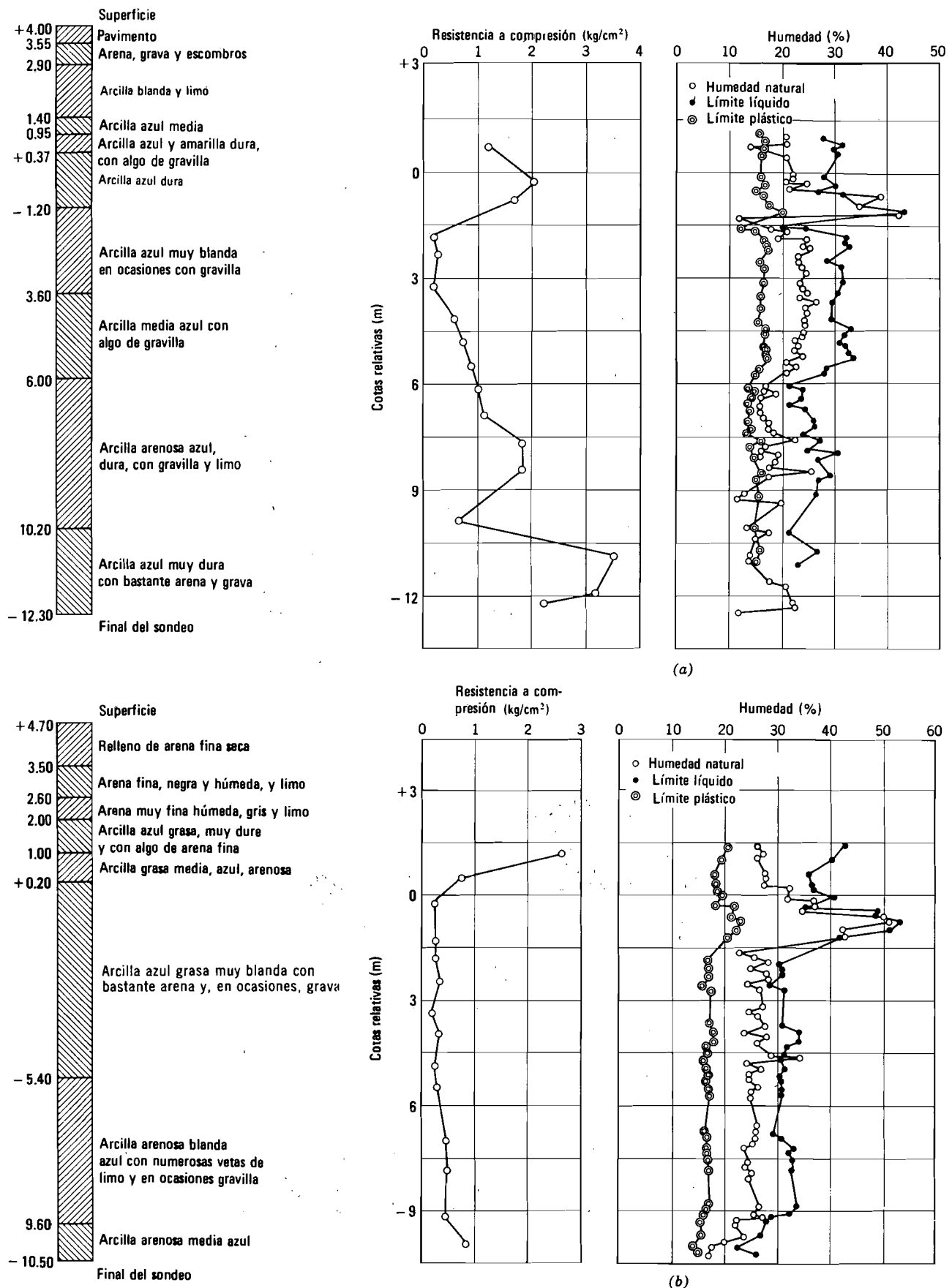
Fig. 7.14. Suelos de Chicago. a) Sondeo en la calle División cerca de la Avenida de Milwaukee (1200N, 1600W). b) Sondeo en la calle del Congreso y en la Avenida de Racine (500S, 1200W). (Según Peck y Reed, 1954).
