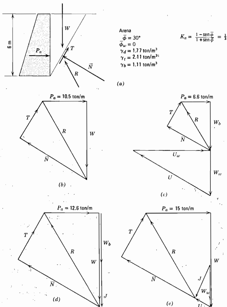
Fig. 23.10. Polígonos de fuerzas para varios casos. b) Terreno seco. c) Terreno sumergido. d) Filtración vertical. e) Drenaje vertical.
