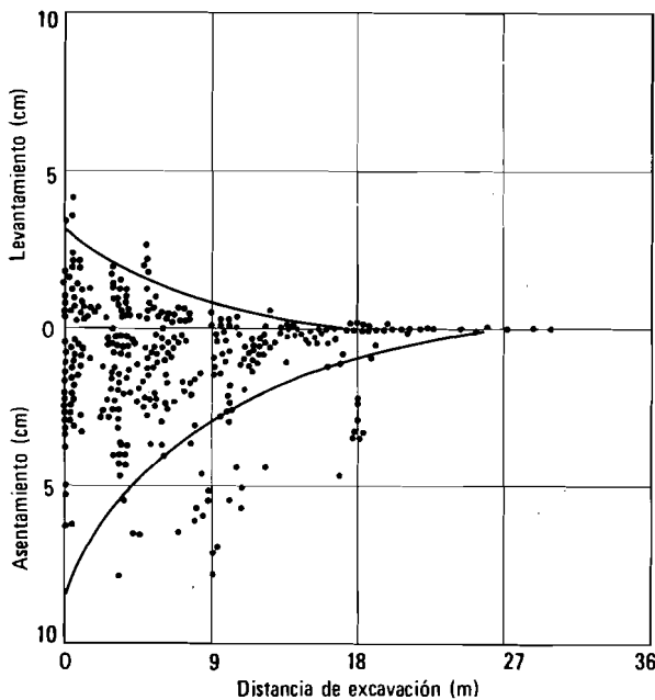
Fig. 33.9. Movimientos en edificios debido a la hincada de pilotes, Chicago, Ill. (Según Horn, 1966.) Citado por Ireland (1955).
