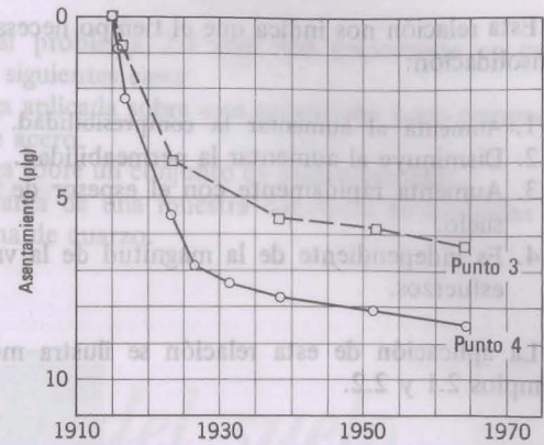
Fig. 2.6. Asentamiento del edificio N.º 10 del I. T. M.
