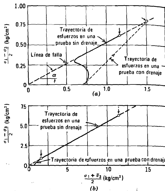
Fig. 29.2. Trayectorias de esfuerzos en la prueba triaxial sin drenaje de una arena saturada. (a) Suelta e_0 = 0.85 . (b) Algo compacta, e_0 = 0.75 .
