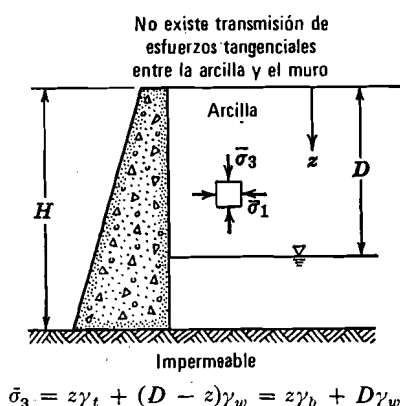
Fig. 23.12. Empuje pasivo en el caso de saturación capilar del relleno.
