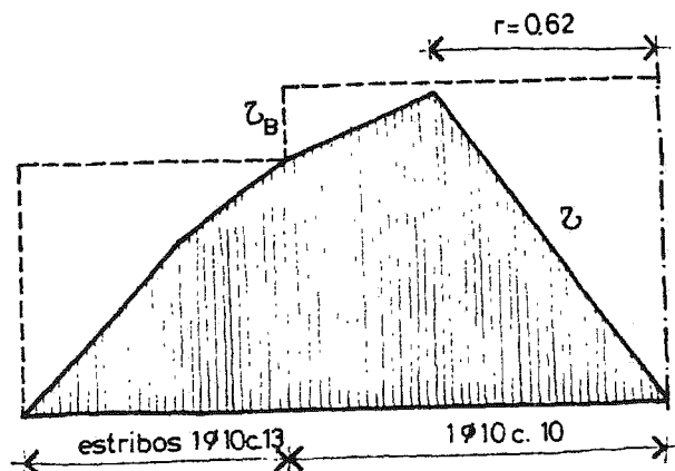
Planilla de esfuerzos de corte, momentos y esfuerzos de tracción
