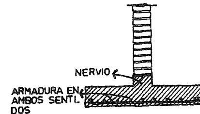
cimiento para suelos limo arenosos (zapatas corridas)
