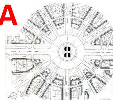
Fig. 22. Planta de la plaza de l'Étoile en París.
