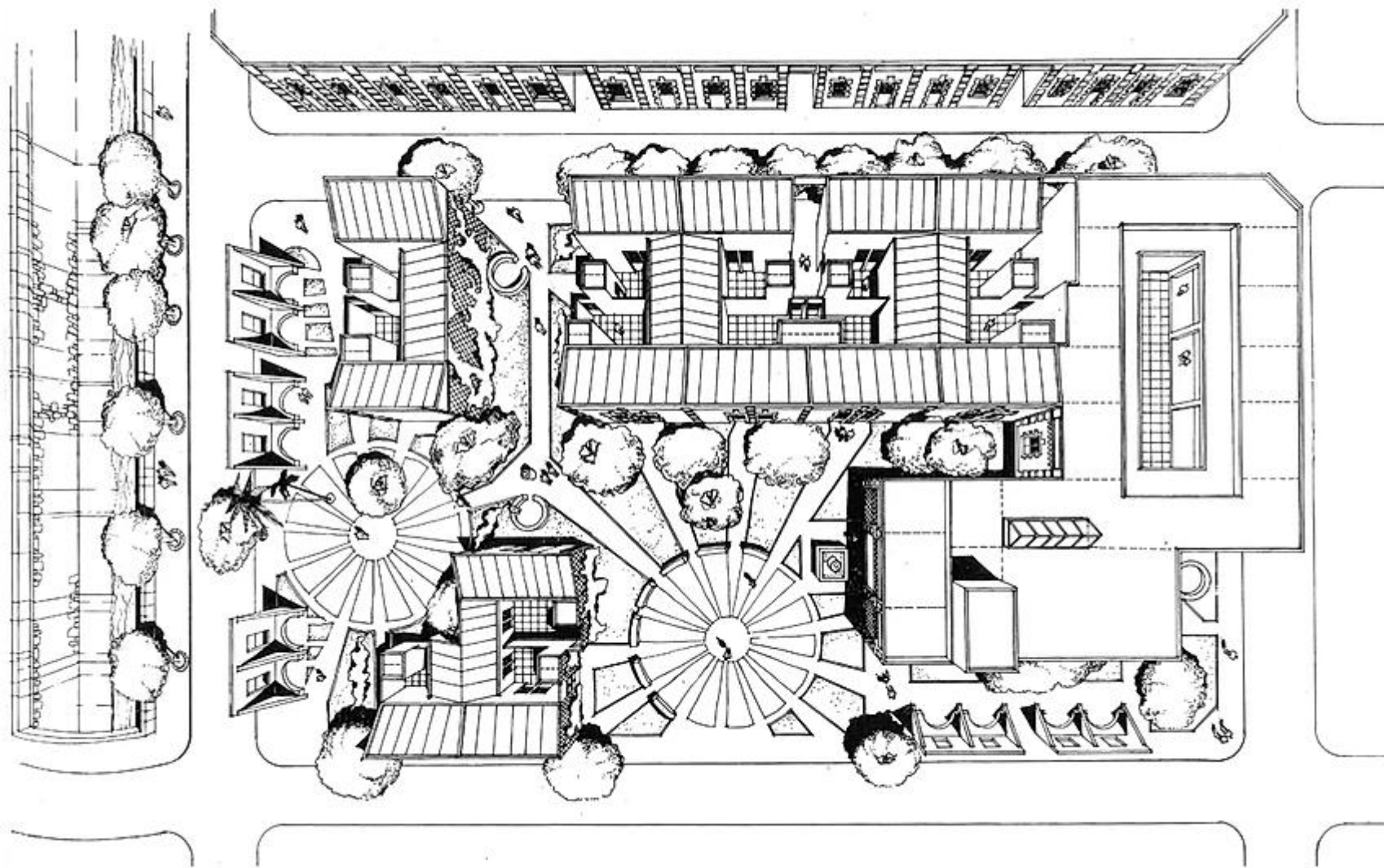
Planimetría fugada – Paseo de las Artes – Arquitecto Miguel Ángel Roca
